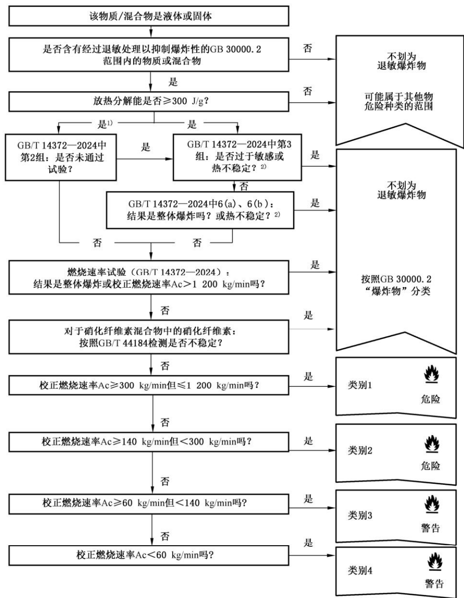
图 A.1 退敏爆炸物的判定逻辑图
