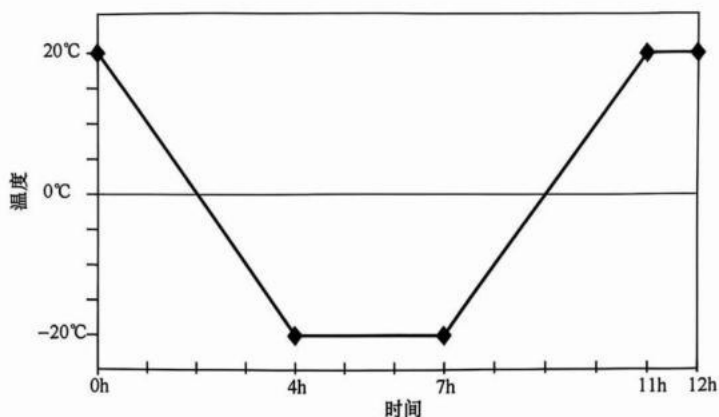
图 4.3.3-4 冻融循环制度
