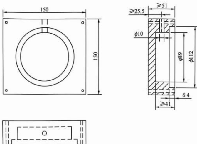
图 7.2.2-2 试验槽示意图
