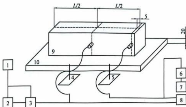
图 5.0.4 各部件连接和相对位置示意图
