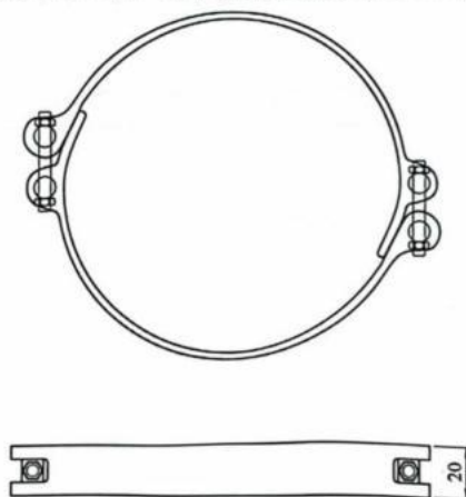
图 7.1.5 不锈钢环箍
