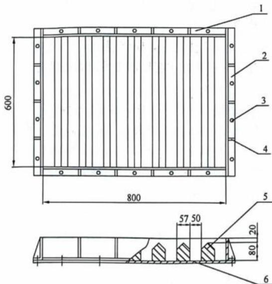
图 9.0.2 混凝土早期抗裂试验装置示意图
