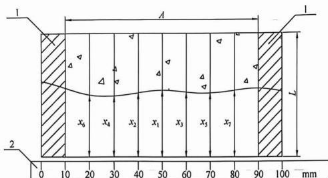
图 7.1.7 显色分界线位置编号
