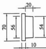
图 8.3.2-2 波纹管 密封端塞
