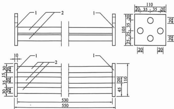
图 8.3.2-3 波纹管法测试支架
