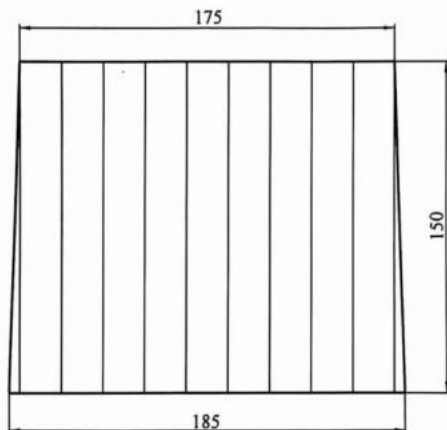
图 6.1.2 梯形板示意图
