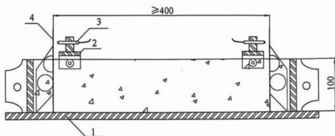
图 8.1.3 非接触法混凝土收缩变形测定仪原理示意图
