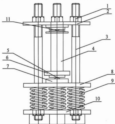
图 10.0.2 弹簧式压缩徐变仪
