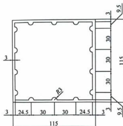
图 4.2.2 橡胶试件盒横截面示意图
