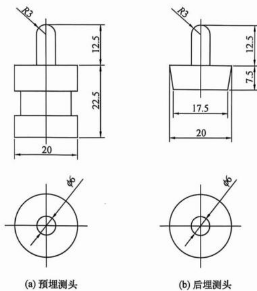
图 8.2.2-1 卧式收缩试验用测头
