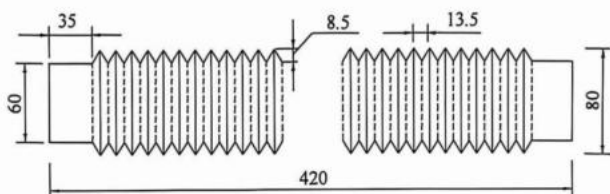
图 8.3.2-1 波纹管
