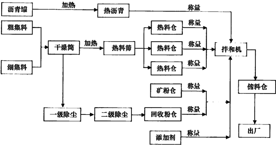
图 B.1 沥青混合料拌和工艺流程图
