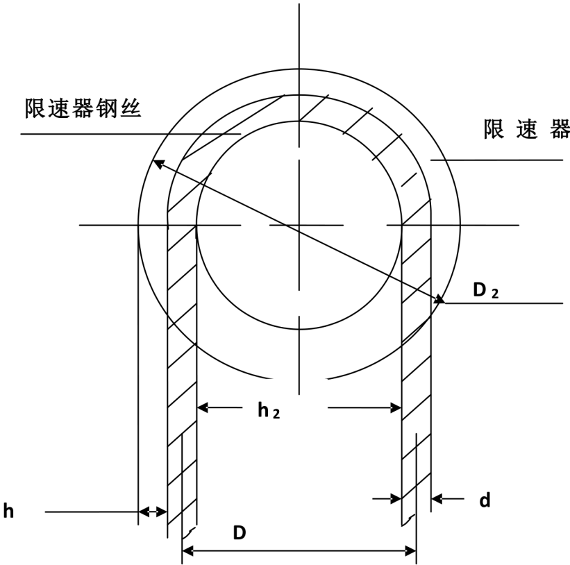
图B. 1 电梯限速器节圆直径图
