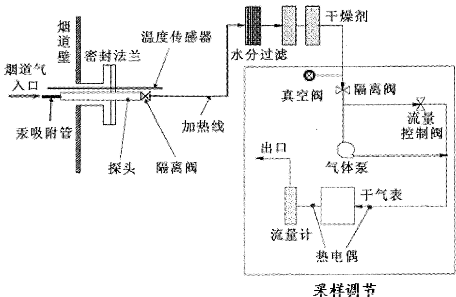
图1 气态汞采样系统图
