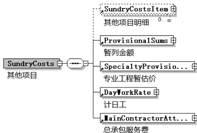
图 C.2.22 其他项目元素
