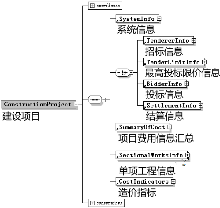
图 C.1.1 建设项目元素
