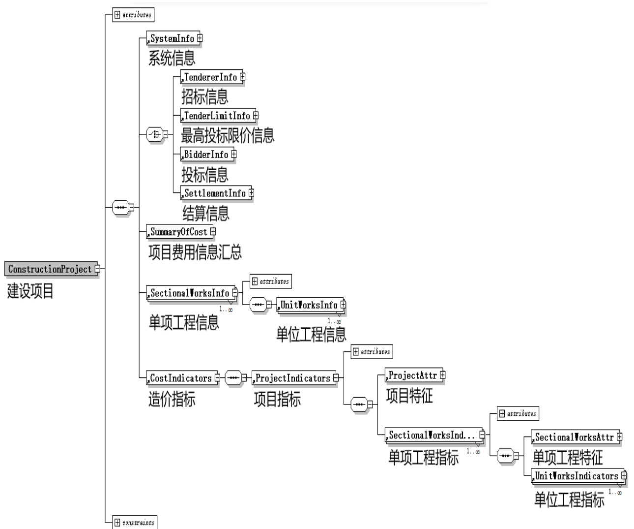
图 C.3.1 建设项目文件的组成元素及关系图
