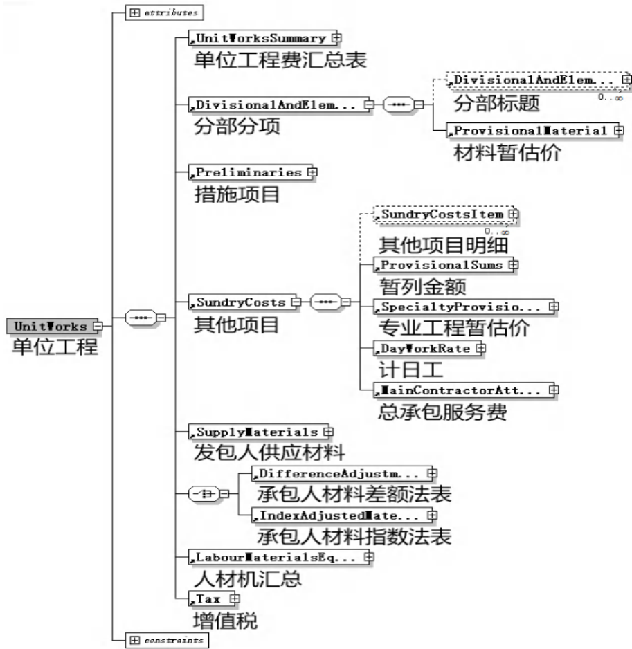
图 C.3.2 单位工程文件组成元素及关系图
