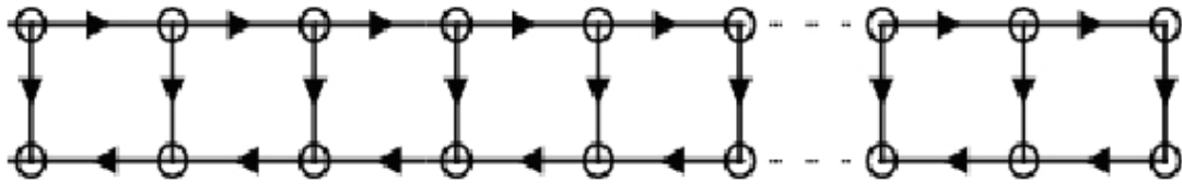
图 3 矩形环单程水准测量闭合环示意图
