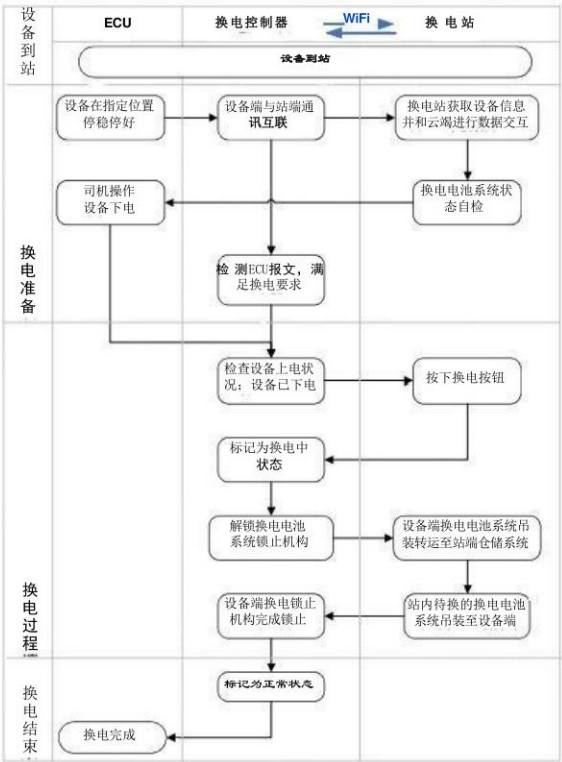
图4 换电场站作业流程图
