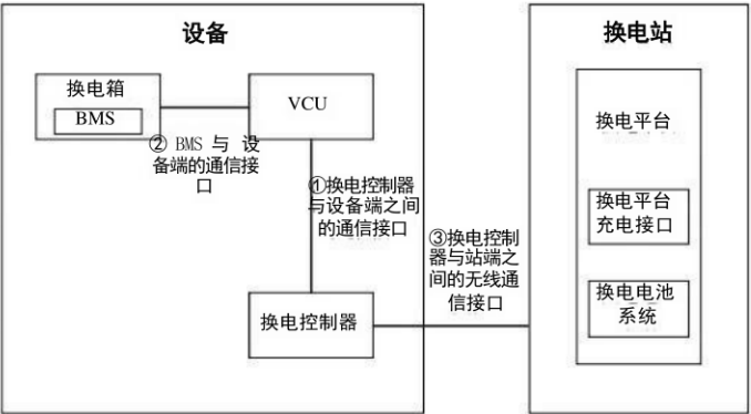
图3 换电控制器与设备端、换电场站之间流程关系图
