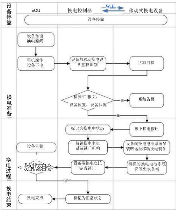
图5 移动式换电装备作业流程图
