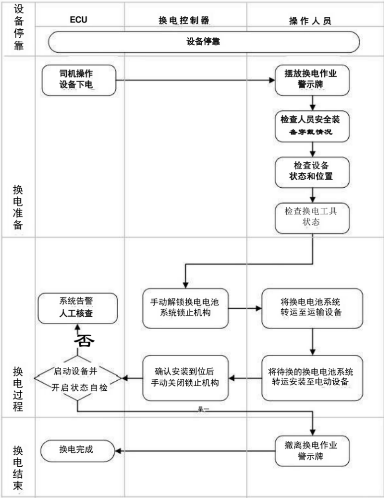
图6 手动应急换电作业流程图
