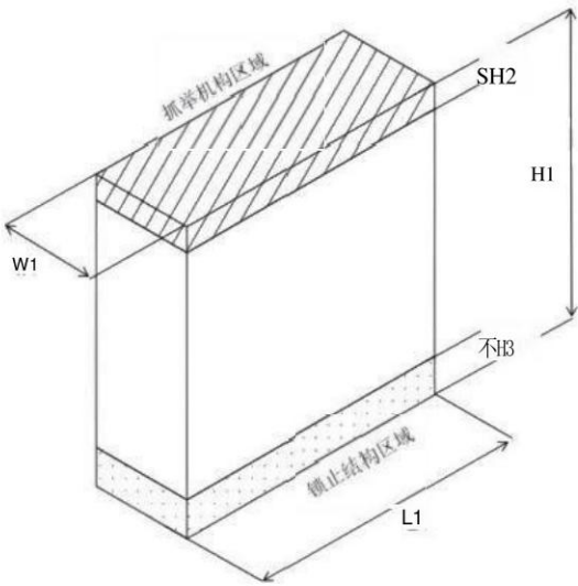
图2 吊装式换电电池系统外廓尺寸示意图
