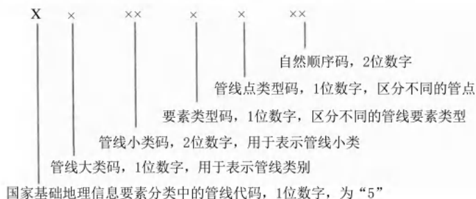
图7.2.5 管线要素编码结构
