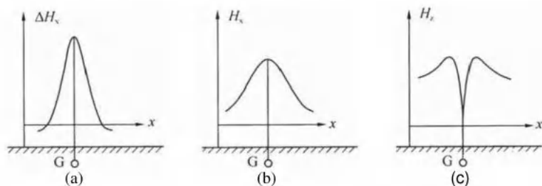
图 1 电磁感应法管线定位示意
