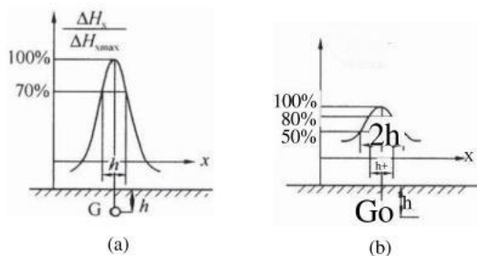
图 2 电磁感应法管线定深示意
