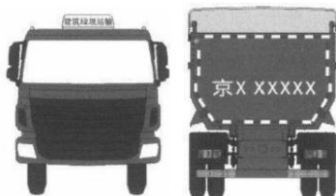
图2 车辆后箱板标示样式及尺寸
