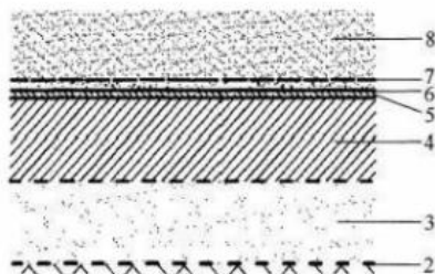
图10.5.4 库区底部单层衬里结构示意图
