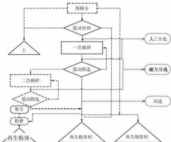
图B.0.1 移动式处理设施生产工艺流程示意
