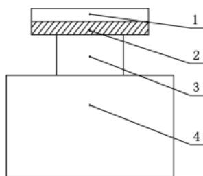
图 A.1 抗振动性能试验装置示意图
