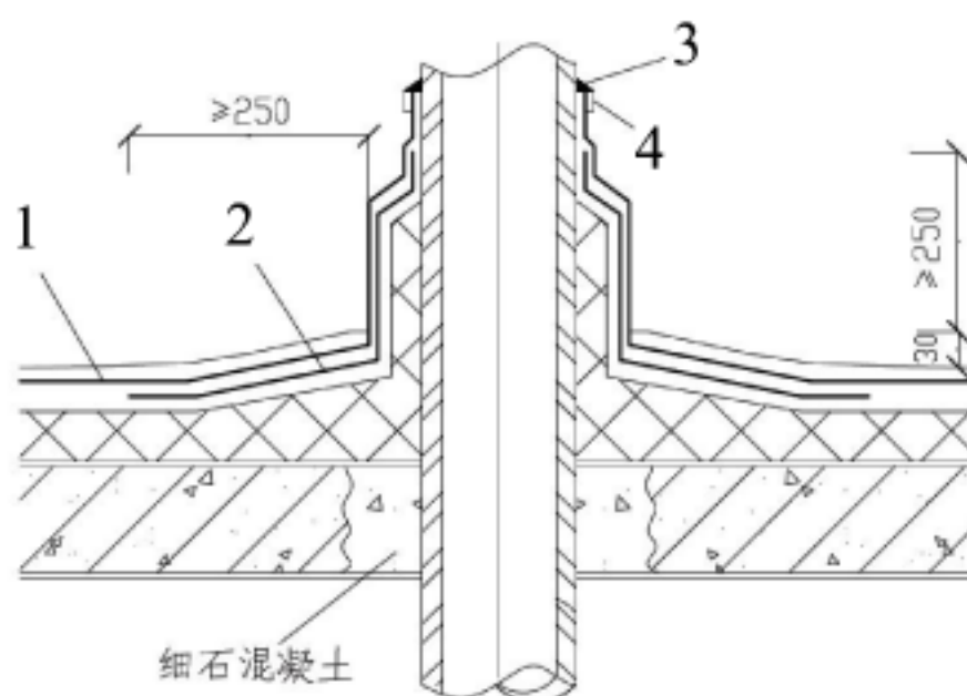
图 20 伸出屋面管道
