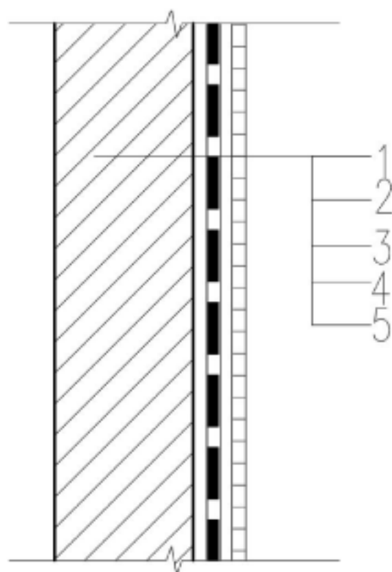
图 29 块材饰面外墙防水构造（无保温层）
