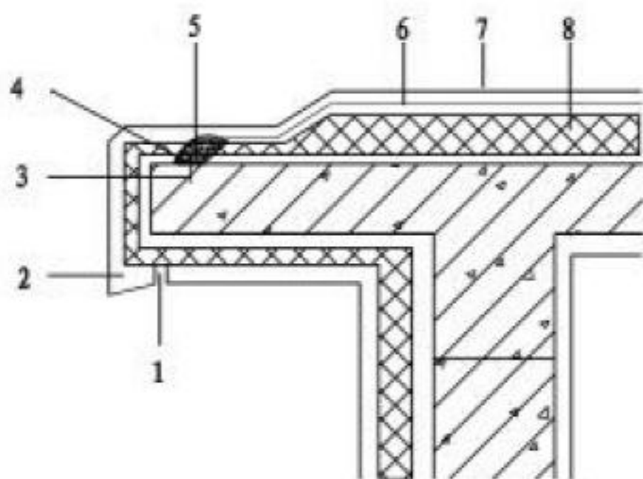
图 1 卷材防水屋面檐口
