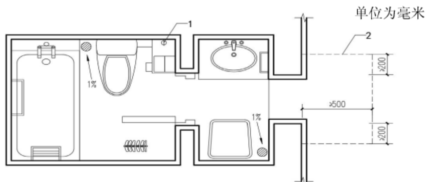
图 41 楼、地面门口处防水层延展示意
