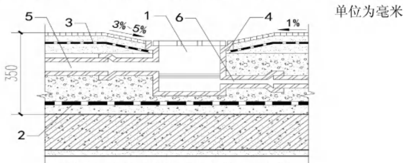
图 46 同层排水的地漏防水构造
