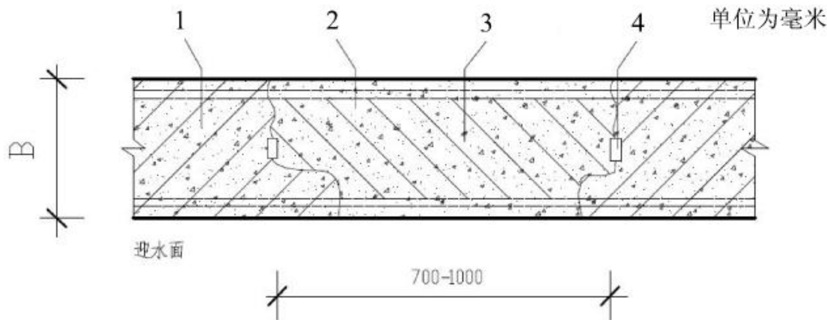
图 55 后浇带防水构造（三）
