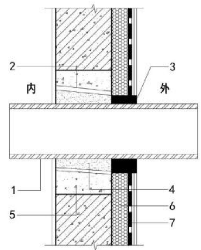
图 38 伸出外墙管道防水构造
