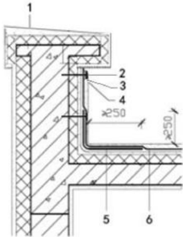
图 10 低女儿墙
