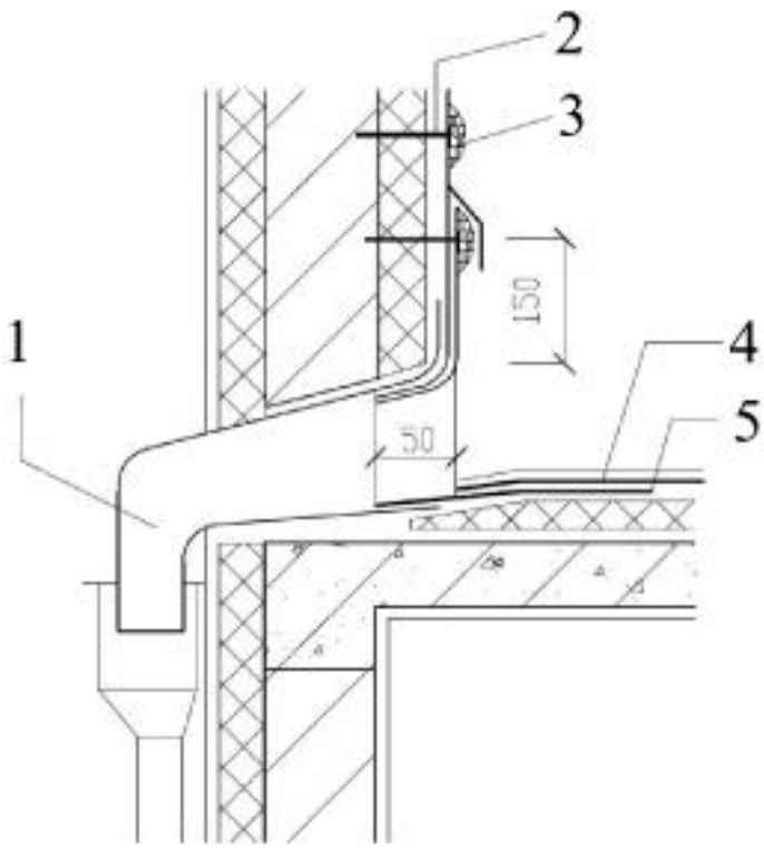
图 17 横式水落口
