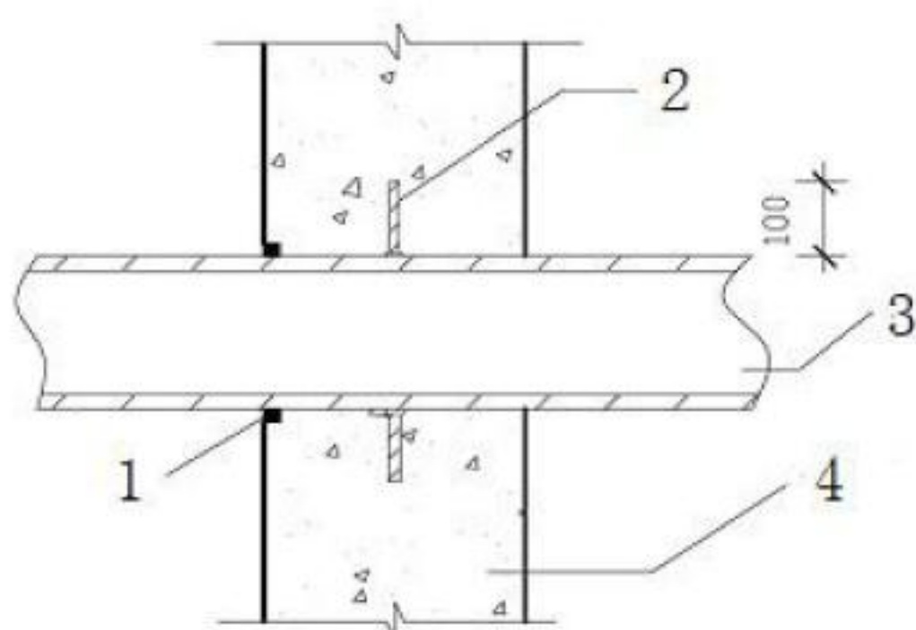
图 57 固定式穿墙管防水构造（一）
