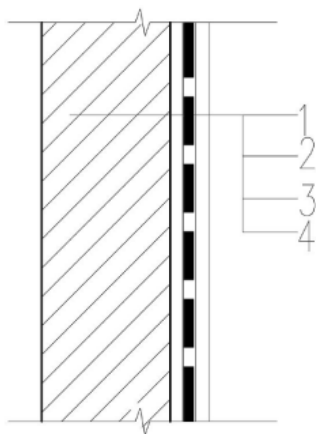
图 28 涂料饰面外墙防水构造图（无保温层）
