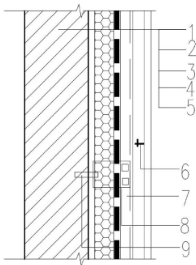
图 32 幕墙饰面外保温外墙整体防水构造
