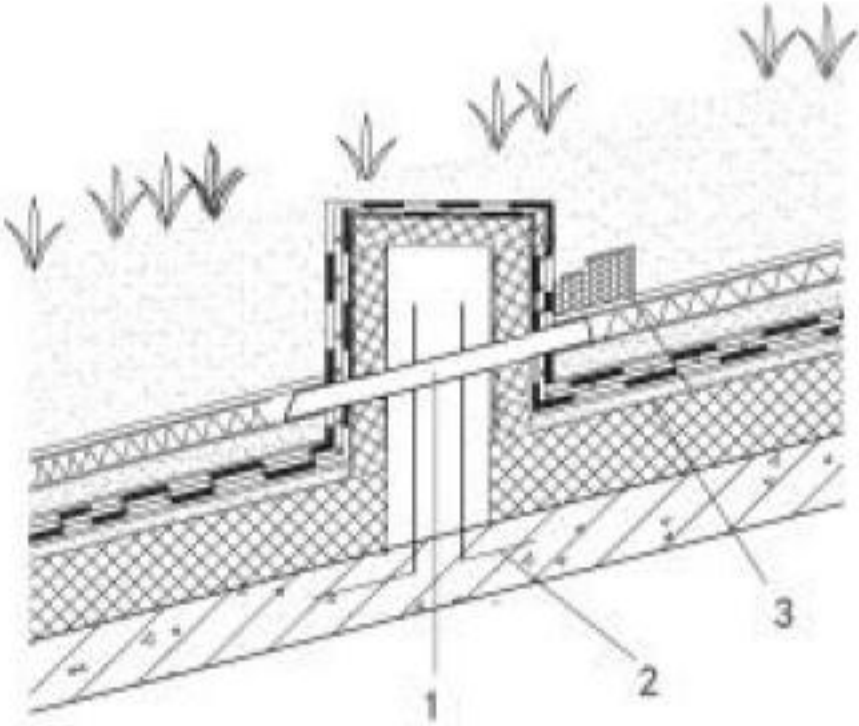
图 26 坡屋面防滑挡墙
