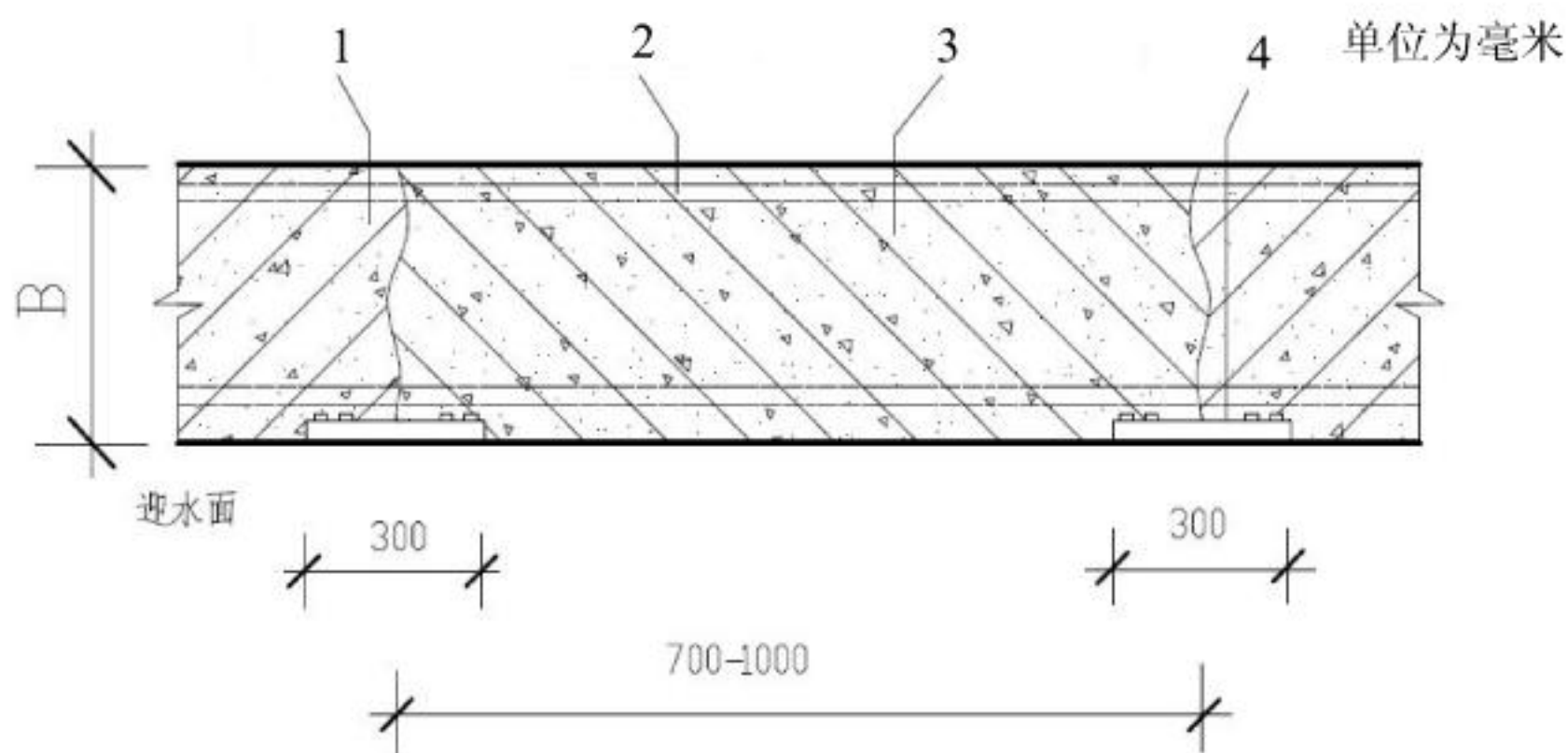
图 54 后浇带防水构造（二）
