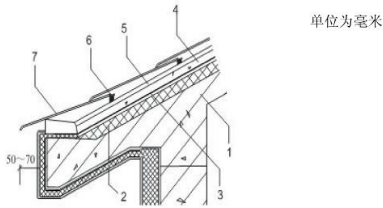
图 3 烧结瓦，混凝土瓦屋面檐口构造（一）
