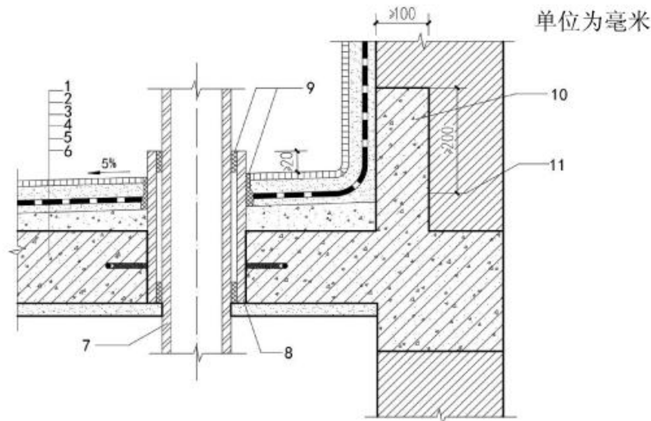
图 42 管道穿越楼板的防水构造（一）
