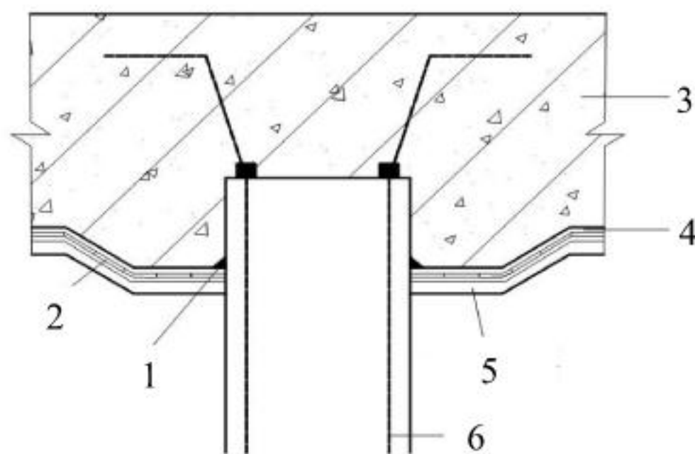
图 63 桩头防水构造（二）
