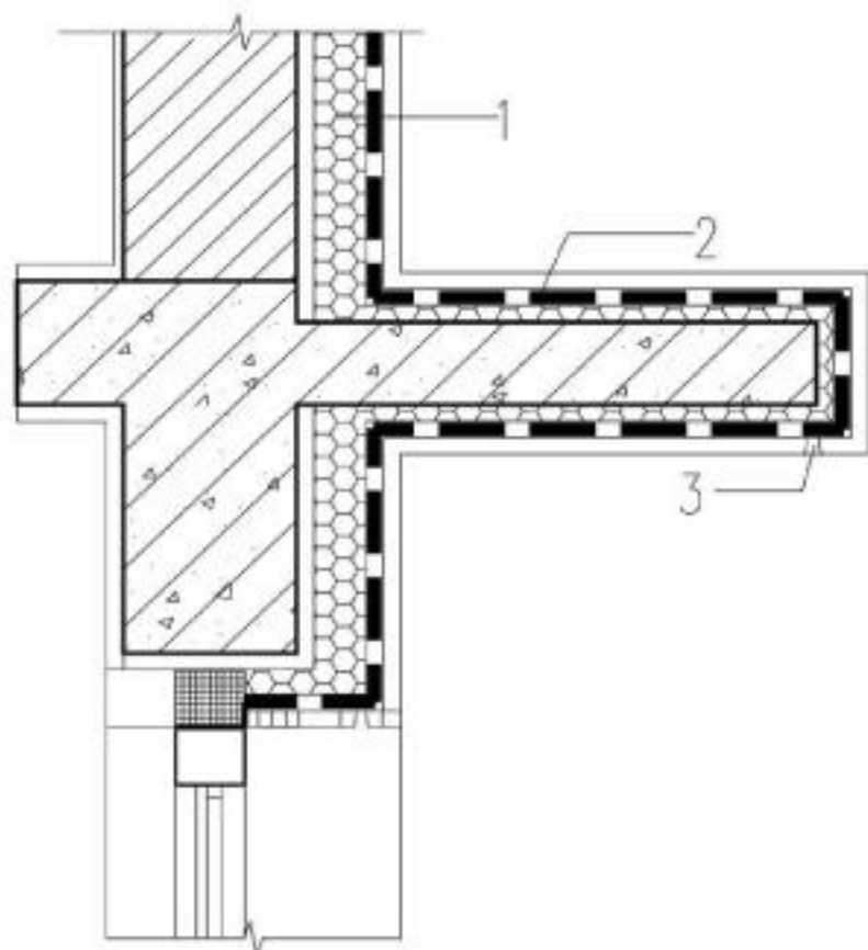
图 35 雨棚防水构造
