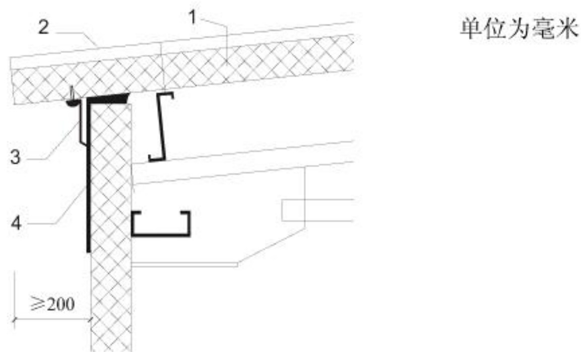
图 6 金属板屋面檐口构造
