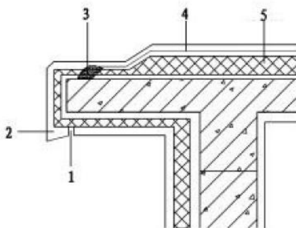
图 2 涂膜防水屋面檐口
