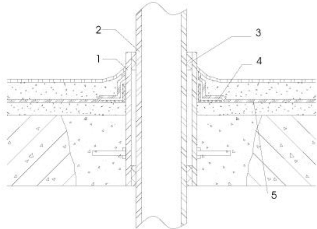
图 43 管道穿越楼板的防水构造（二）
