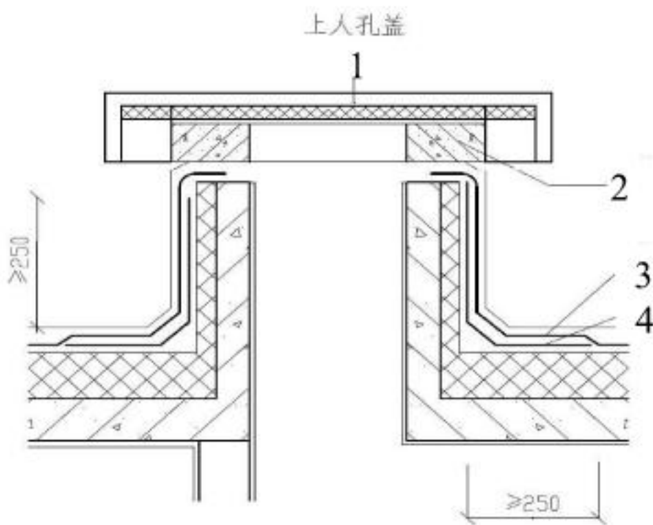
图 22 垂直出入口
