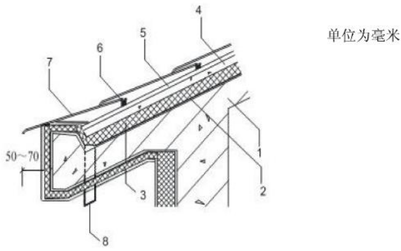
图 4 烧结瓦，混凝土瓦屋面檐口构造（二）
