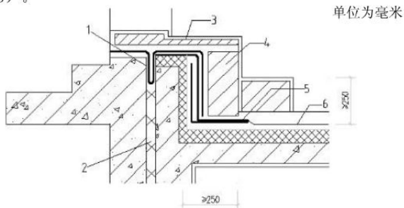
图 23 水平出入口
