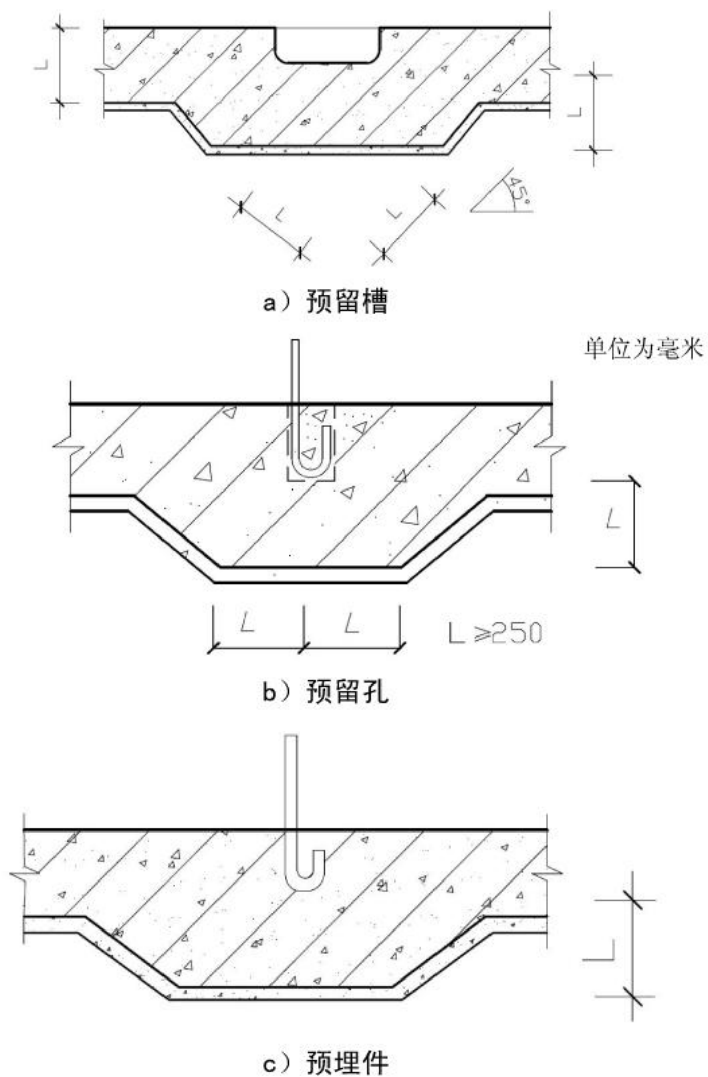
图 61 预埋件及预留孔(槽)处理
