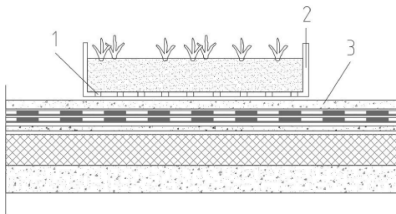
图 27 容器种植
