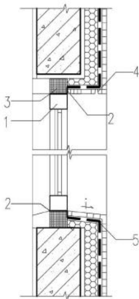
图 34 门窗框防水立剖面构造
