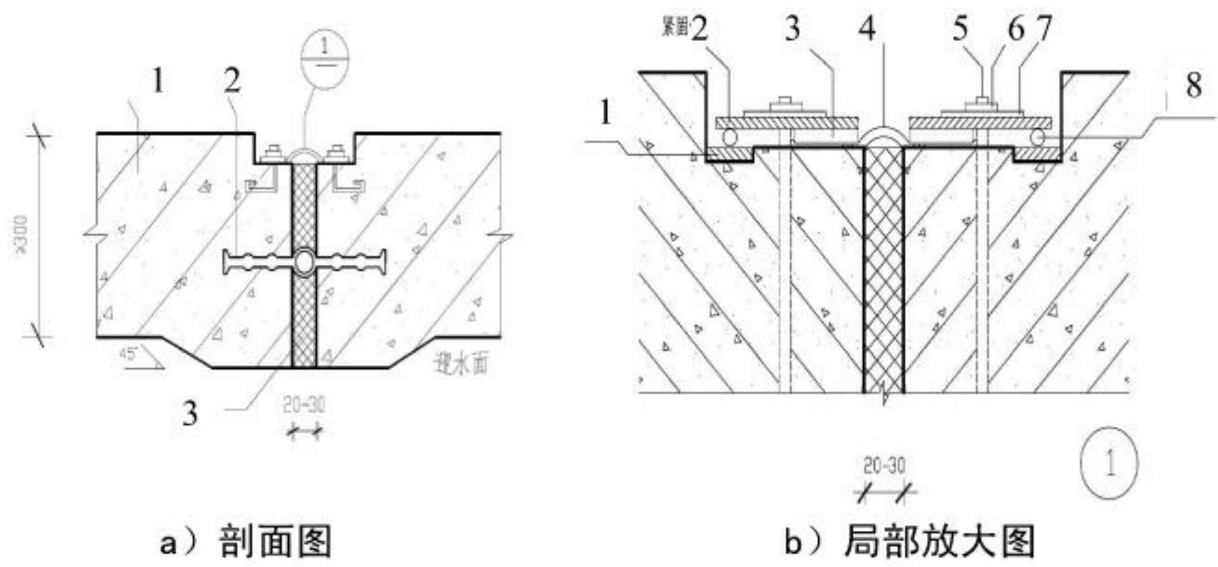
图 51 中埋式止水带与可卸式止水带复合使用
