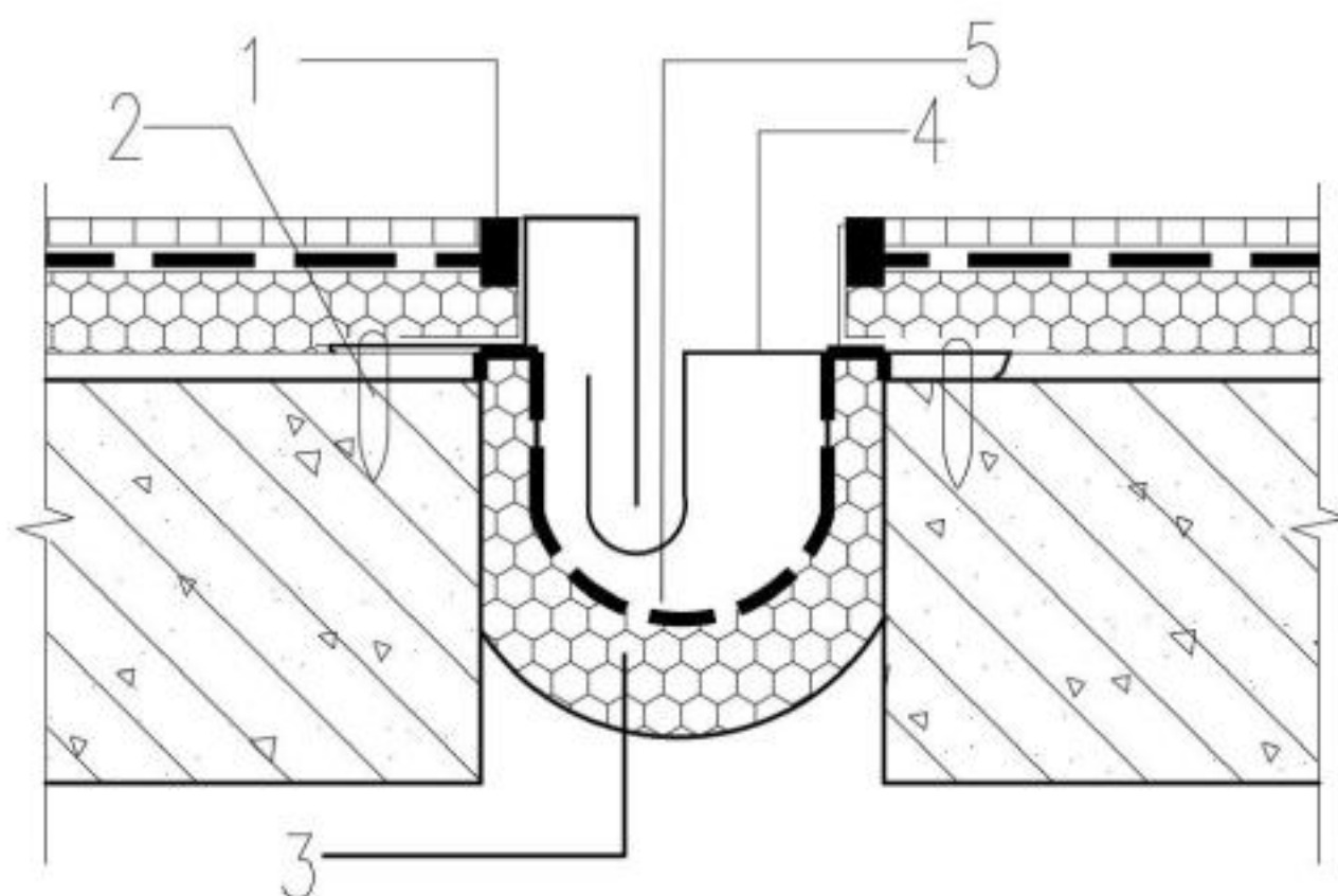
图 36 外墙沉降缝
