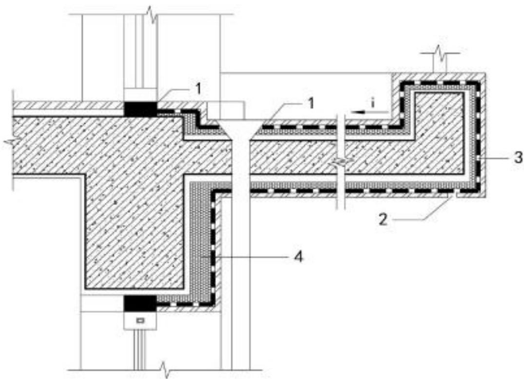
图 48 阳台防水构造
