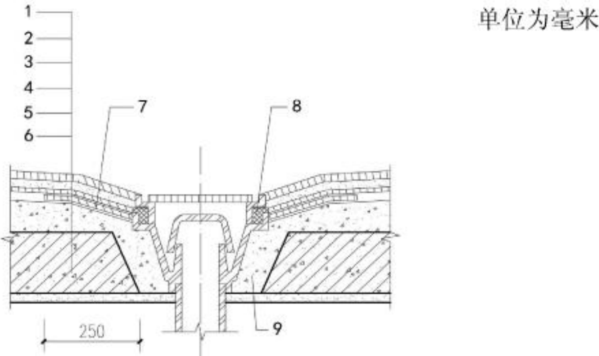
图 44 地漏防水构造
