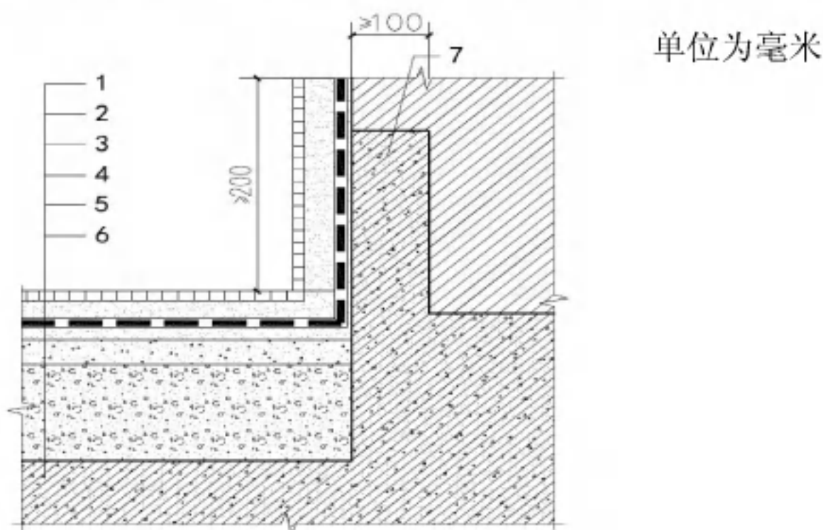
图 47 防潮墙面的底部构造
