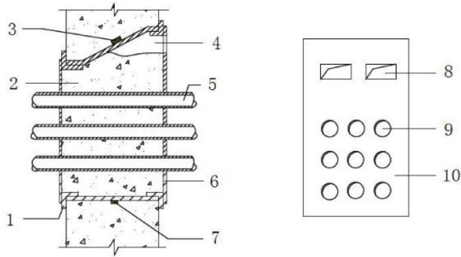
图 60 穿墙群管防水构造
