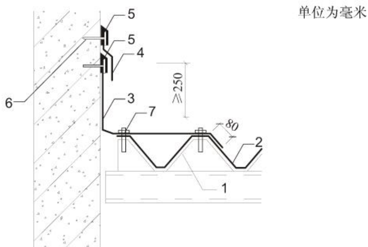
图 14 压型金属板屋面山墙防水构造
