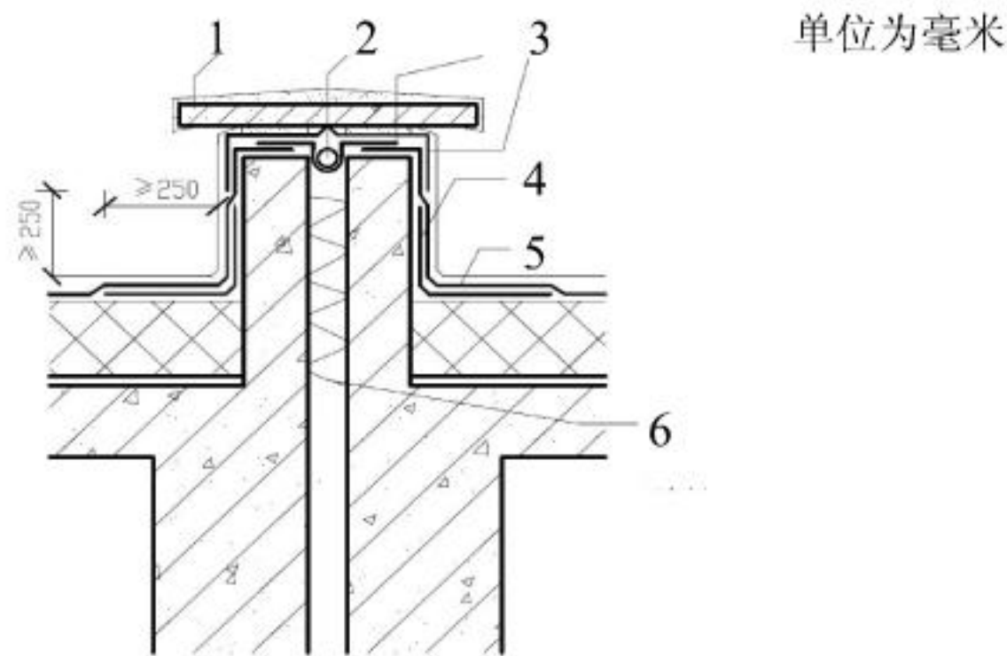
图 18 等高变形缝
