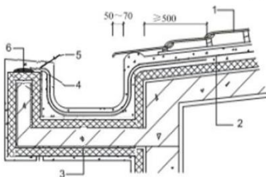
图 8 瓦屋面檐沟构造
