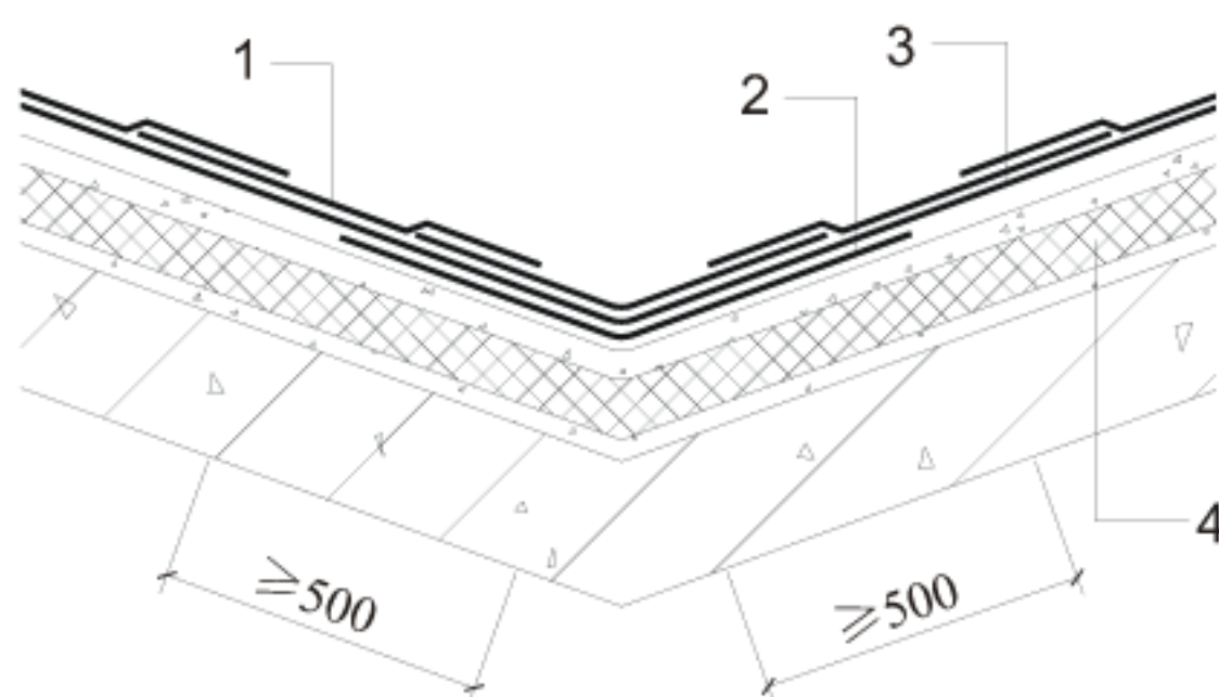
图 9 沥青瓦屋面檐沟和天沟
