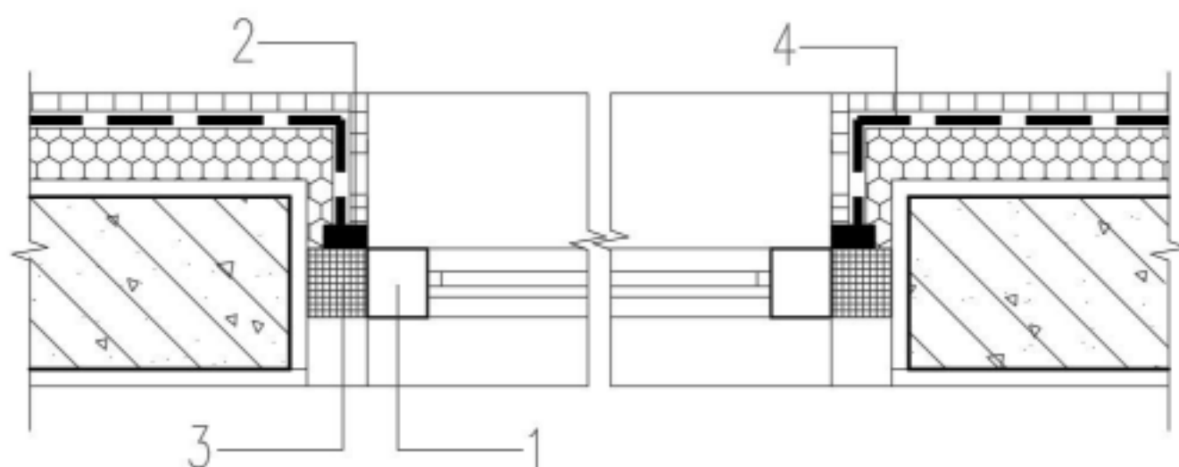
图 33 门窗框防水水平剖面构造
