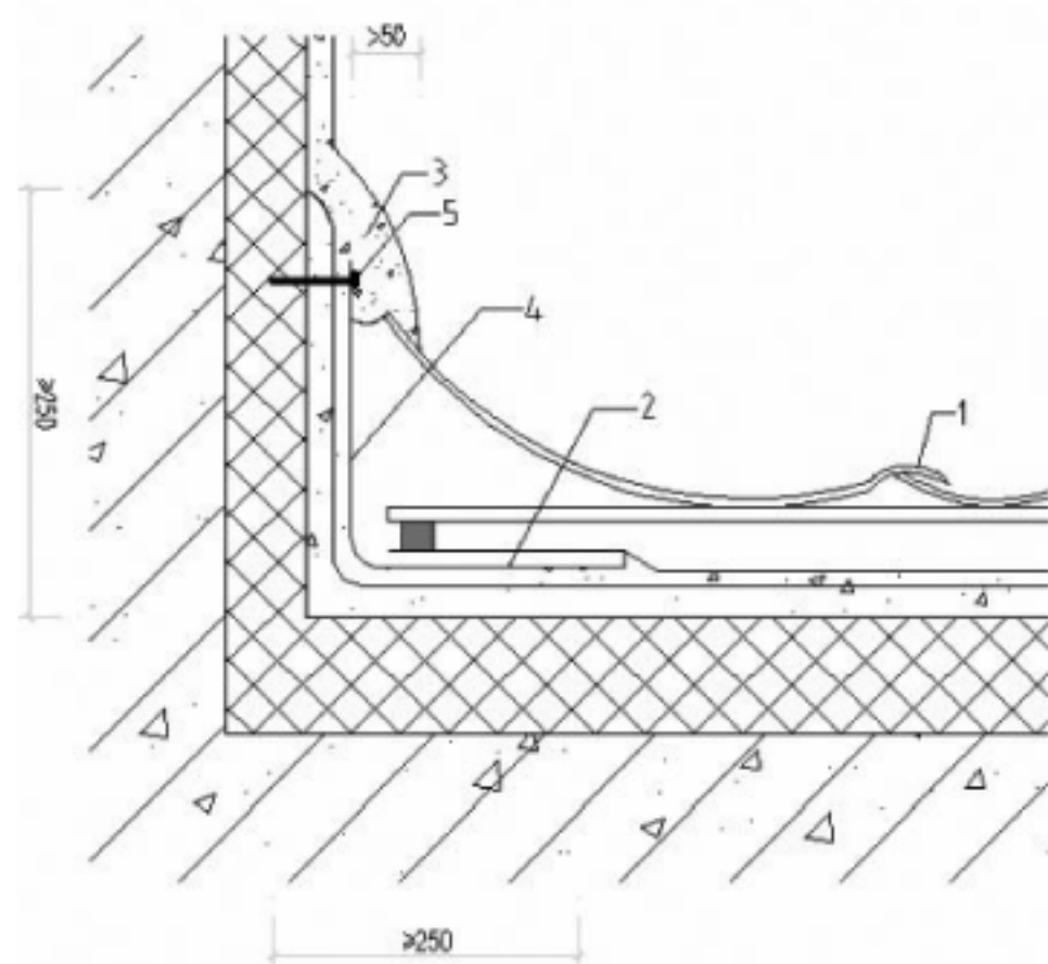
图 12 烧结瓦、混凝土瓦屋面山墙防水构造
