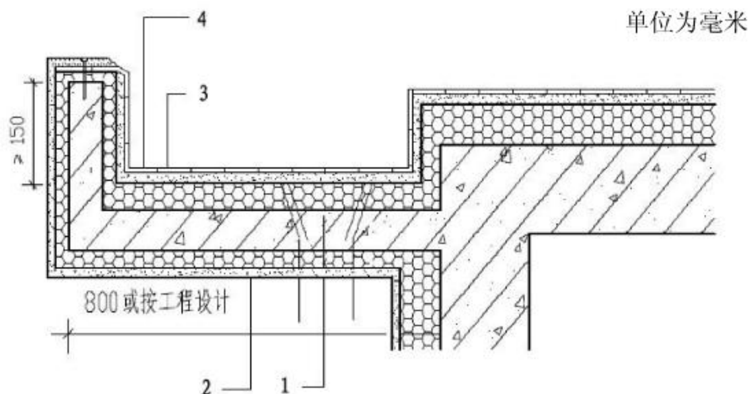
图 7 卷材、涂膜防水屋面檐沟
