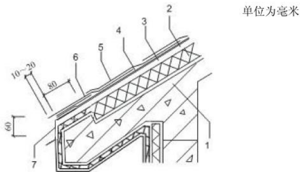
图 5 沥青瓦屋面檐口构造
