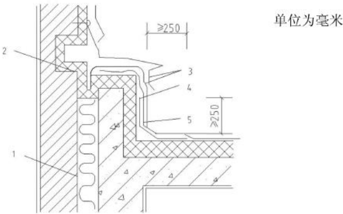
图 19 高低跨度变形缝
