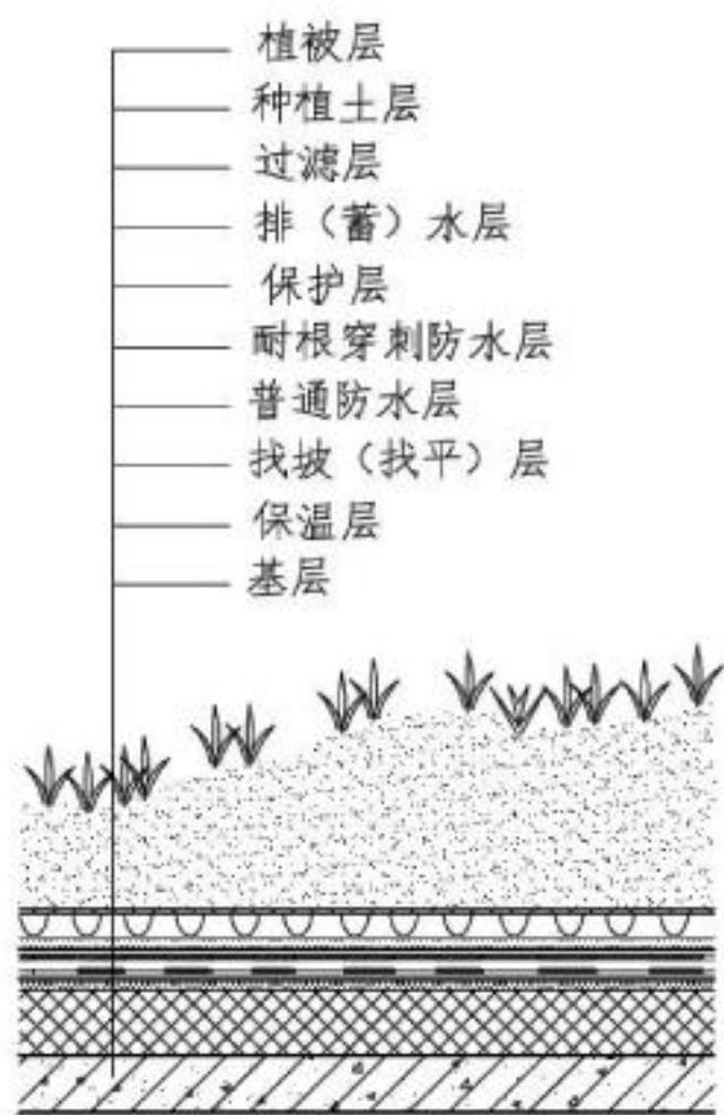
图 24 种植平屋面设计的基本构造层次
