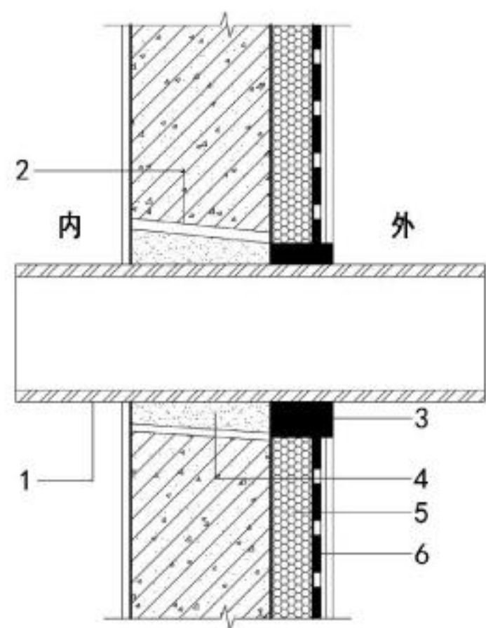
图 37 伸出外墙管道防水构造
