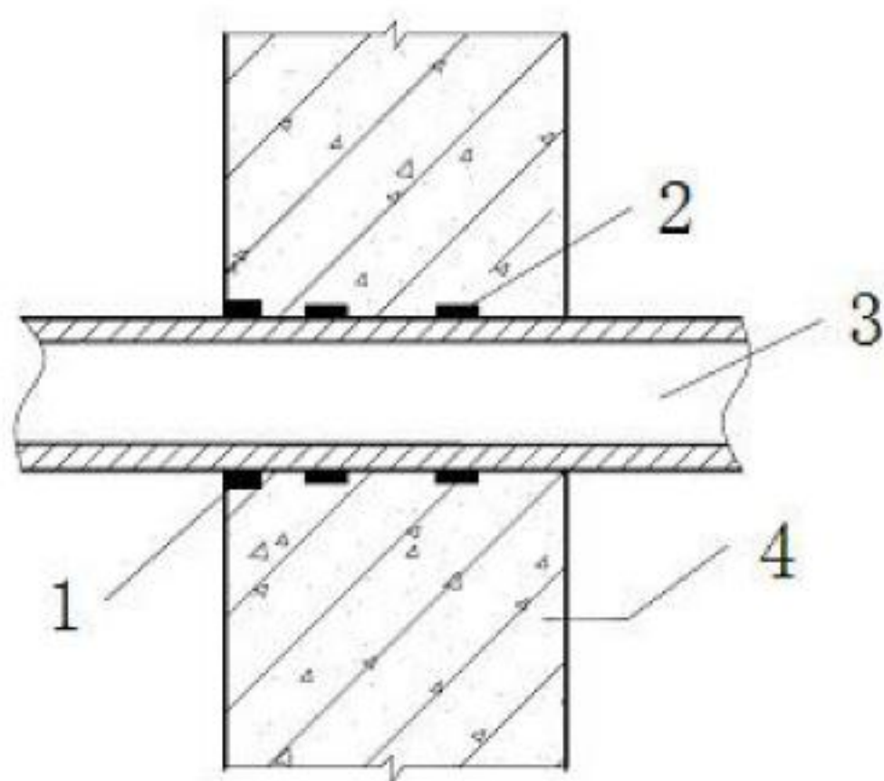
图 58 固定式穿墙管防水构造（二）
