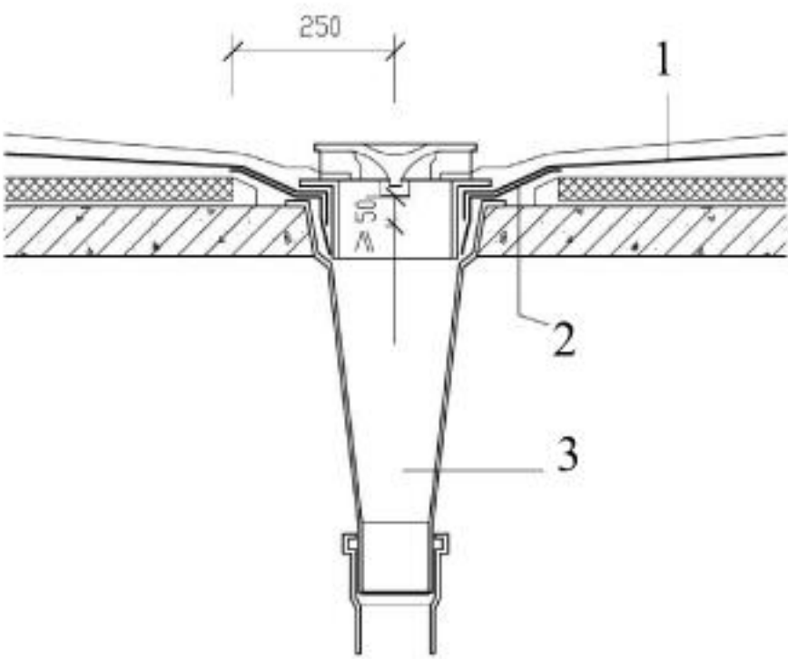
图 16 防直式水落口
