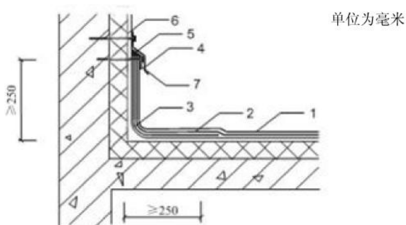
图 13 沥青瓦屋面山墙防水构造
