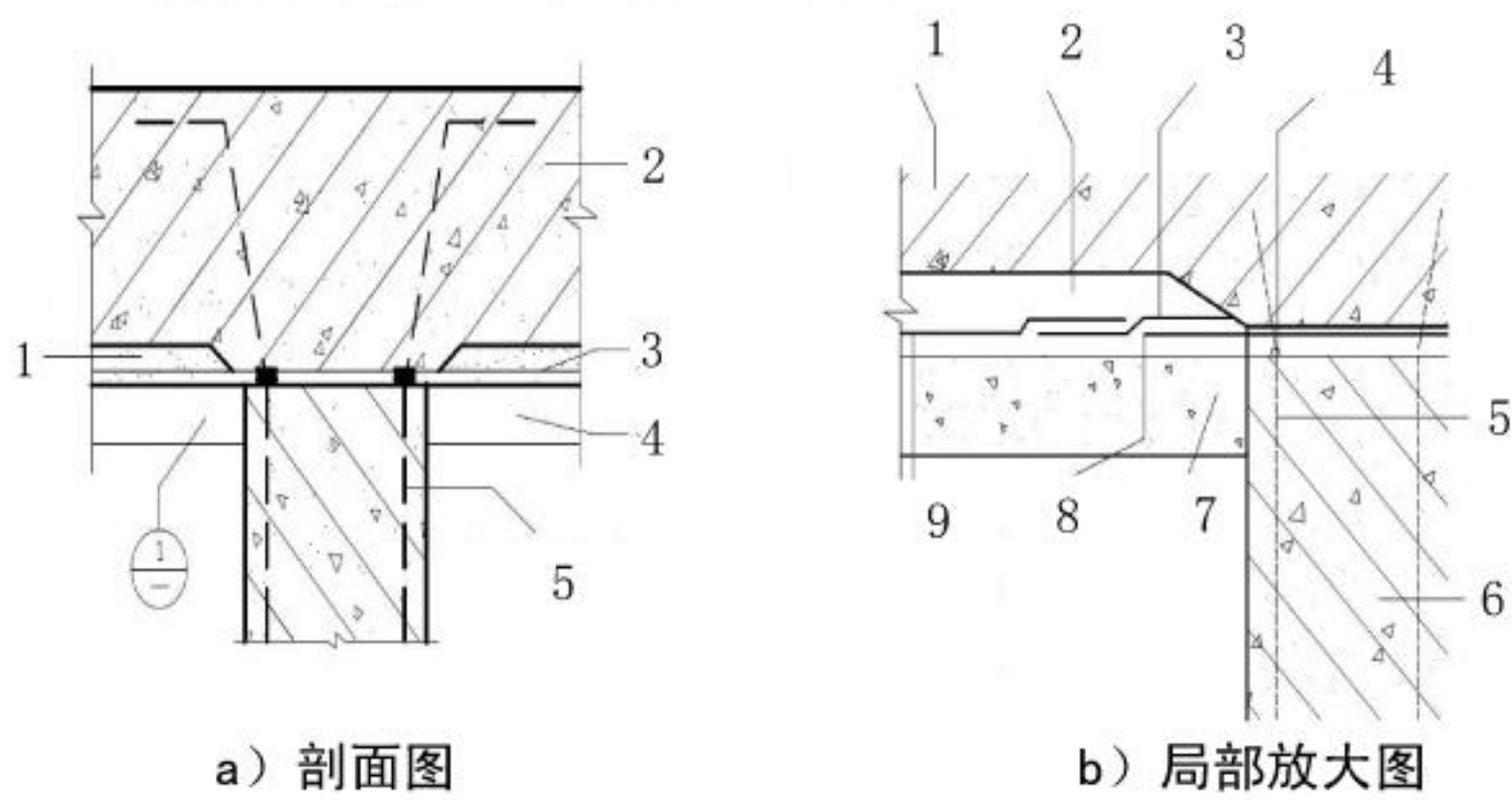
图 62 桩头防水构造（一）
