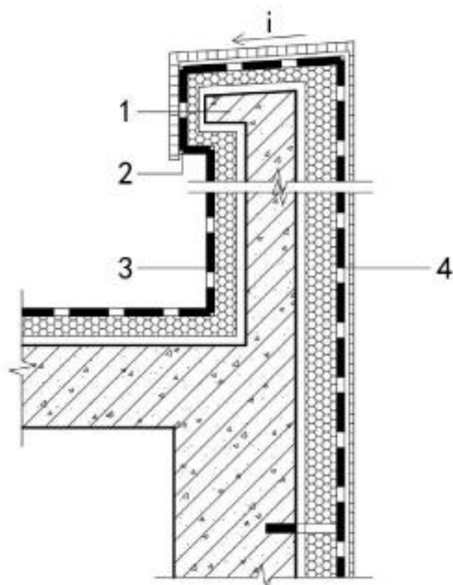
图 39 混凝土压顶女儿墙构造
