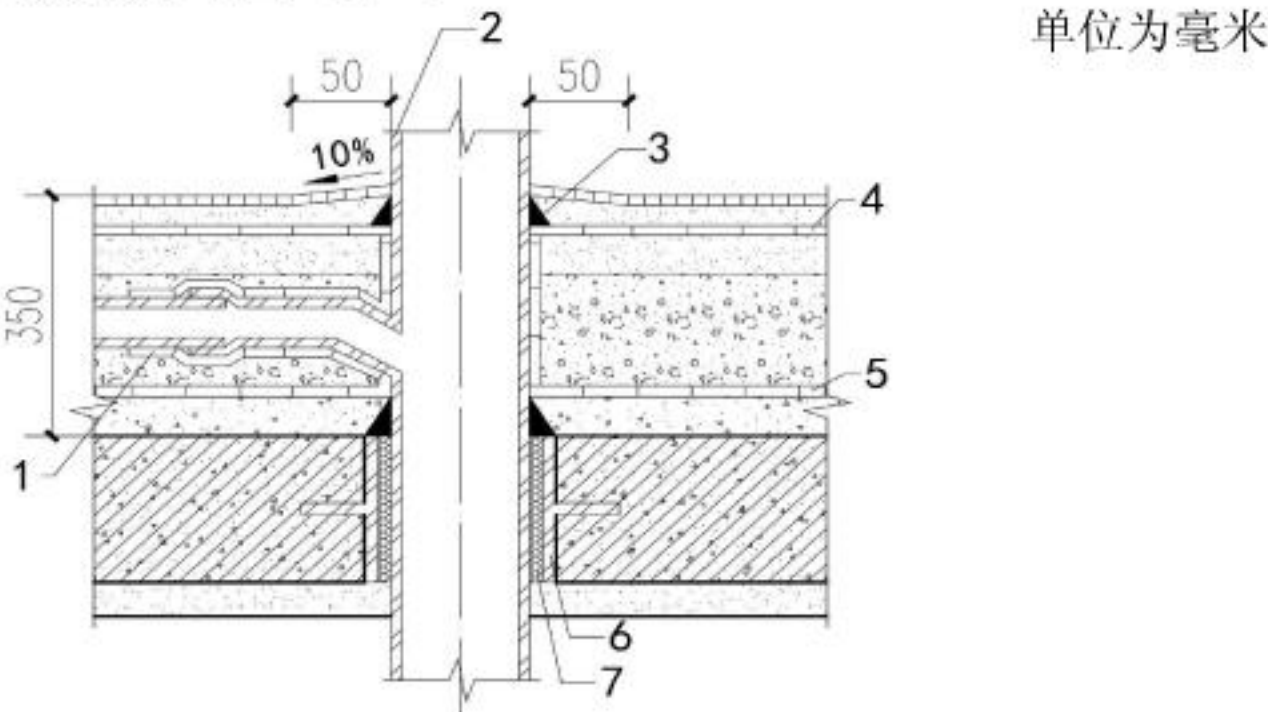
图 45 同层排水管道穿越楼板的防水构造
