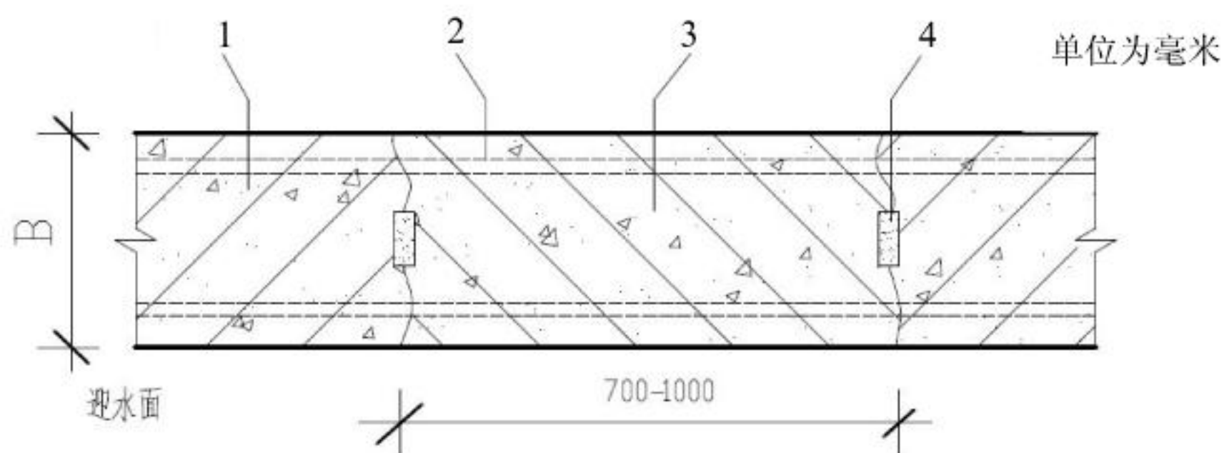
图 53 后浇带防水构造（一）
