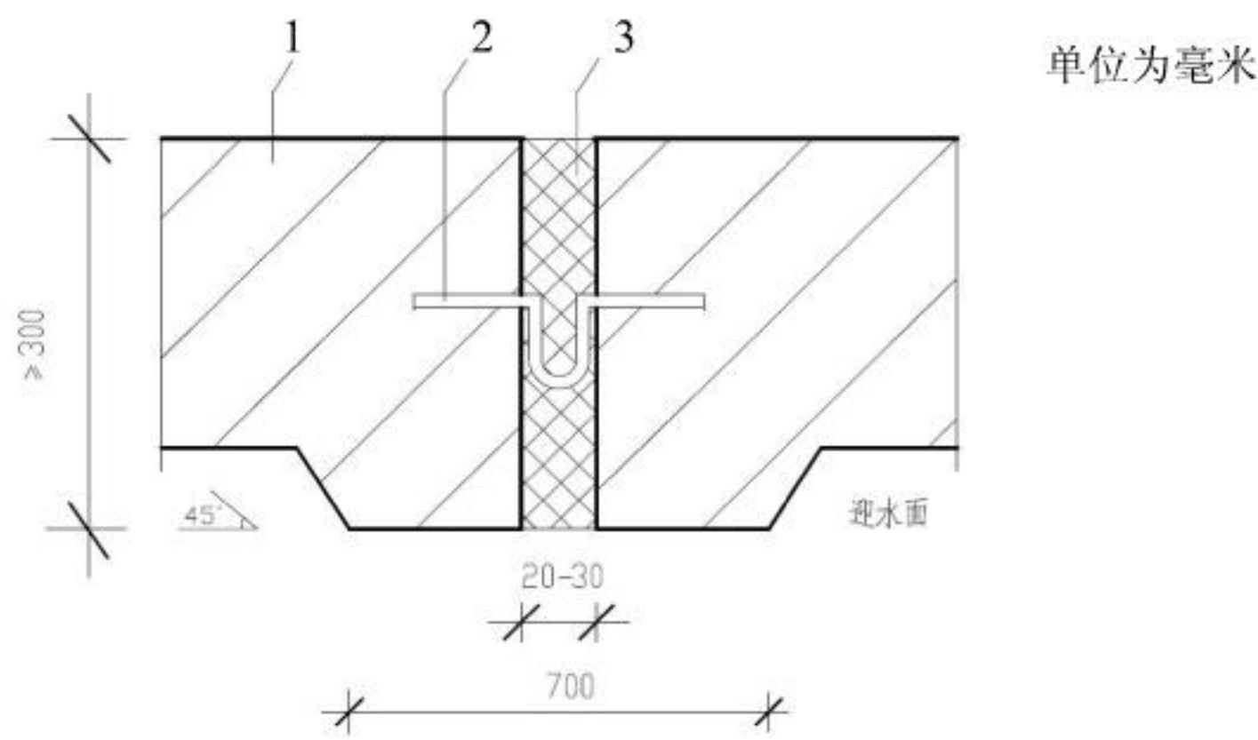
图 52 中埋式金属止水带
