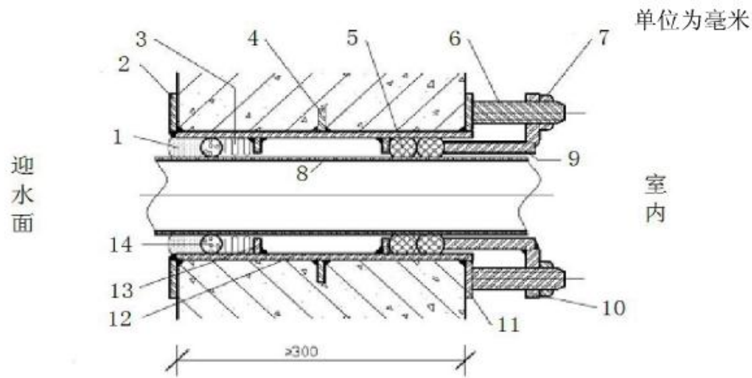
图 59 套管式穿墙管防水构造
