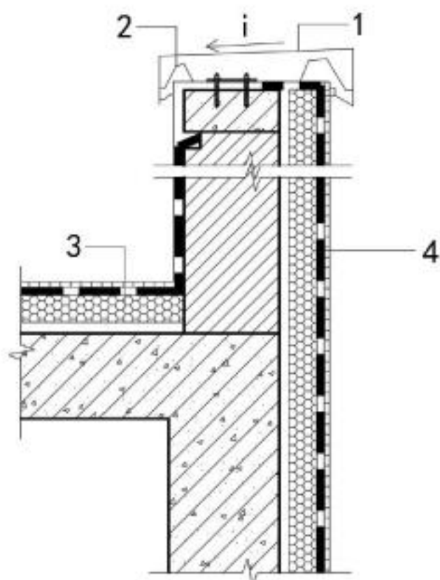
图 40 金属压顶女儿墙构造
