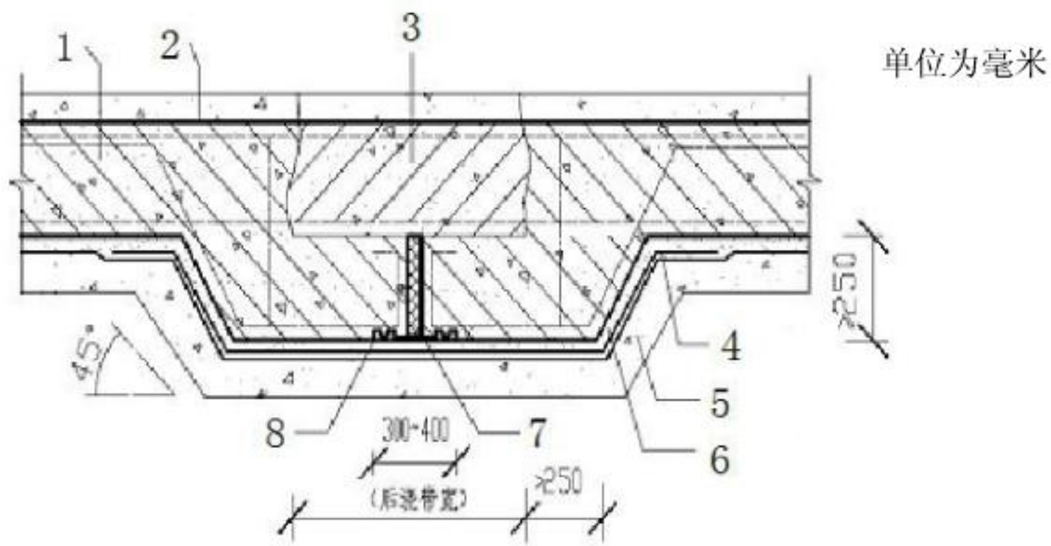
图 56 后浇带超前止水构造
