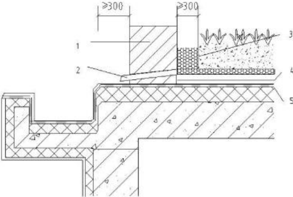
图 25 种植平屋面设计的基本构造层次
