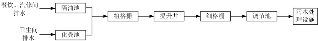
图8 预处理工艺流程图
