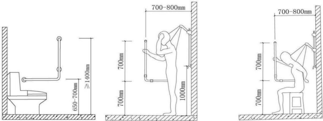
图8 L 型扶手
