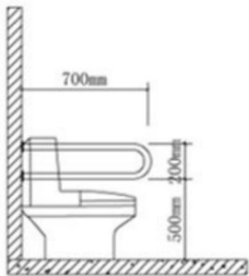
图10 U形扶手
