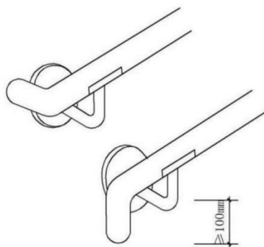
图5 扶手端头拐向墙侧或向下方弯曲
