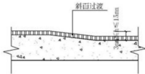
图2 斜面过渡处理
