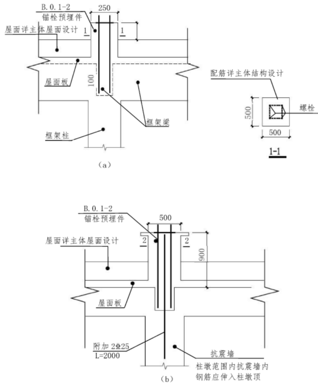
图 B.1 柱墩示意图
