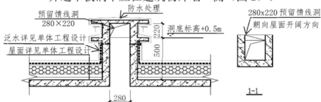
图 1 上线井道
