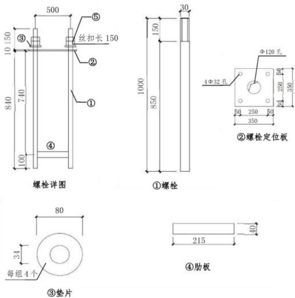
螺栓材料表
