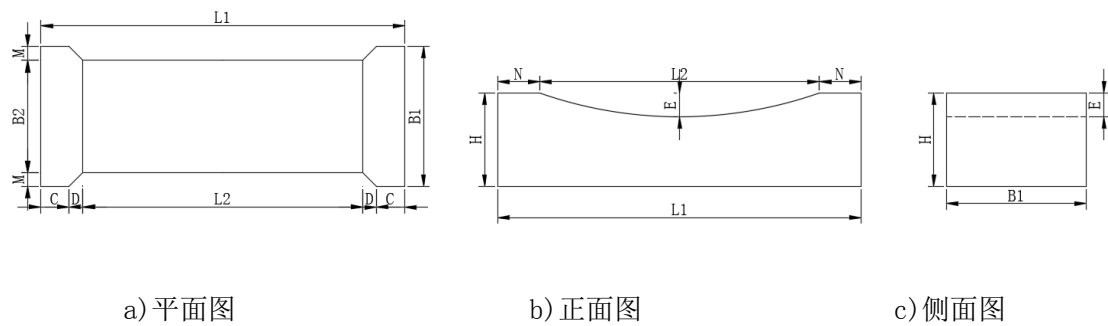
图 3 边沟盖板形状示意图
