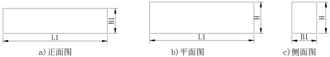
图 6 路平石形状示意图
