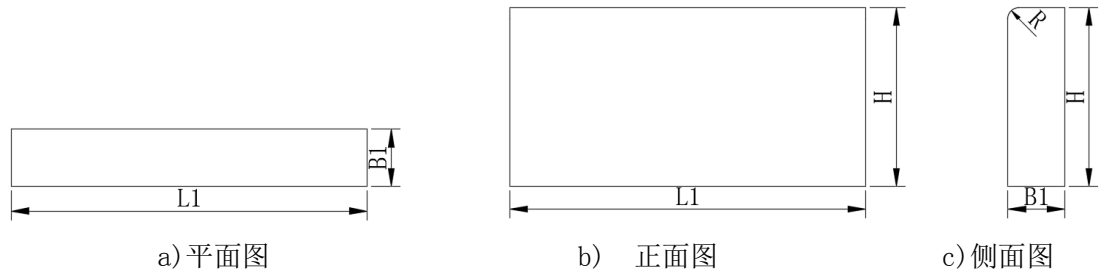
图 5 路缘石形状示意图
