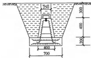
图 F.0.2 普通地面标石埋设 (mm)
