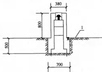
图 F.0.3 岩层墩标埋设 (mm)
