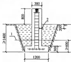
图 F.0.4 土层墩标埋设
