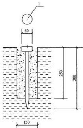
图 F.0.7 一二级控制点现场浇注标石造埋规格 (mm)
