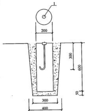
图 F.0.6 一二级控制点预制混凝土标石造埋规格 (mm)
