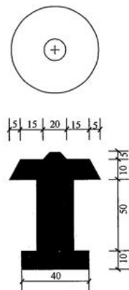
图 F.0.1 GNSS 控制点标志 (mm)
