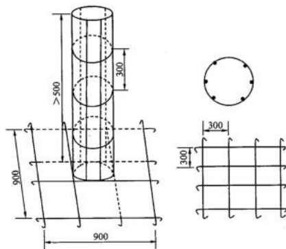
图 C.0.4 观测墩配筋 (mm)
