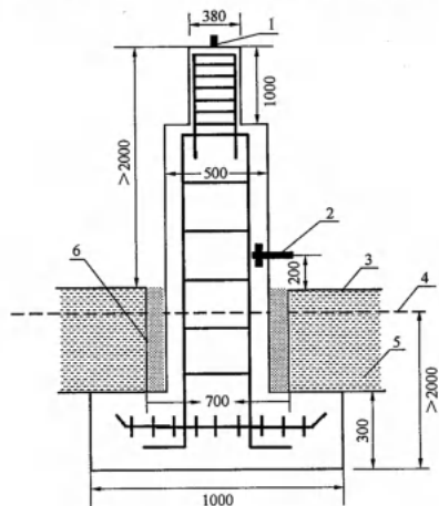
图 C.0.2 土层观测墩 (mm)
