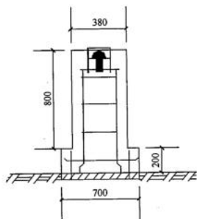
图 F.0.5 楼顶墩标埋设 (mm)
