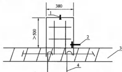
图 C.0.3 屋顶观测墩 (mm)
