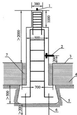
图 C.0.1 基岩（岩层）观测墩 (mm)
