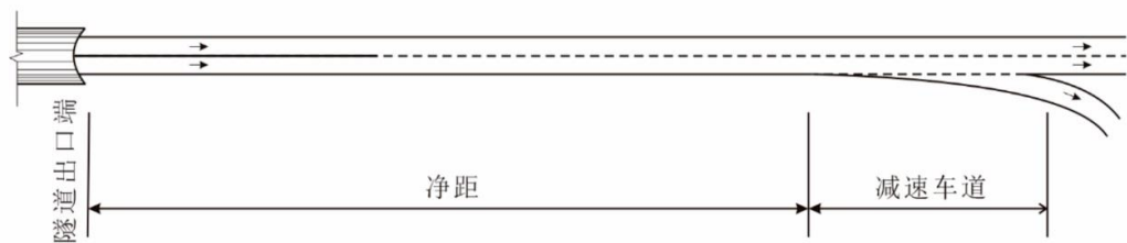
图16 隧道与前方互通式立体交叉出口之间的净距示意图
