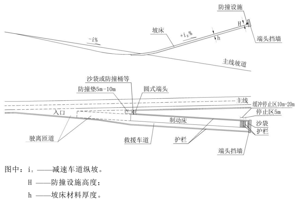
图1 避险车道设置示意图
