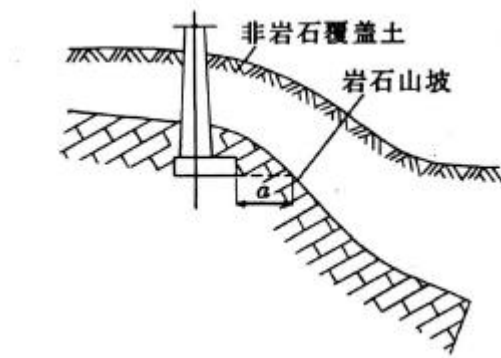
图4 岩石山坡基础前缘的安全距离
