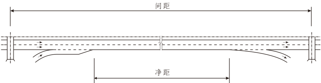
图14 互通式立体交叉与服务区、停车区之间的净距示意图
