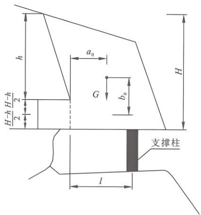
图 M.1 后缘有陡倾裂隙坠落式崩塌支撑体反力计算示意图
