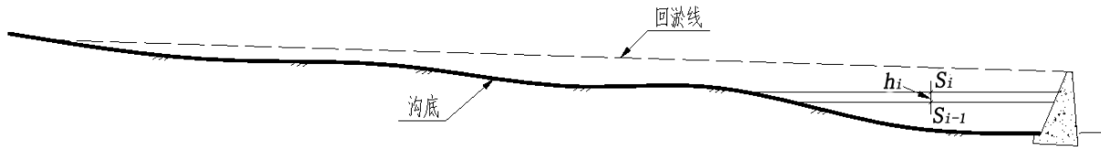
图 L.1 用等高线法计算拦挡坝库容纵断面
