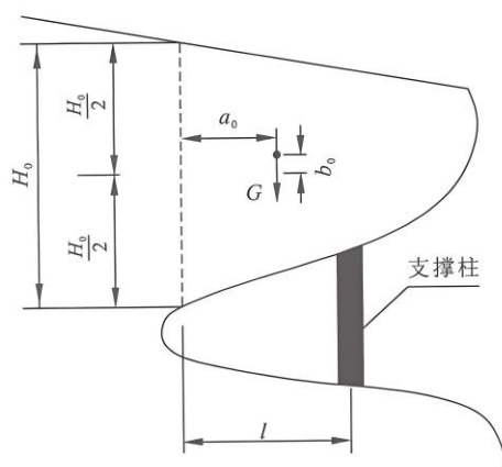
图 M.2 后缘无陡倾裂隙的坠落式岩墙支撑体反力计算示意图
