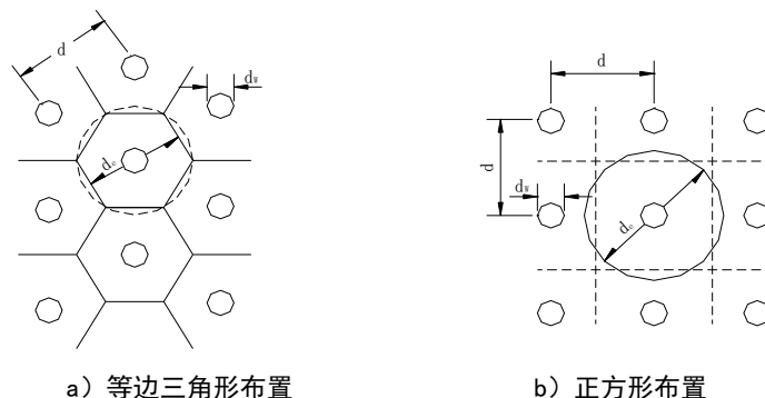
图5 排水体的布置形式
