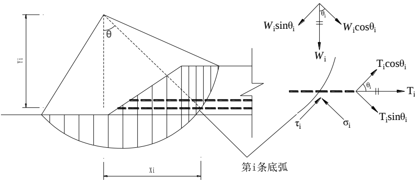
图3 圆弧滑动法稳定验算示意图
