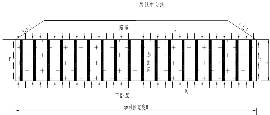
图6 等效实体法计算简图
