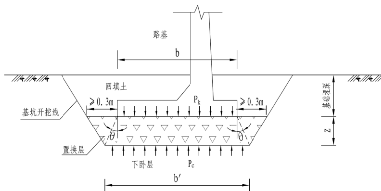
图1 附加应力计算示意图
