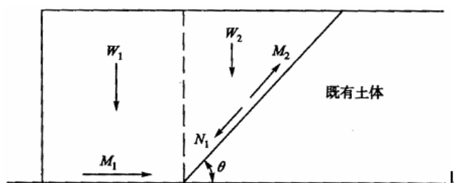
图7 泡沫混凝土底面抗滑稳定性验算示意图
