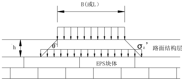
图9 竖向应力计算示意图
