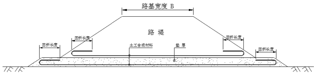
图2 土工合成材料加筋布置设计示意图
