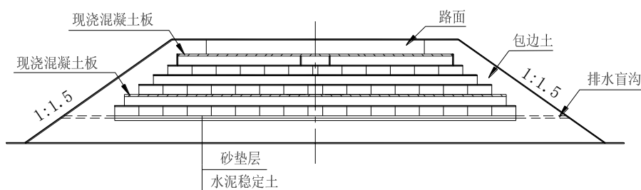
图8 EPS 块体轻质路堤典型横断面示意图
