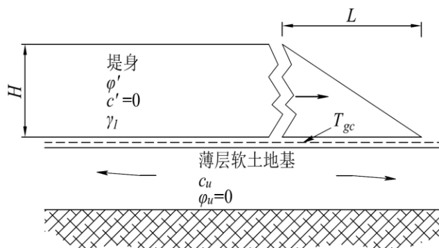
图4 薄层软土水平滑动稳定验算示意图
