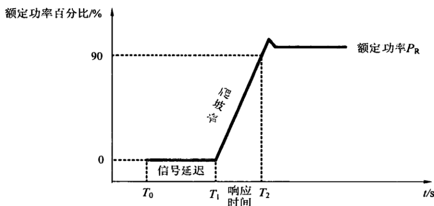
图 2 爬坡率和响应时间
