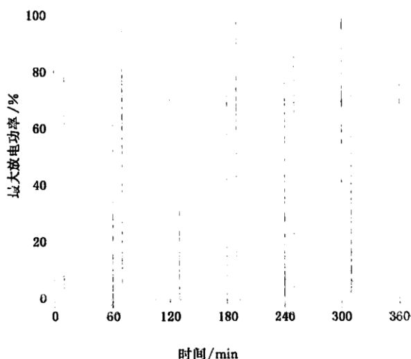
c) 持续放电 10 min 的 6 h 电压暂降治理典型工作周期
