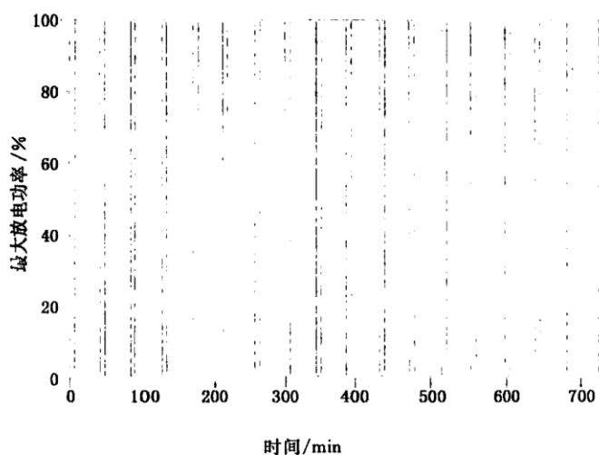
b) 持续放电 5 min 的 12 h 电压暂降治理典型工作周期
