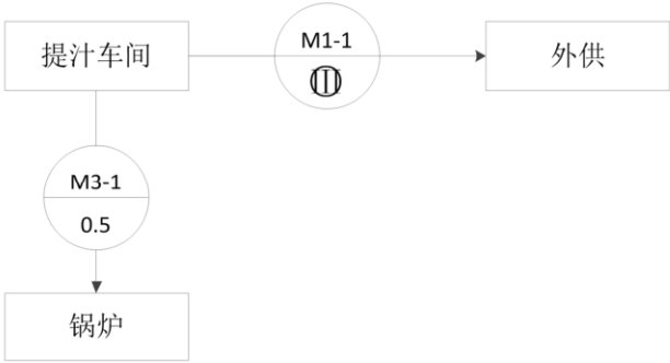
图 A.3 蔗渣计量采集点网络图（外供，汽车衡）
