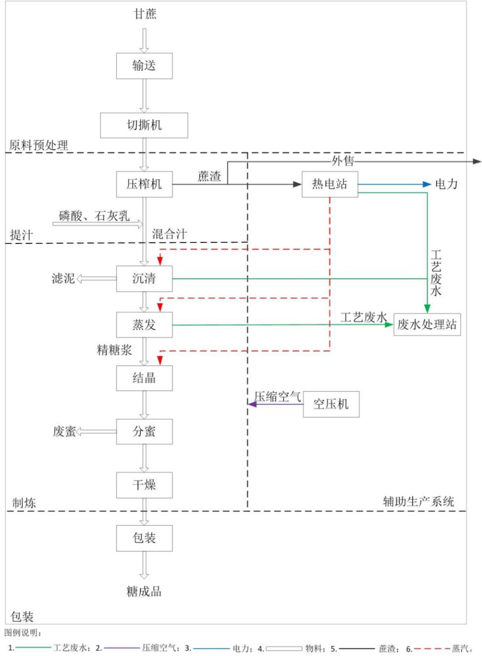
图 A.1 甘蔗制糖企业生产界区及工艺流程示意图
