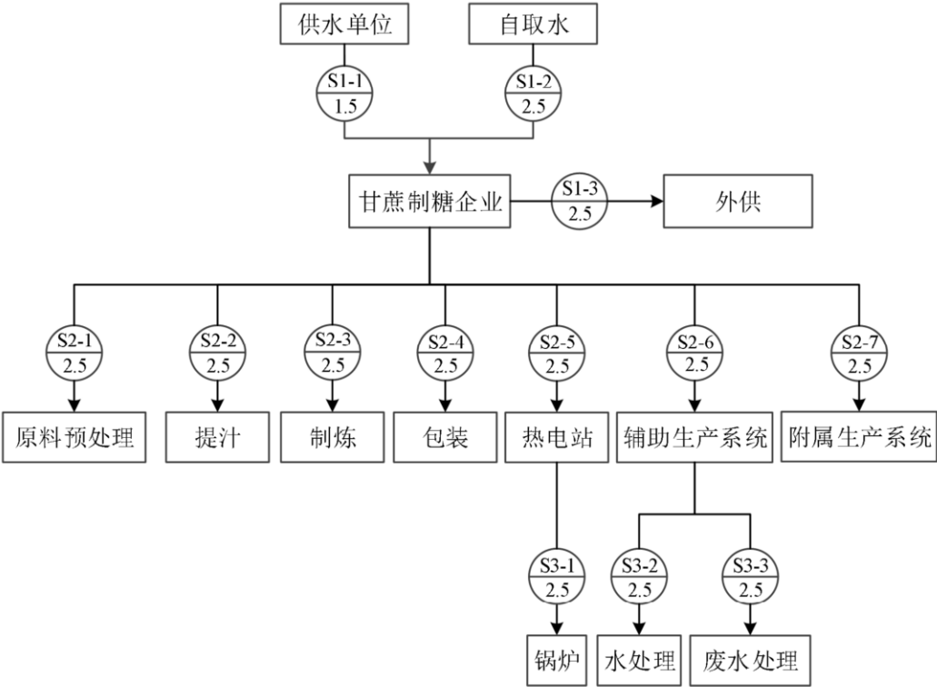
图 A.6 水计量采集点网络图
