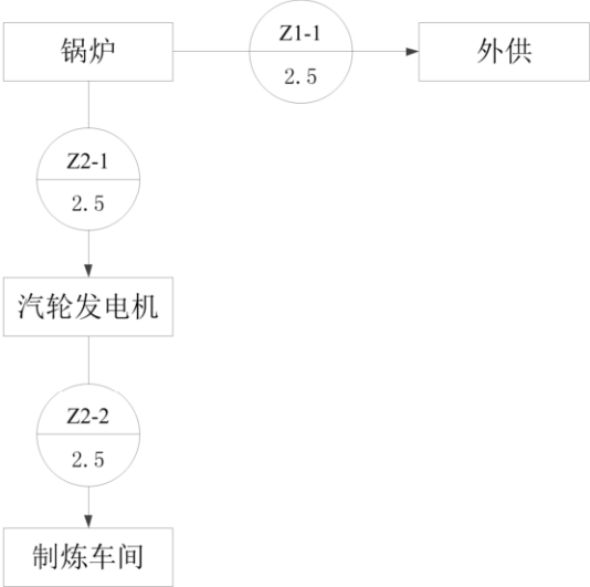
图 A.4 蒸汽计量采集点网络图
