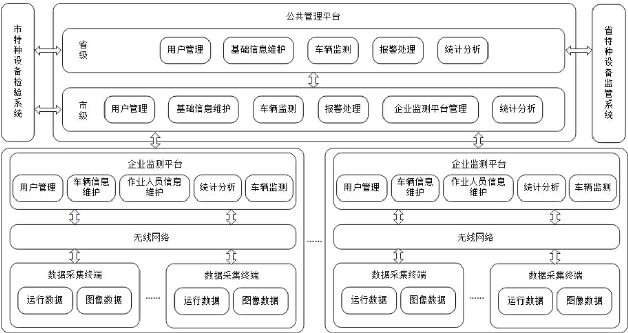
图 1 场车运行监测系统总体架构
