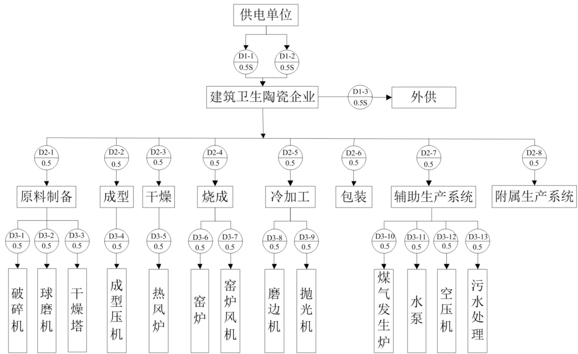
图 A.5 电力计量采集点网络图
