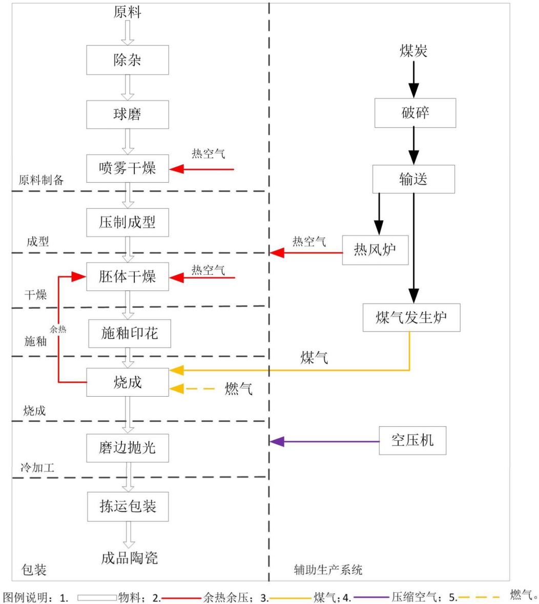
图 A.1 建筑陶瓷企业生产界区及生产工艺流程图
