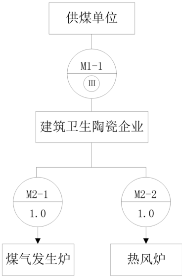
图 A.4 煤炭计量采集点网络图
