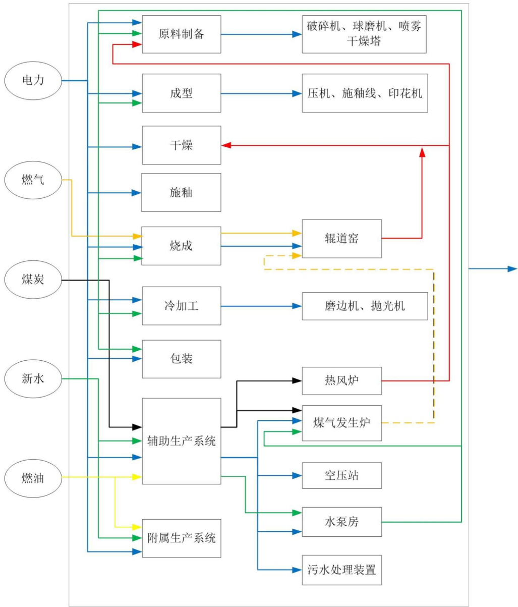
图例说明： 1. ——— 电力； 2. ——— 燃气； 3. ——— 燃煤； 4. ——— 新水； 5. ——— 燃油； 6. - - - 煤气； 7. ——— 余热余压。
