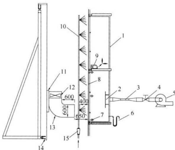
图 E.0.2 幕墙物理四性现场检测示意
