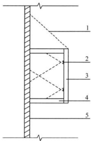
图 D.0.2 幕墙淋水试验装置示意
