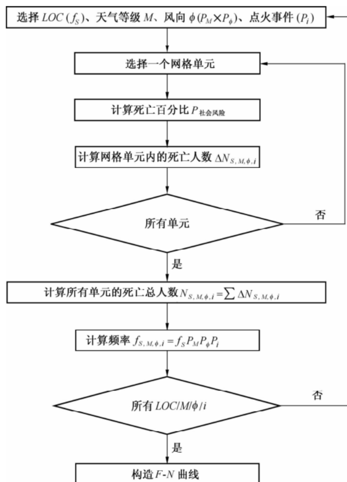
图 2 社会风险计算流程
