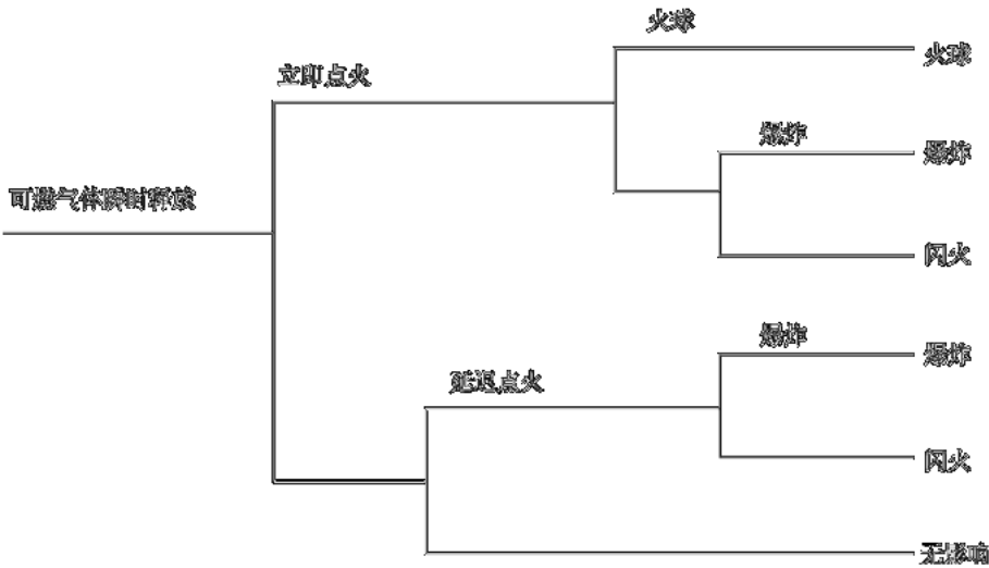
图 G.1 可燃气体瞬时释放事件树
