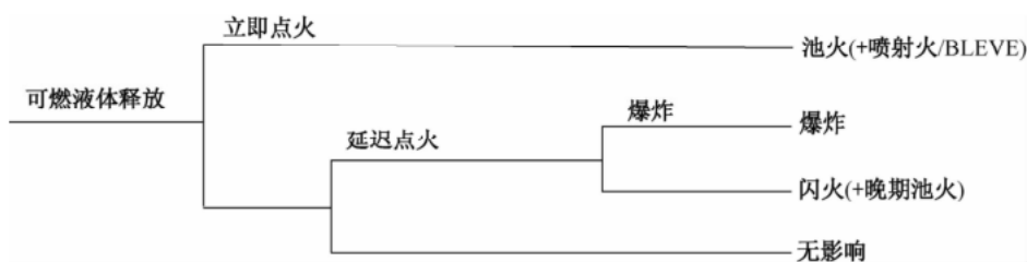
图 G.5 可燃液体释放事件树
