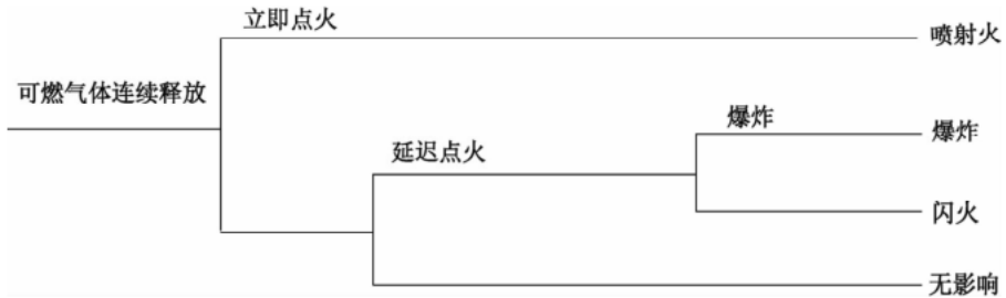
图 G.2 可燃气体连续释放事件树
