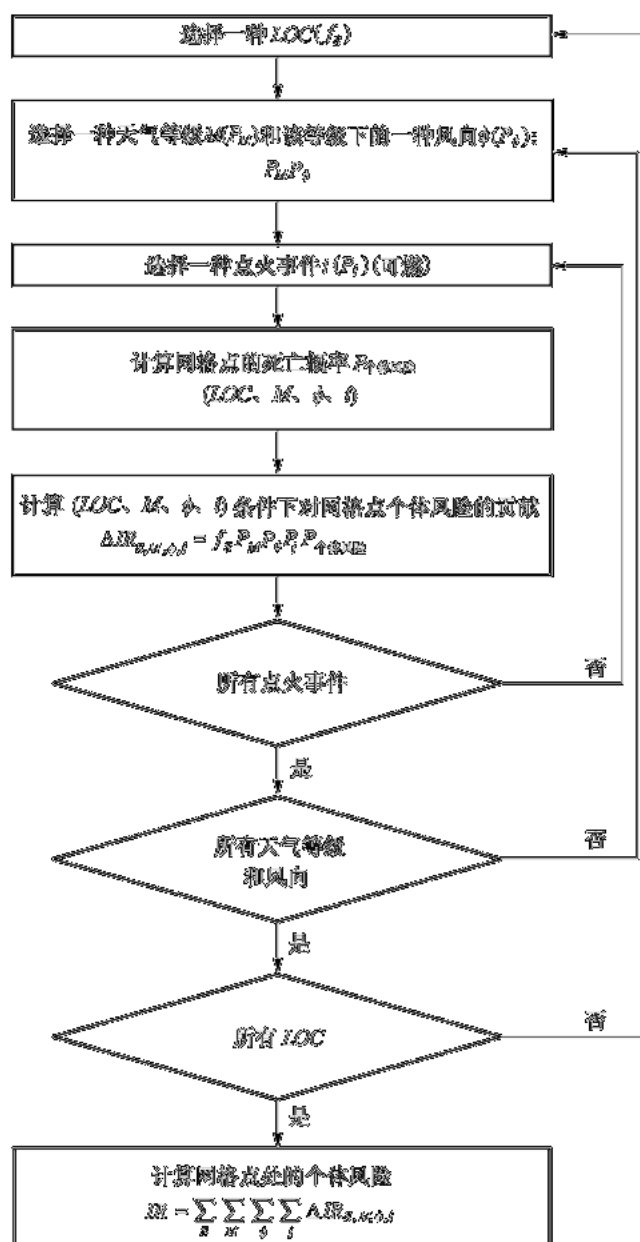
图 1 网格点处的个体风险计算程序
