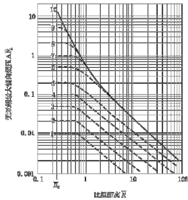
图 E.1 TNO 模型的 Sachs 比拟爆炸超压
