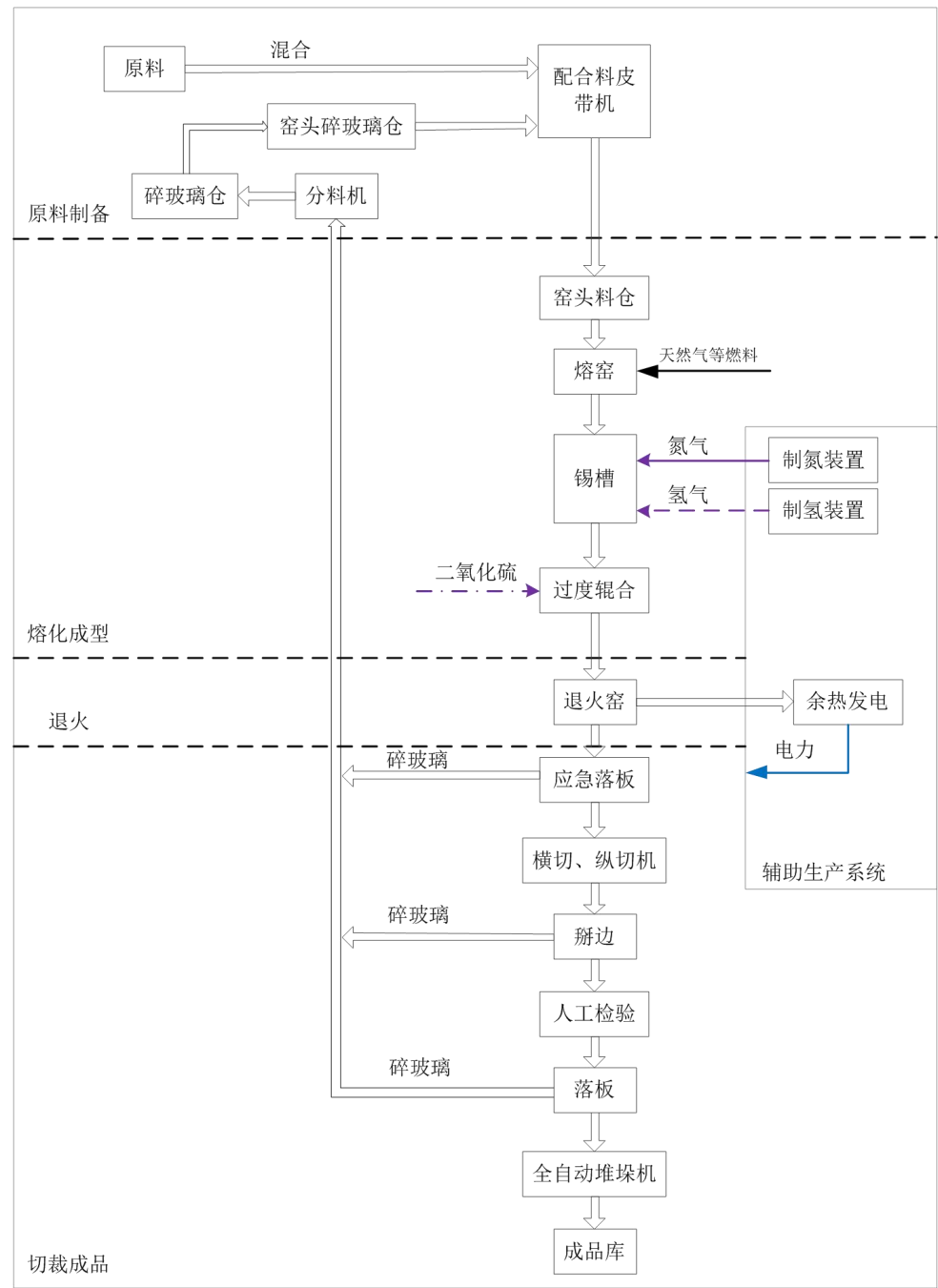
图 A.1 平板玻璃企业生产界区及生产工艺流程图
