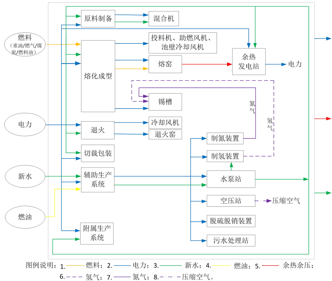
图 A.2 平板玻璃企业能源流向图
