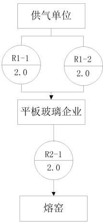
图 A.3 燃气计量采集点网络图
