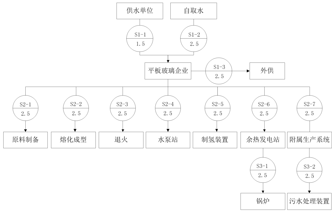
图 A.5 水计量采集点网络图
