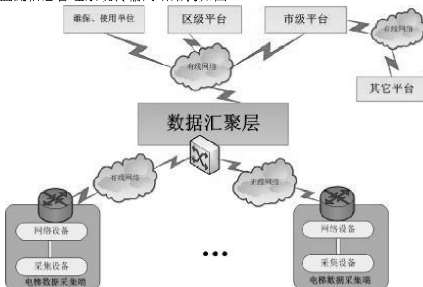
图2 电梯运行安全监测信息管理系统传输网络结构图
