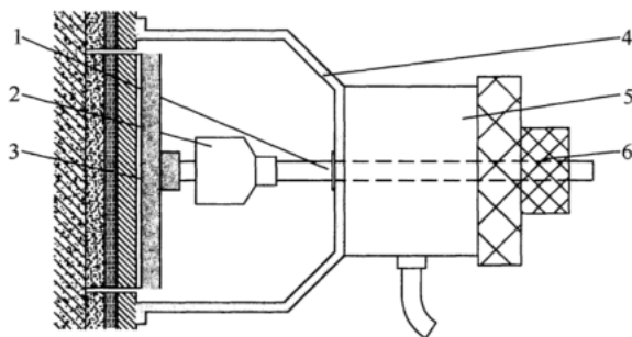
图 4.0.4 粘结强度检测仪安装示意
