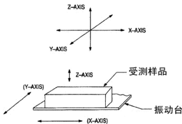
图3 试验件摆放安置示意图
