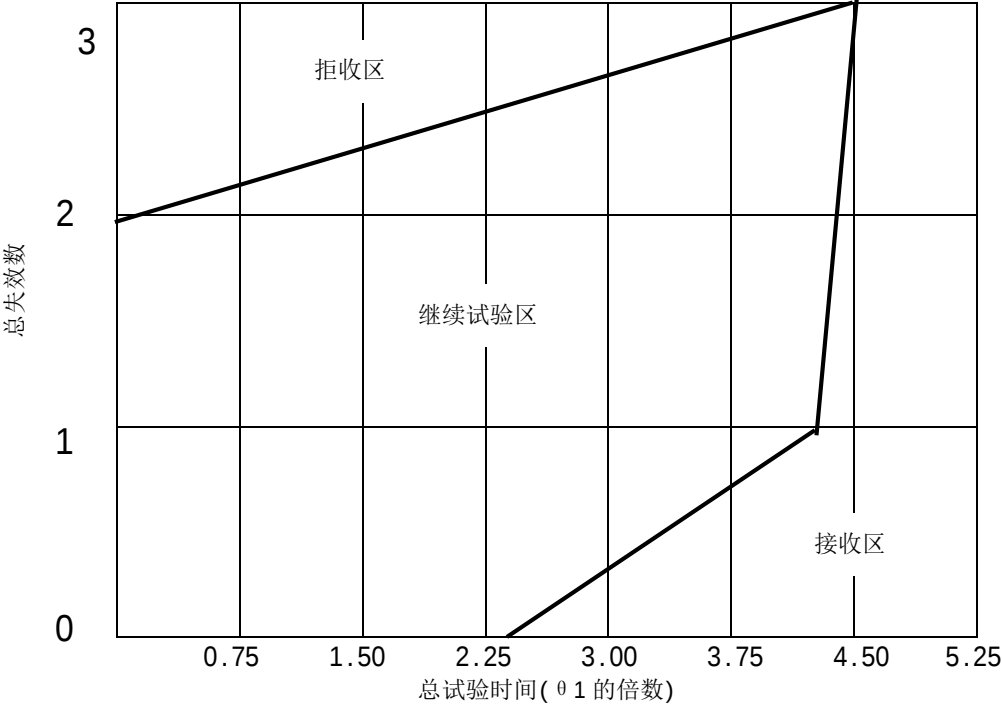
图A.2 试验方案 2 的判决标准图
