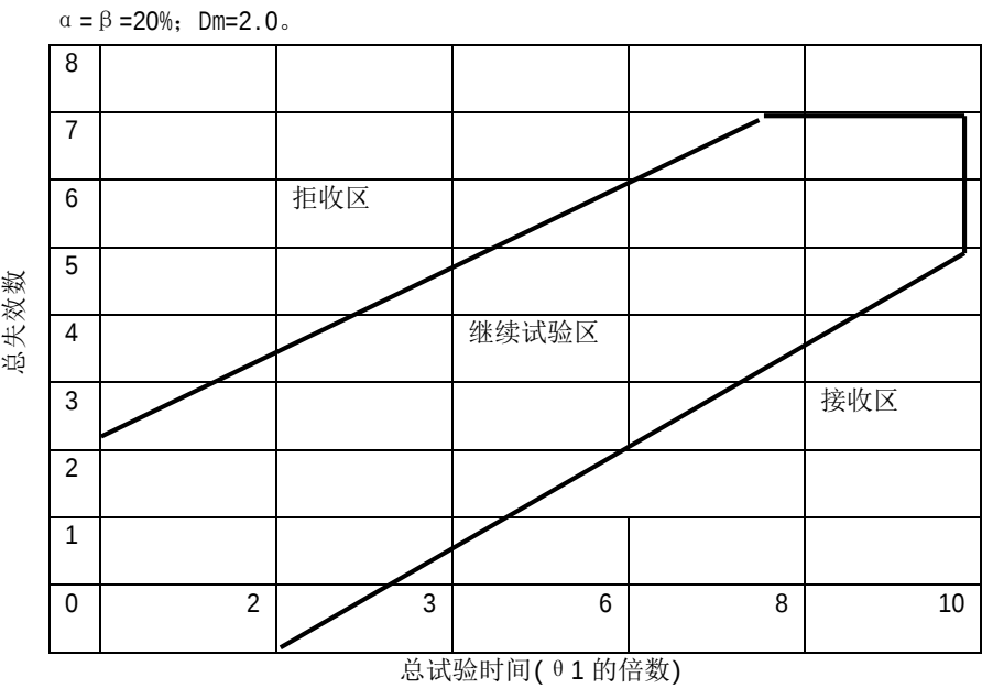
图A.1 试验方案 1 的判决标准图
