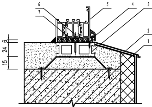
1——墙体，2——披水板，3——附框，4——附框压条，5——窗框，6——滑槽固定螺钉，7——滑动扣件
