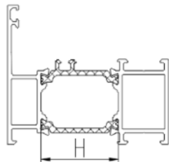
图4 聚酰胺隔热条截面尺寸示意图
