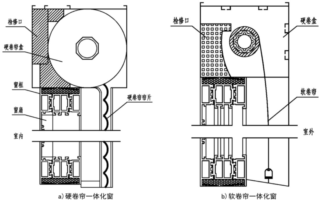
图A.2 外遮阳一体化窗示意图
