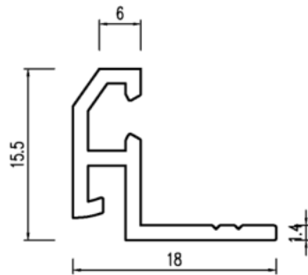
图7 附框压条示意图
