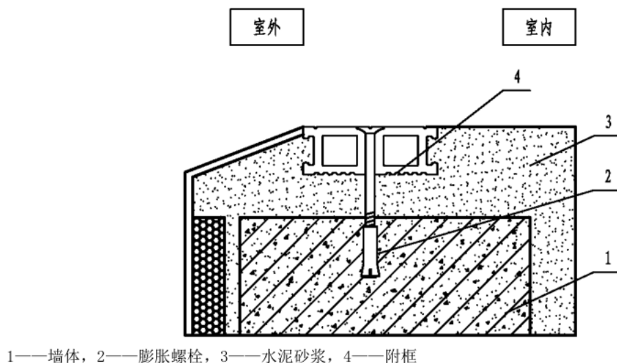
图13 改造居住建筑凹侧面附框安装构造示意图
