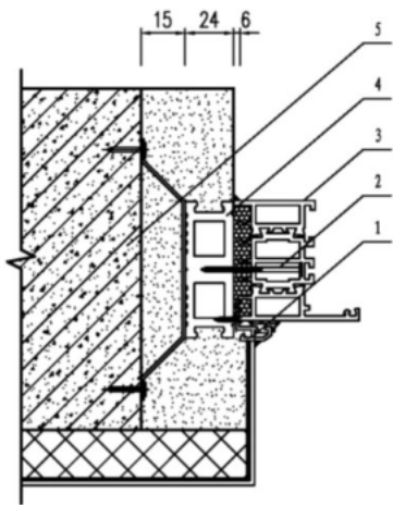
1——附框压条，2——固定螺钉，3——窗框，4——附框，5——墙体
