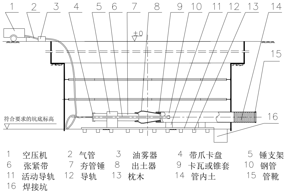
图 1 夯管施工连接示意图
