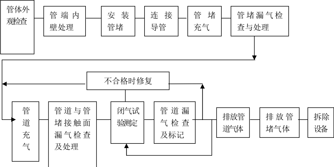
图 D.0.2 管道闭气试验流程示意框图
