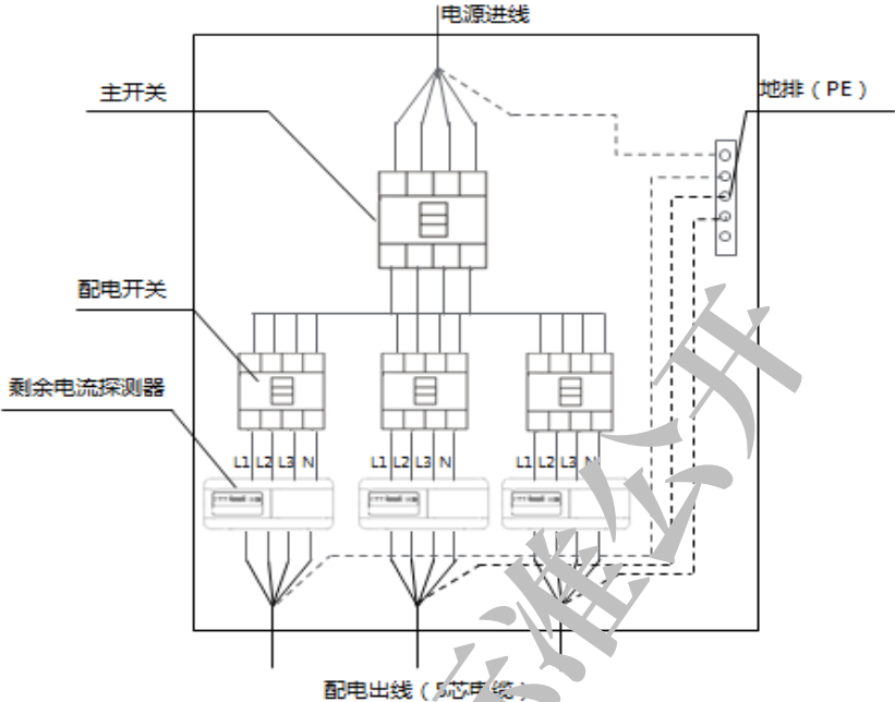
图C.1 剩余电流探测器安装在5芯配电出线开关下方的一次线接法
