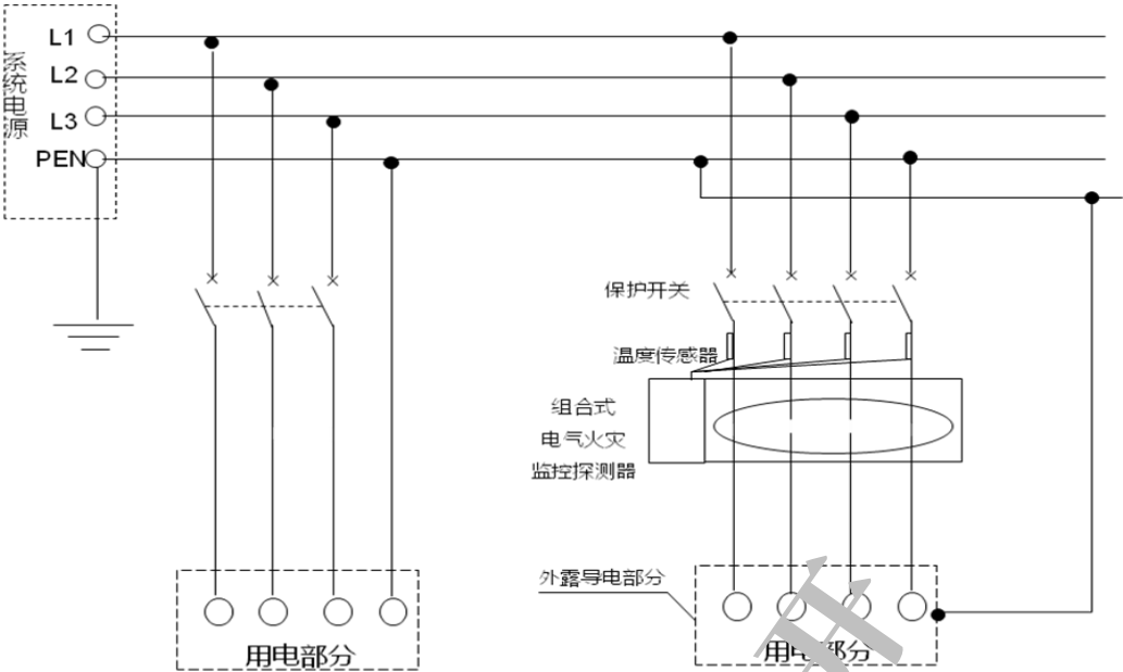
图B.3 TN-C-S系统
