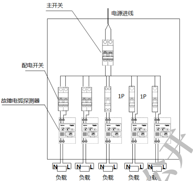
图C.3 WAFD故障电弧探测器安装在配电箱出线开关下方的一次线接法
