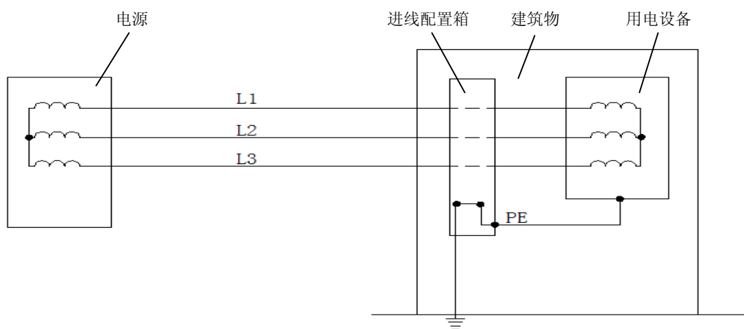
图 I.5 IT 系统
