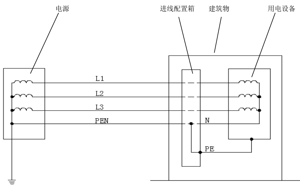
图 I. 2 TN-C-S 系统
