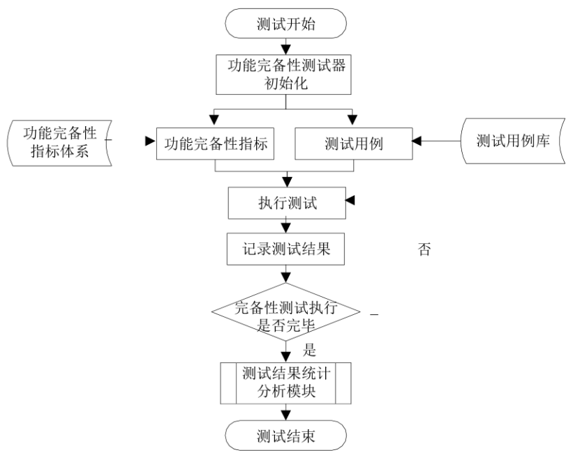
图2 企业资源管理软件功能完备性测试流程
