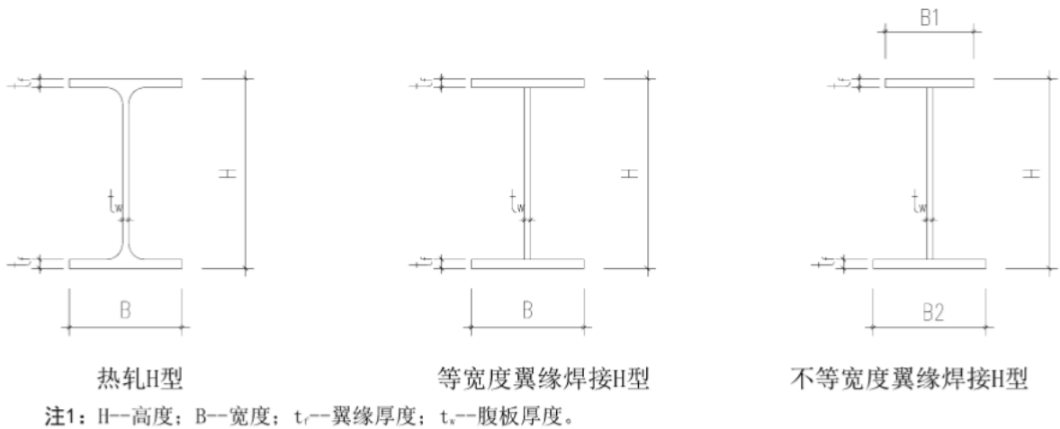
图1 H型钢梁截面形式
