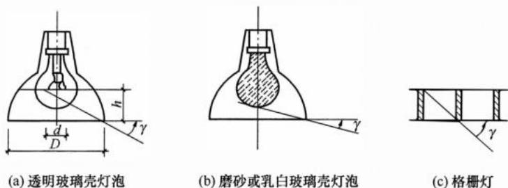
图 4 遮光角示意
