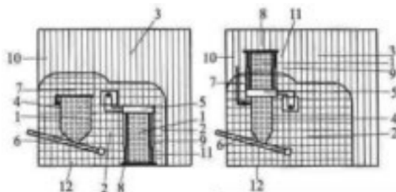
图 D.0.5 建筑物内的无抽气排风设施的圆筒翻斗装置
