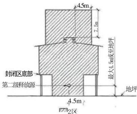
图B.0.1-8 可燃物质轻于空气、通风良好的压缩机厂房
