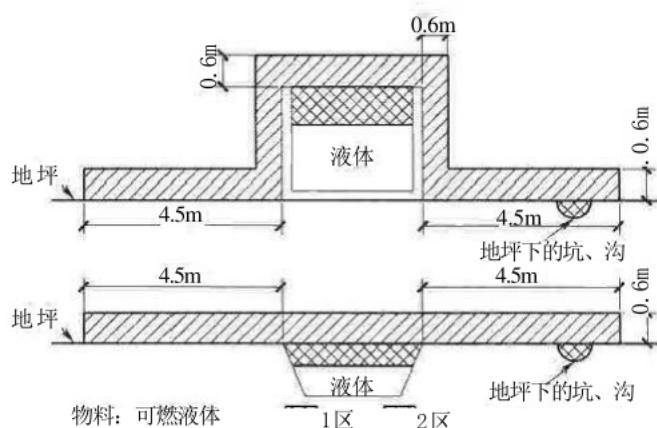
图 B.0.1-18 可燃性液体紧急集液池、油水分离池
