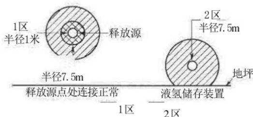
图 B.0.1-19 通风良好的户内或户外液氢储存装置
