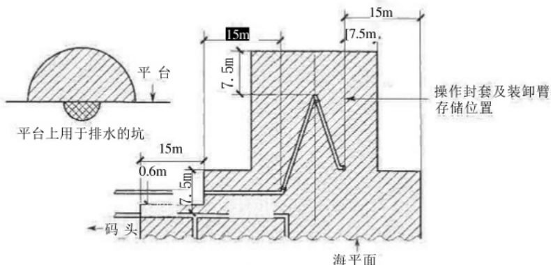
图 B.0.1-22 码头或水域处理可燃性液体的区域
