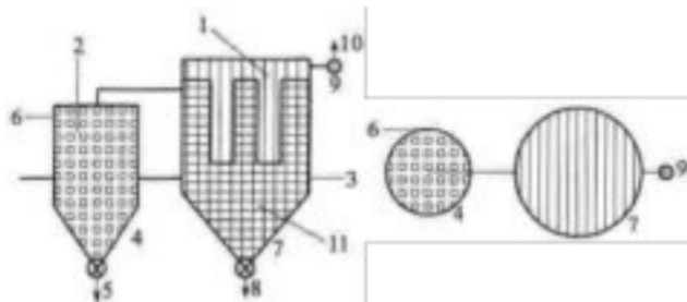
图D.0.4 建筑物外的旋风分离器和过滤器
