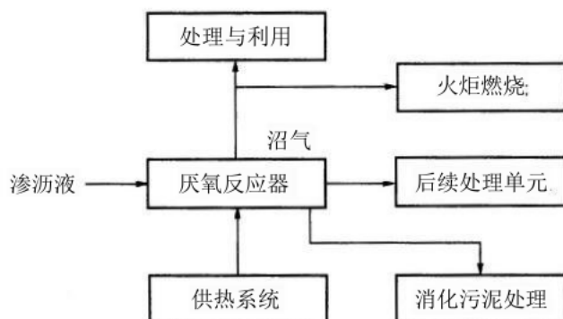
图5.4.1 厌氧生物处理系统工艺流程框图
