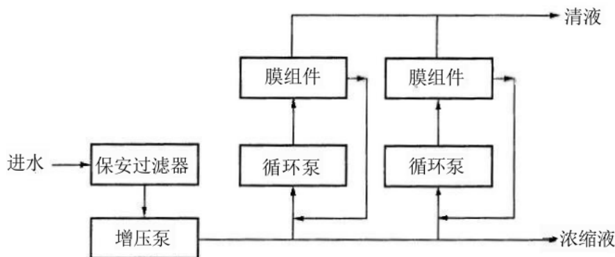
图5.7.1 反渗透系统流程框图
