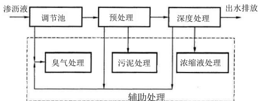
图 2 “预处理+深度处理”工艺流程框图
