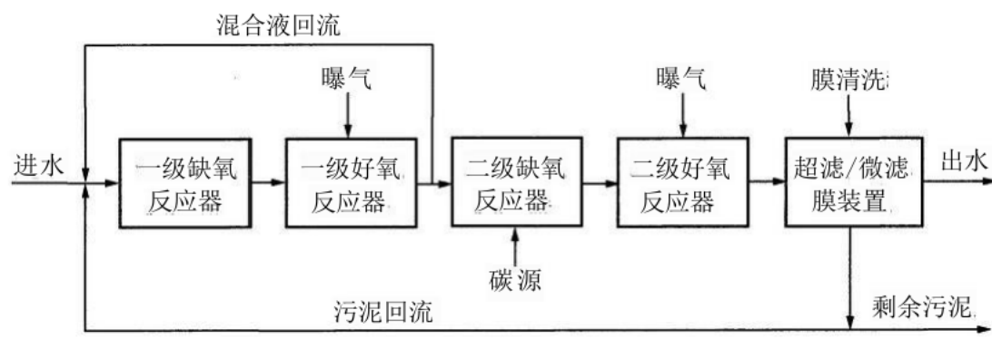
图5.5.3 强化生物处理 MBR 系统流程框图
