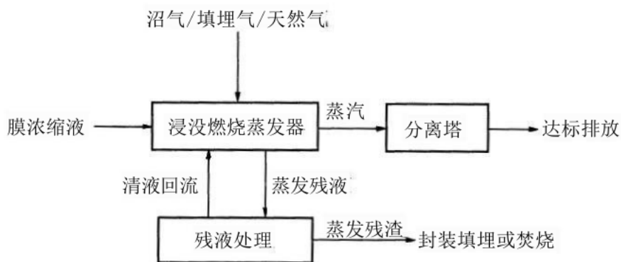
图5.10.1 浸没燃烧蒸发系统流程框图
