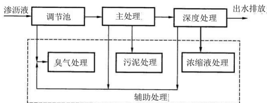
图 1 “主处理+深度处理”工艺流程框图
