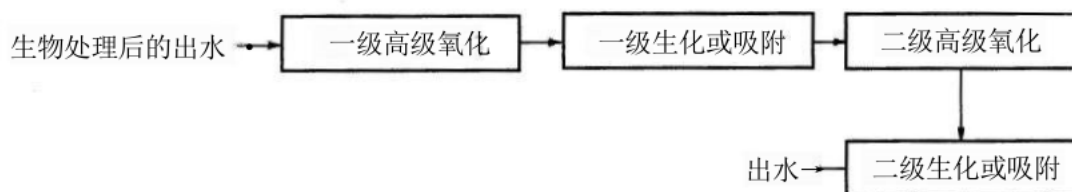
图5.8.2 高级氧化组合工艺流程框图
