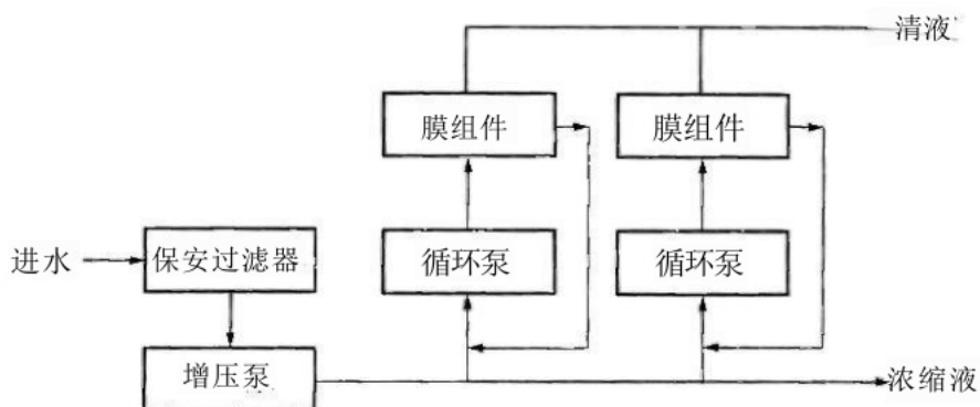
图5.6.1 纳滤系统流程框图
