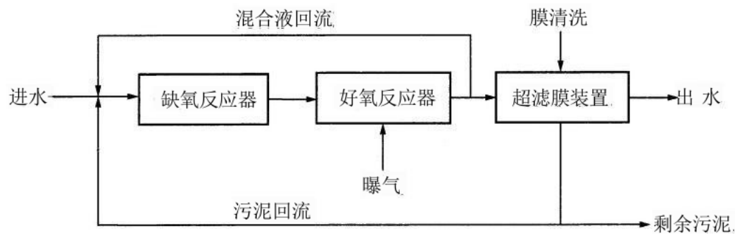
图5.5.2-1 外置式 MBR 系统流程框图
