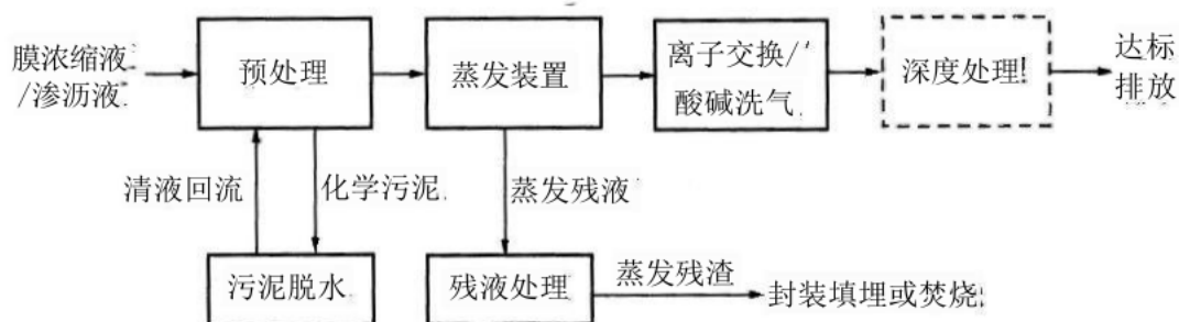
图5.9.1 机械蒸汽再压缩蒸发系统流程框图
