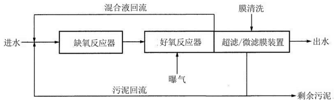
图5.5.2-2 内置式 MBR 系统流程框图
