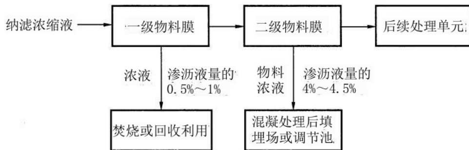
图 3 纳滤浓缩液减量化工艺流程框图
