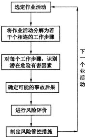
图 A.3 作业活动风险分析流程图
