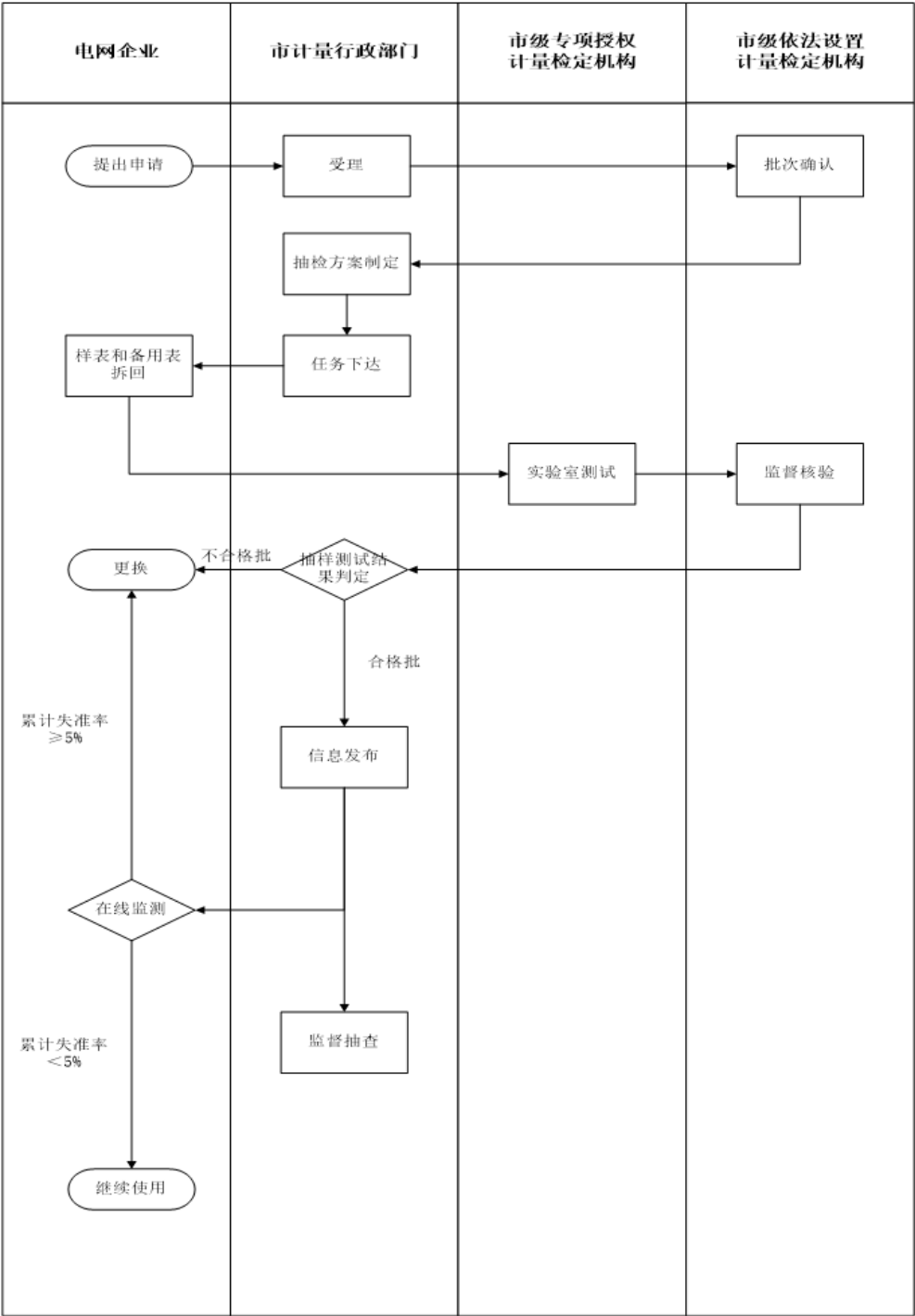
图A. 1 安装式交流电能表状态评价工作规范流程图
