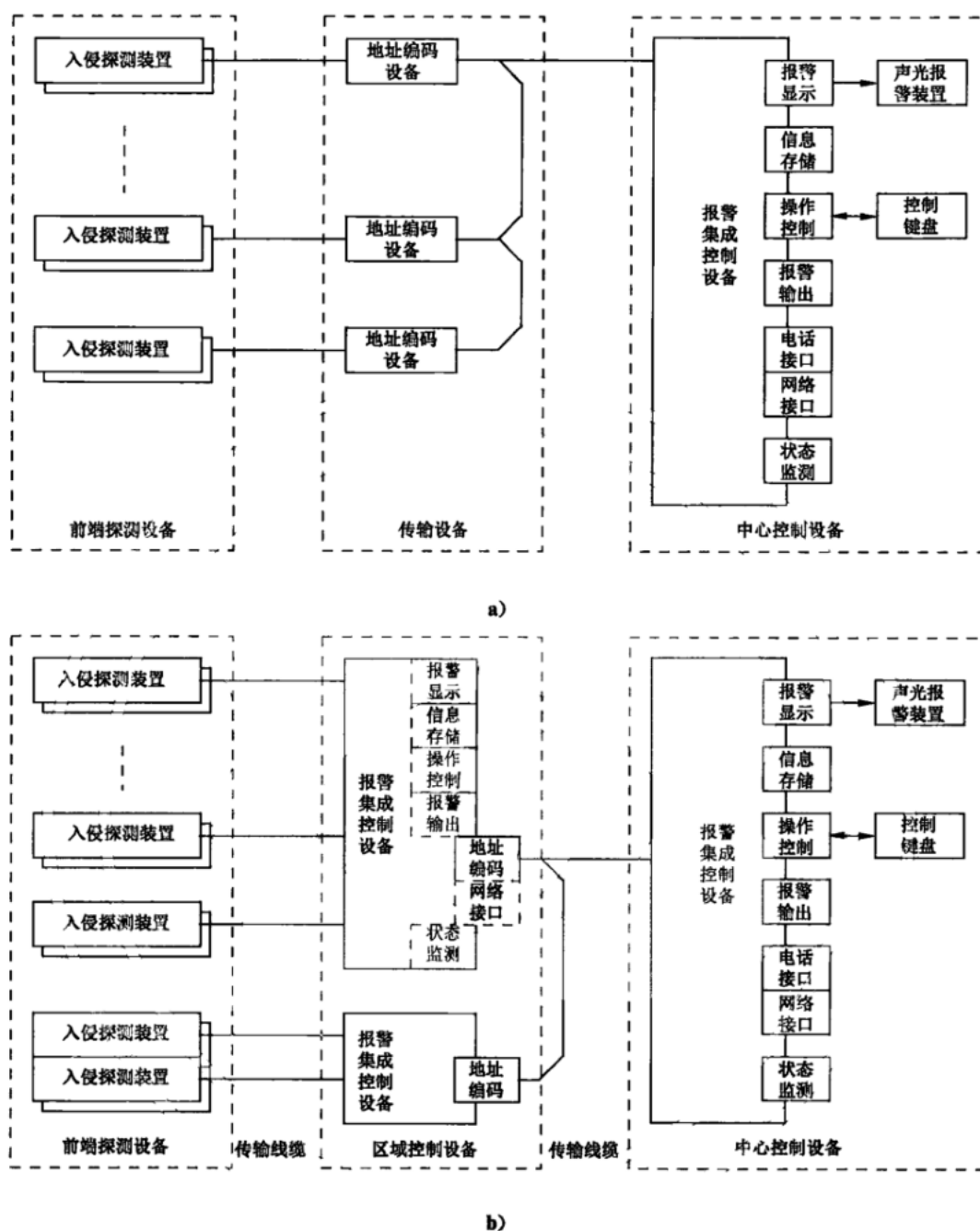
图 3 应用类型为总线制的入侵报警系统
