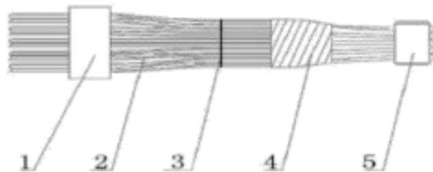
1. 梳束板（或锚具） 2.钢绞线 3.扎丝 4.绑扎胶带 5.牵引螺塞
