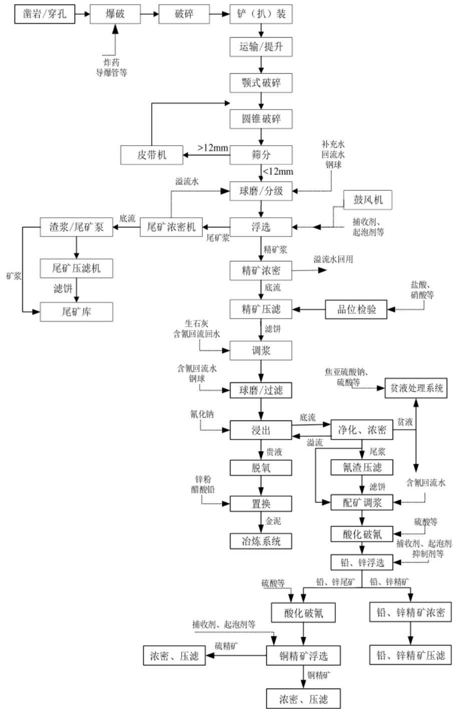
附 录 B (资料性附录) 黄金采选企业典型工艺流程图
