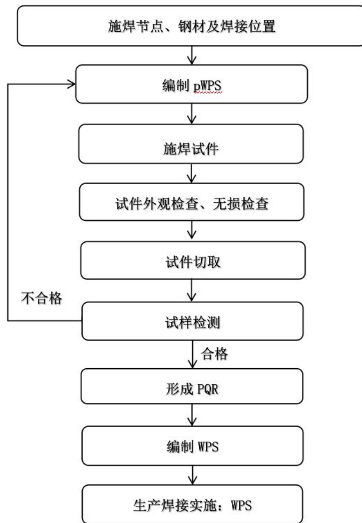
图 D.1.1 焊接工艺评定流程
