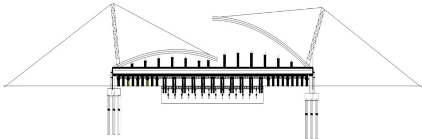
图 14.9.1-1 拱肋竖转施工示意图
