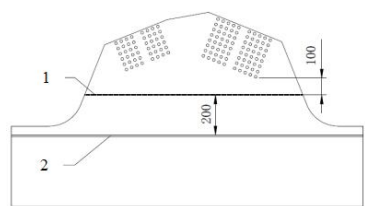
图 7.1.4-2 节点板焊缝错开的最小距离（尺寸单位：mm） 1 一焊缝； 2 一盖板
