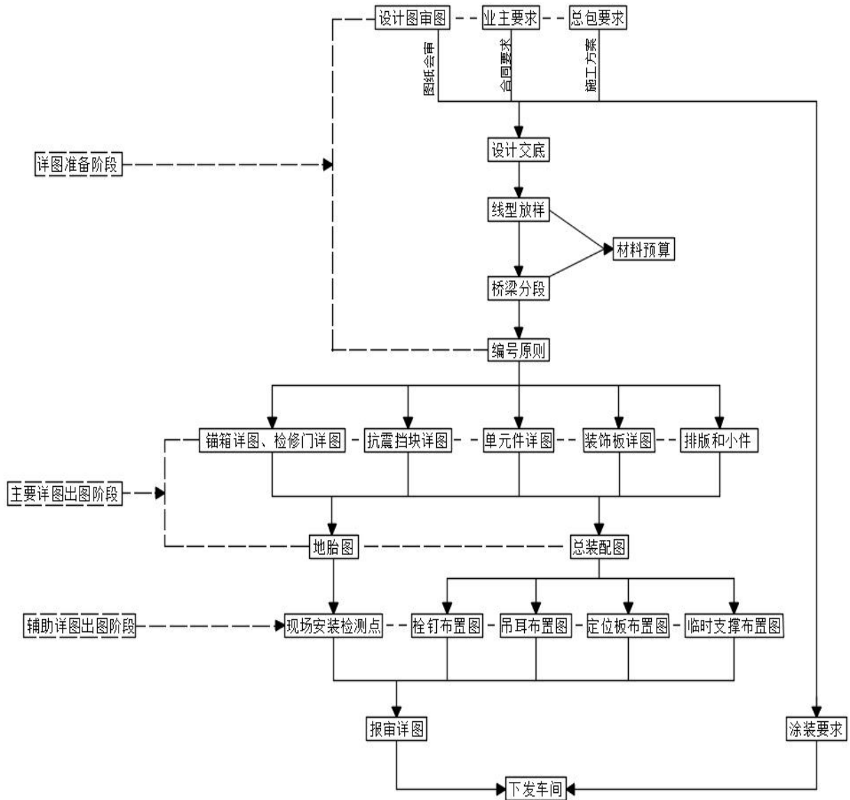
图 A.1.1 深化设计流程图
