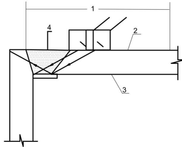
图 12.2.5-1 (b) 带有钢衬垫单面坡口接头焊缝根部区域检测示意图
