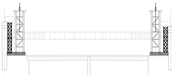
图 14.8.1-2 大节段钢梁提升法安装示意图
