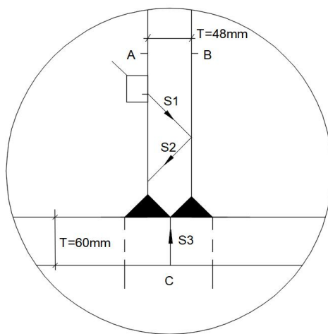
图 K.1.11 探头选用示例图
