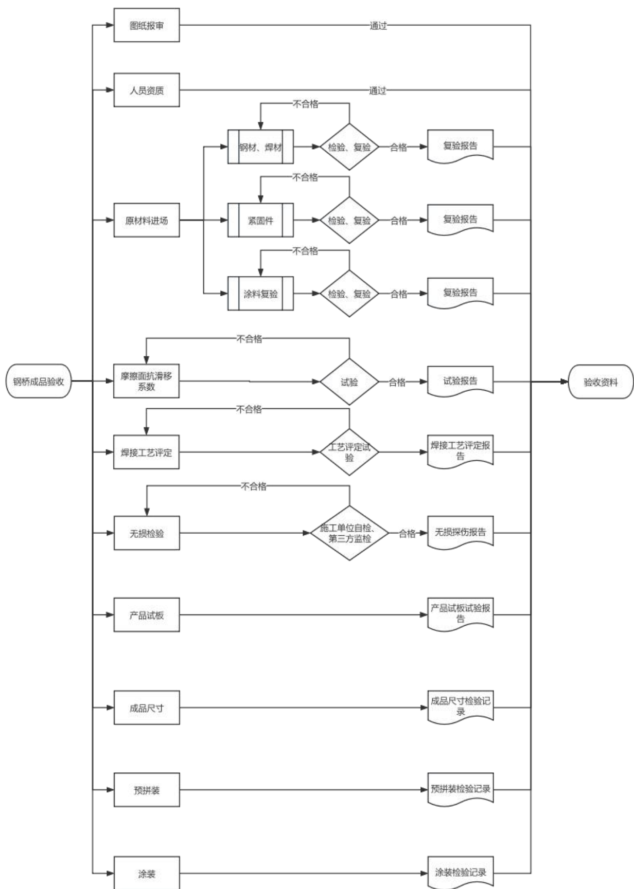
图 12.3.1 钢桥成品出厂验收流程图
