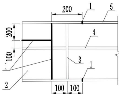
图 7.1.4-1 焊缝错开的最小距离（尺寸单位：mm）
