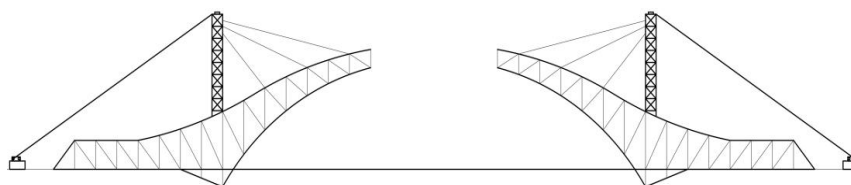
图 14.5.1-2 拱桥悬臂拼装法
