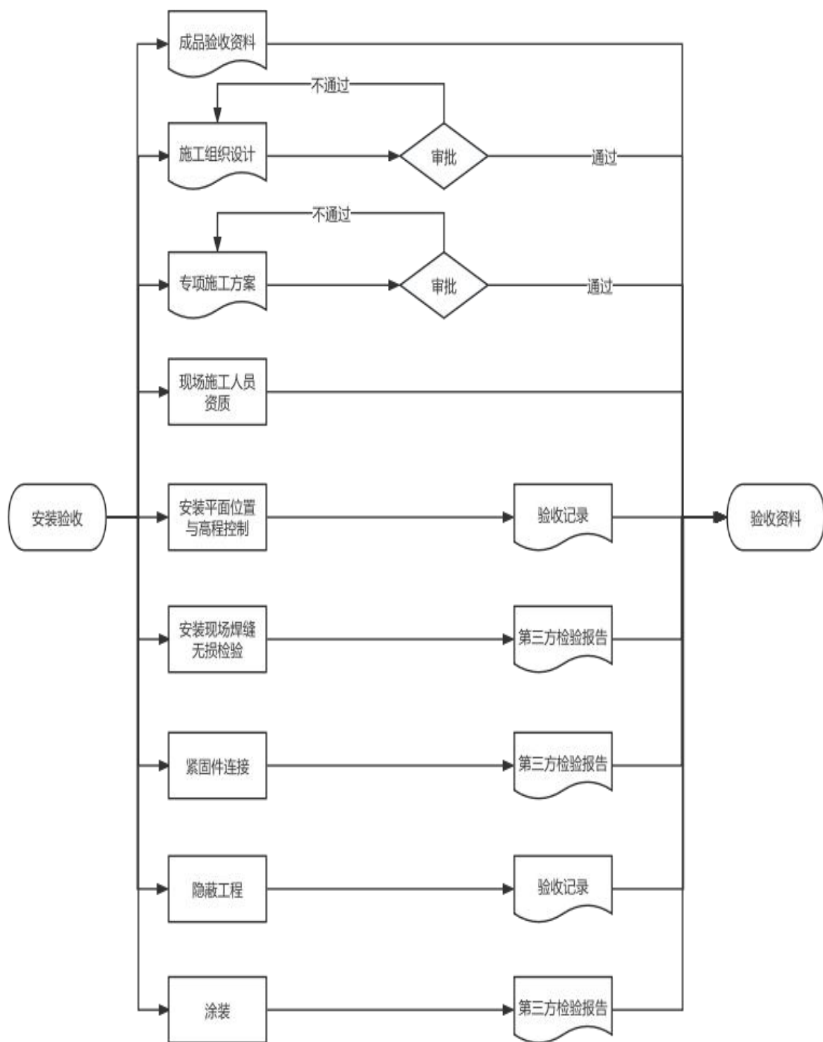
图 14.10.1-1 钢桥安装验收流程图
