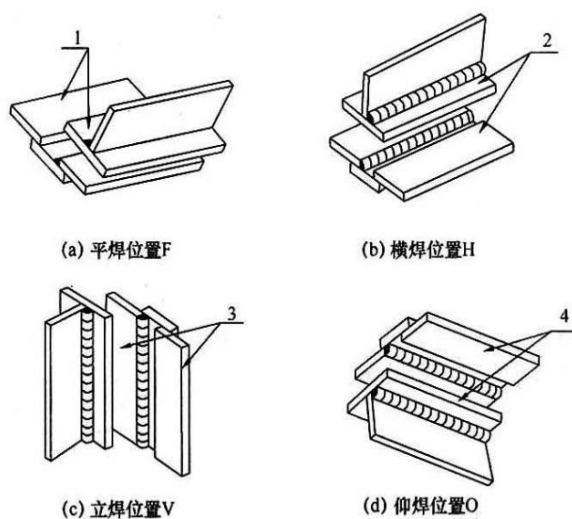
图 D.2.3-2 试板角焊缝焊接位置
