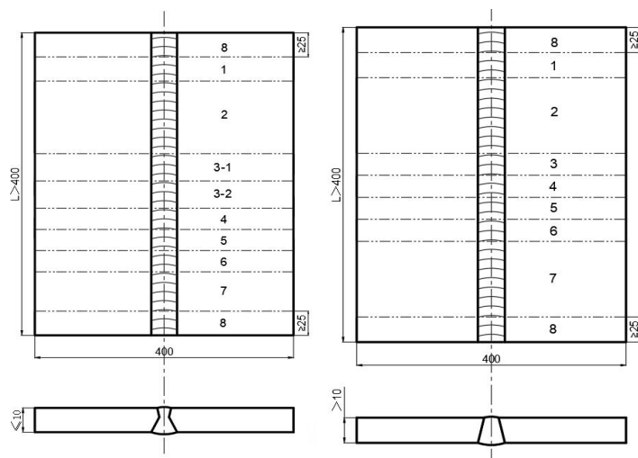
图 D.3.4-1 板材对接接头全熔透和部分熔透试件及试样取样
