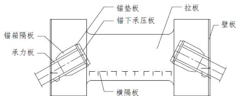
图 2 钢锚箱示意图
