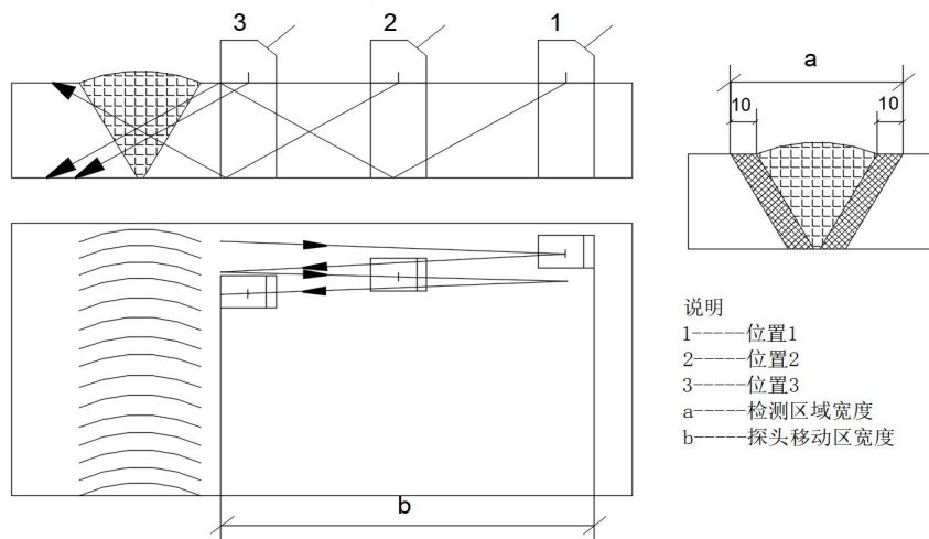
图 K.1.9 扫查纵向显示时检测区域示意图
