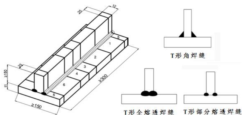
图 D.3.4-2 板材 T 形接头全熔透、部分熔透和角焊缝试件及试样取样
