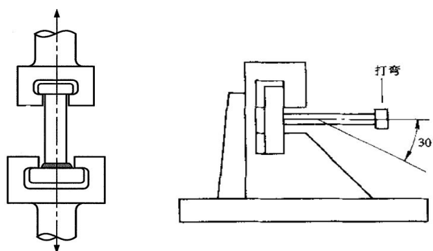
图 E.3.1-2 拉伸和弯曲实验形式
