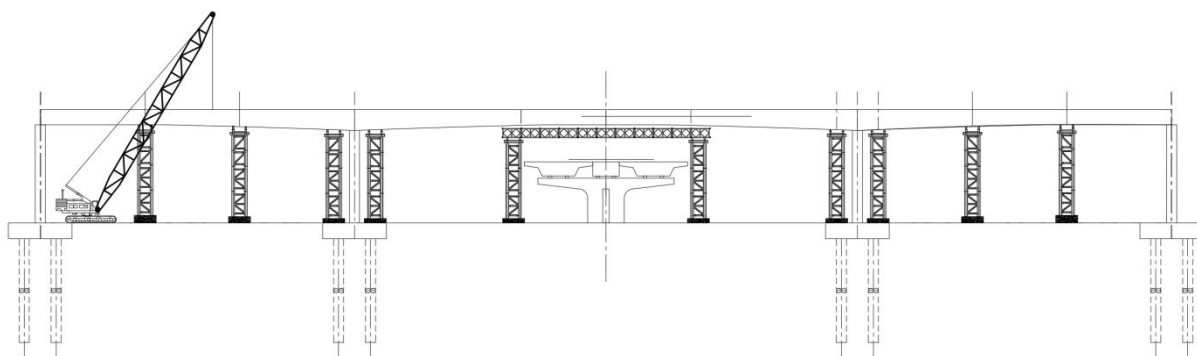
图 14.3.3-1 支架上安装示意图
