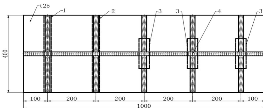
图 D.3.4-3 板材十字拼接接头全熔透焊缝试件取样
