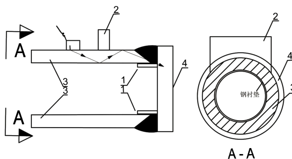
图 12.2.5-2 扫查面受限时 UT 检测补充扫查方法示意图
