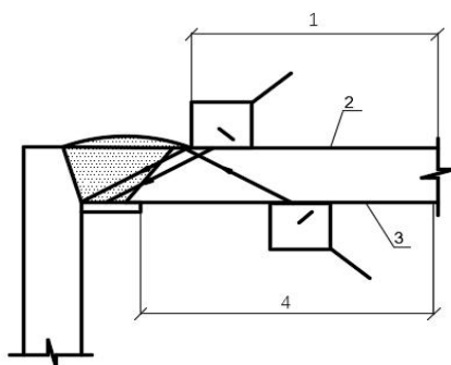
图 12.2.5-1 (c) 带有钢衬垫单面坡口接头焊缝根部区域检测示意图
