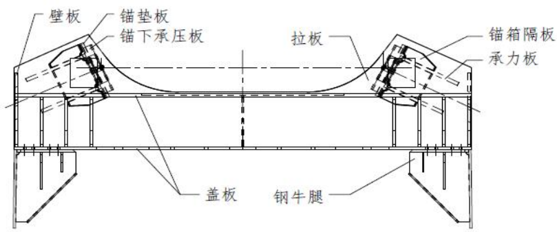
图 1 钢锚梁示意图
