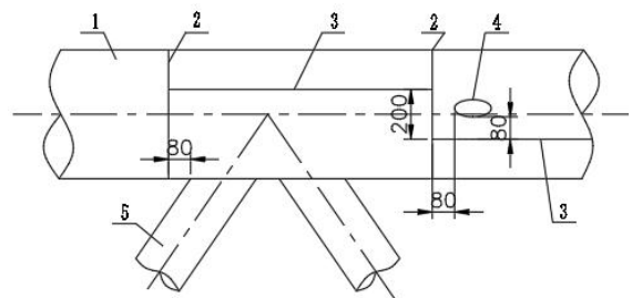
图 7.1.4-3 钢管拱弦管焊缝错开的最小距离（尺寸单位：mm） 1 一弦管； 2 一环焊缝； 3 一纵焊缝； 4 一相贯线焊缝； 5 一支管
