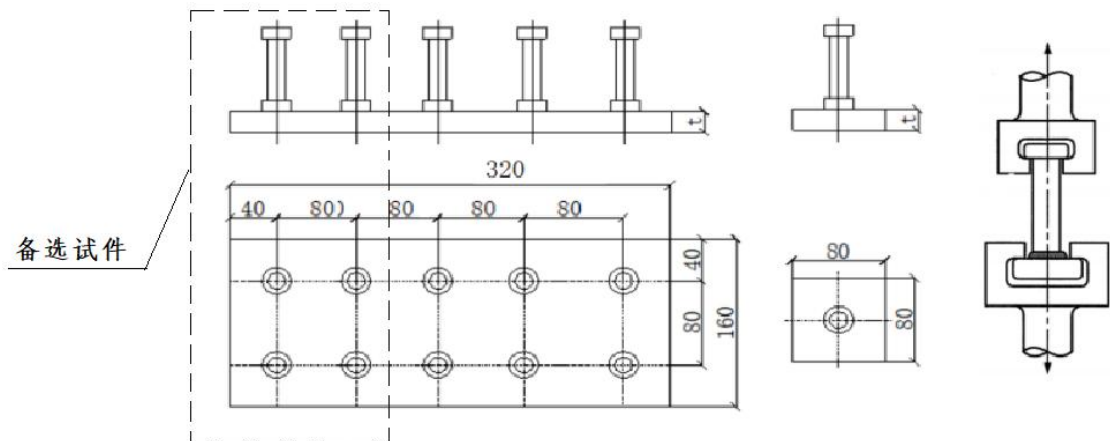
图 E.3.1-1 试件试样形式及尺寸
