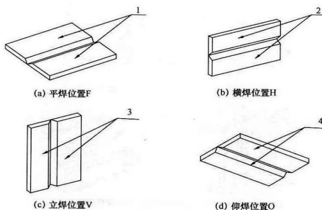
图 D.2.3-1 试板坡口焊缝焊接位置
