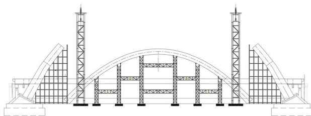
图 14.8.1-1 拱肋提升法安装示意图
