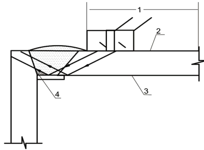
图 12.2.5-1 (a) 带有钢衬垫单面坡口接头焊缝根部区域检测示意图
