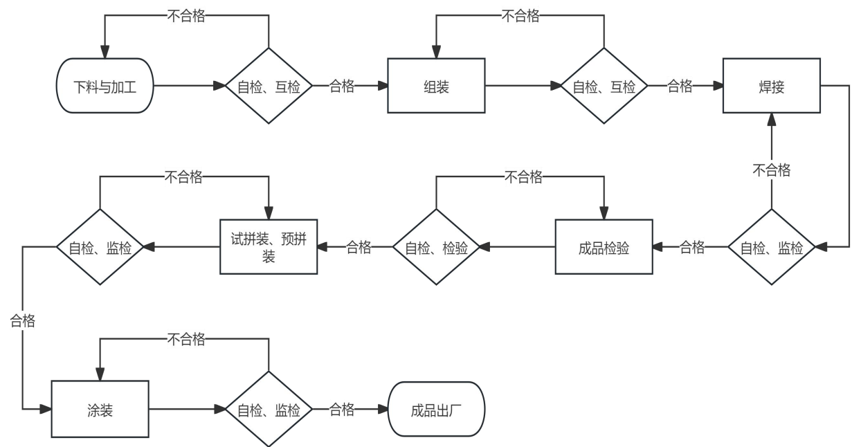
图 12.2.1 钢桥制作过程检验流程图
