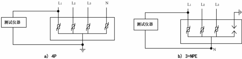
图10.1 电涌保护器压敏电压和泄漏电流测试接线示意图
