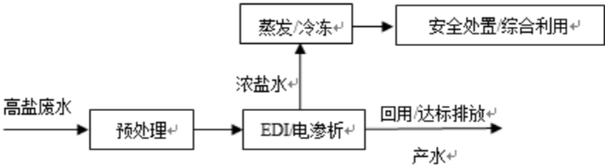
图2 电化学脱盐工艺流程图
