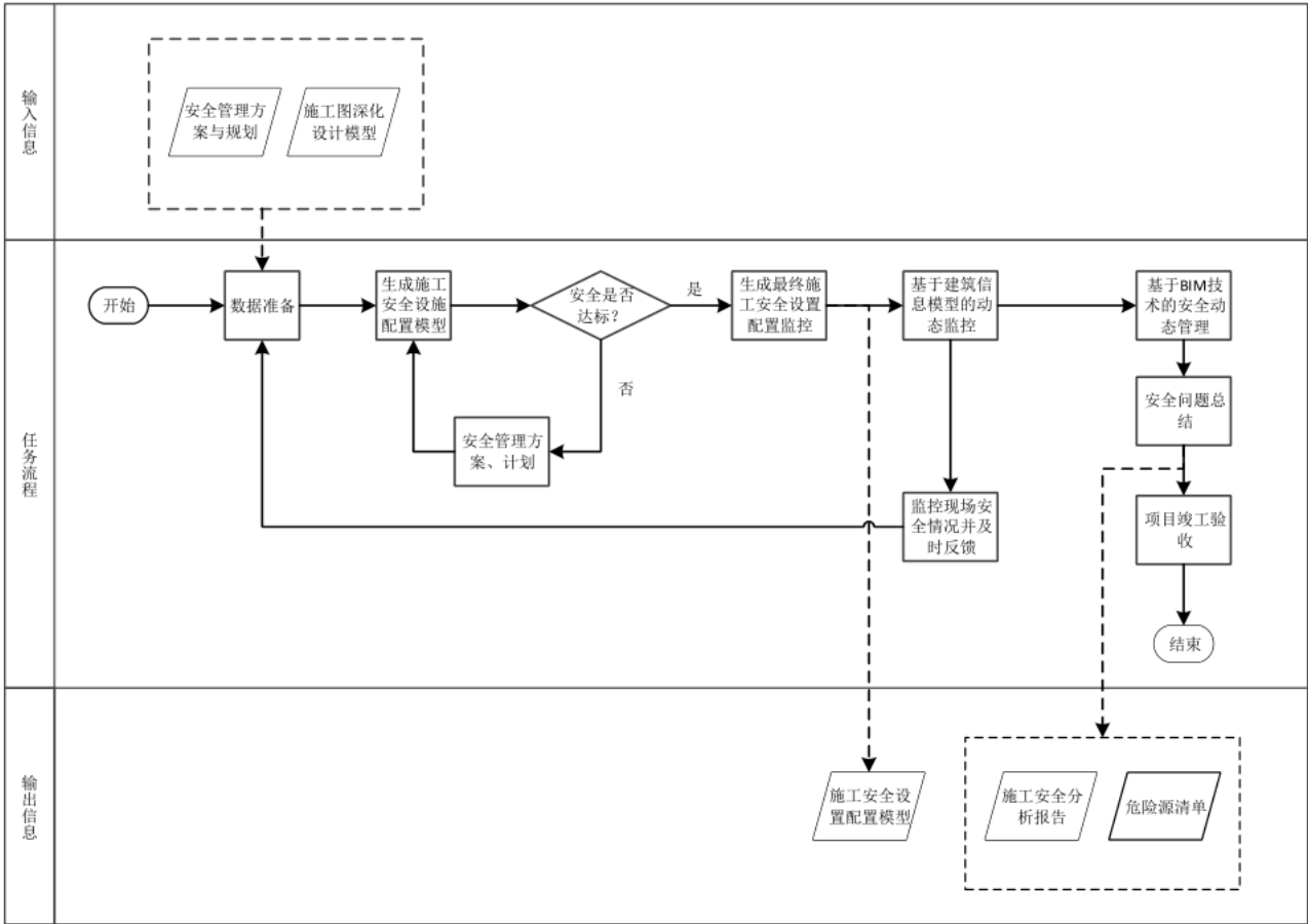
图23 施工安全管理 BIM 应用操作流程图
