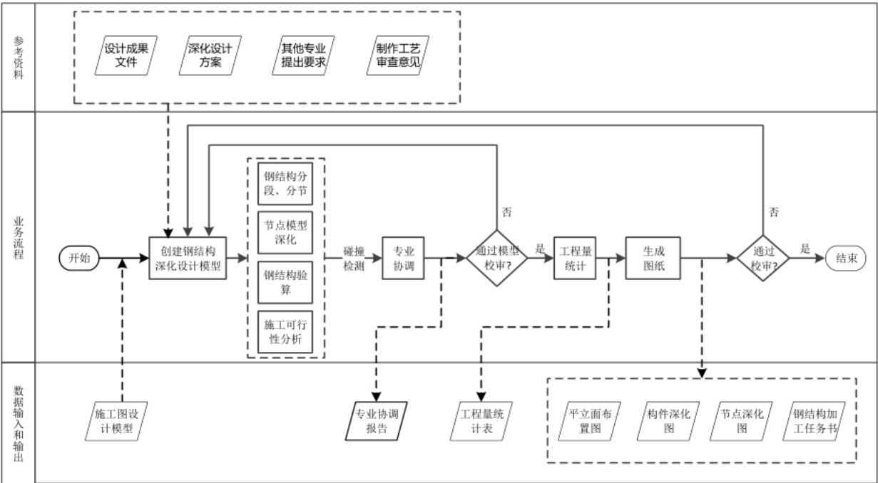
图29 钢结构深化设计 BIM 应用流程图
