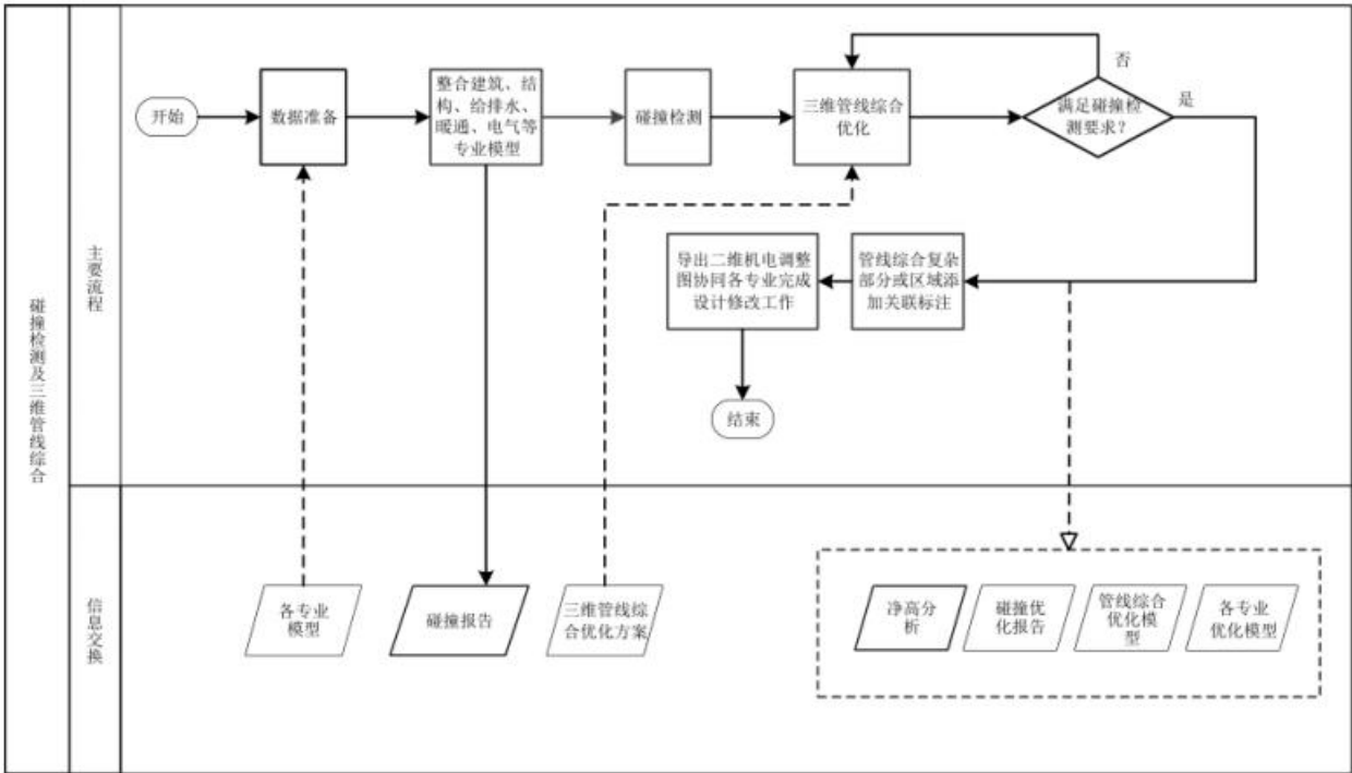
图8 碰撞检测及三维管线综合 BIM 应用操作流程
