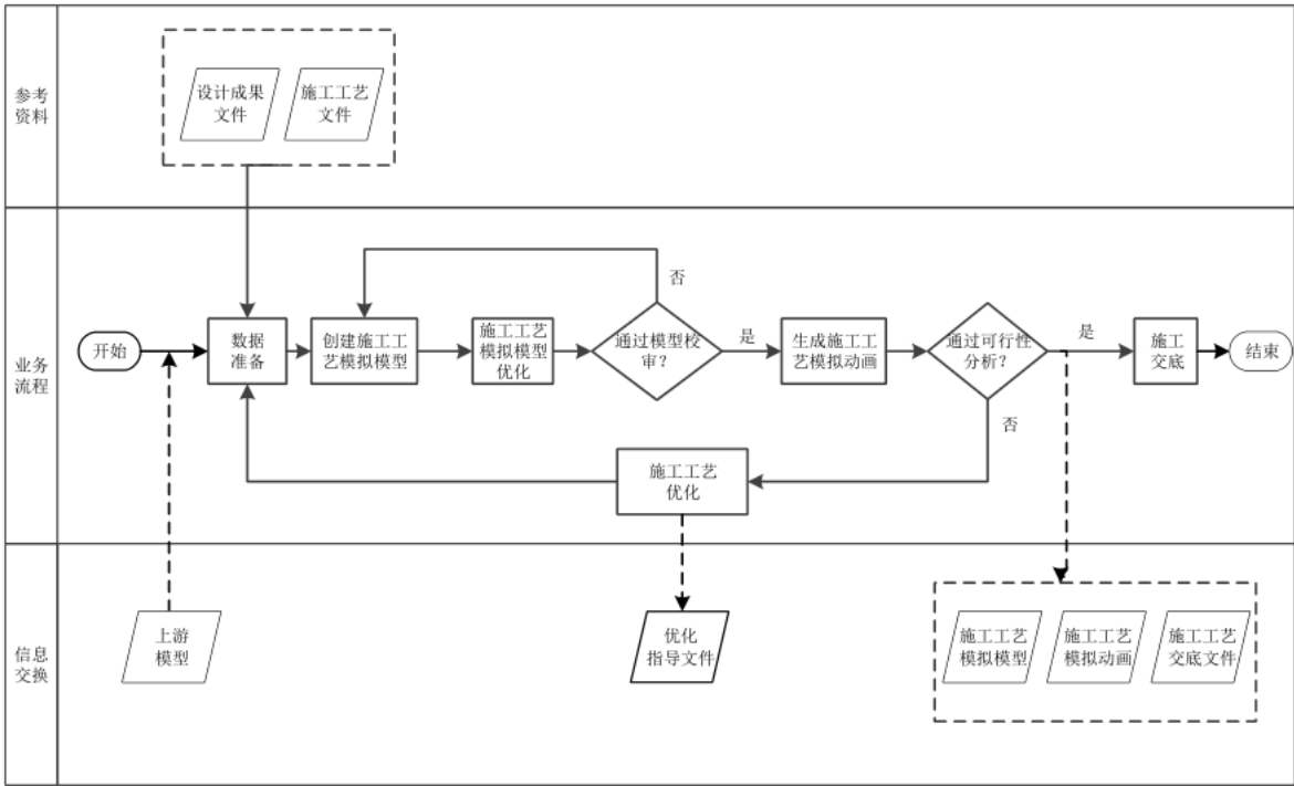
图16 施工工艺模拟 BIM 应用流程图
