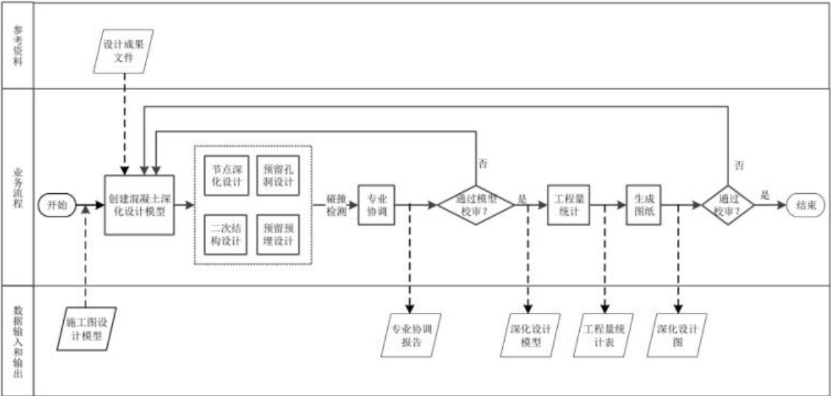
图11 现浇混凝土结构深化设计 BIM 应用流程图
