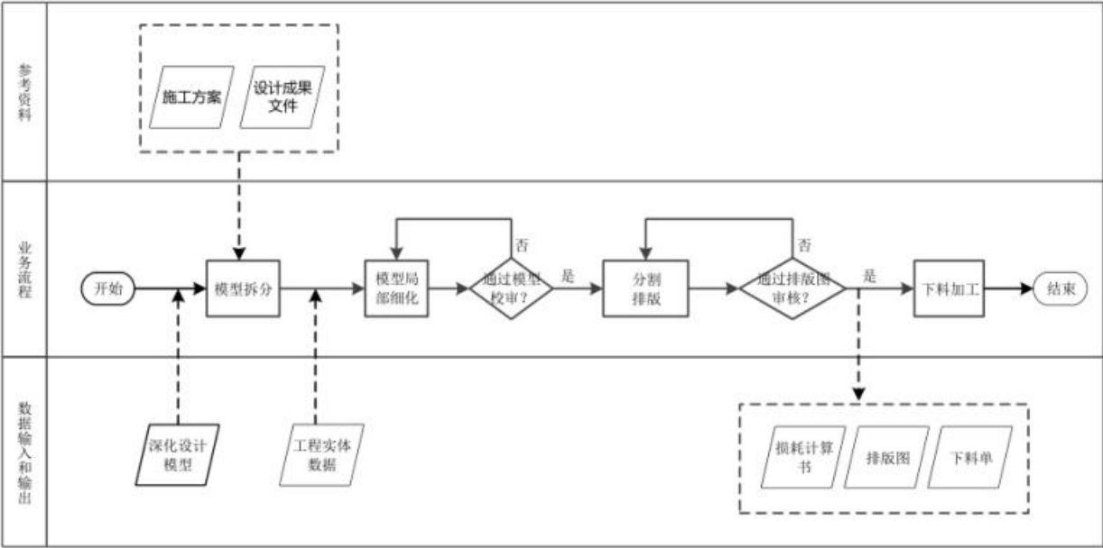
图14 装饰装修材料管理 BIM 工作流程图
