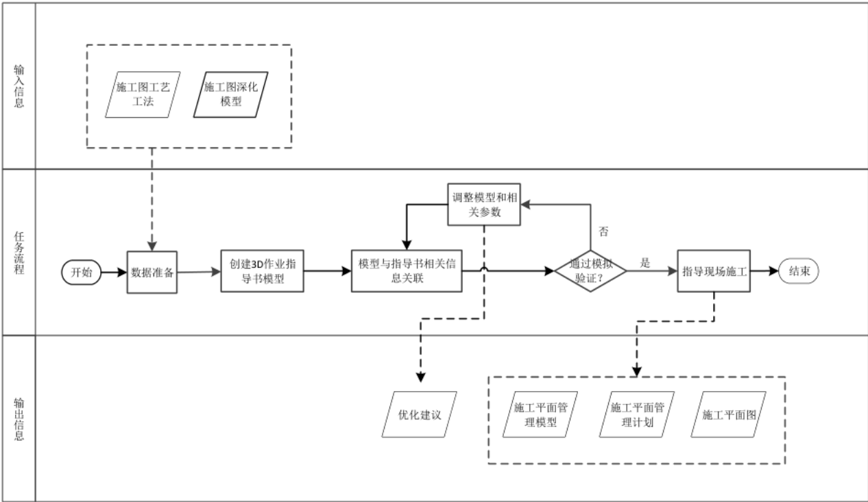
图20 三维作业指导 BIM 技术应用流程图
