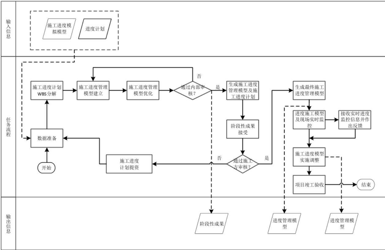
图21 施工进度管理 BIM 应用操作流程
