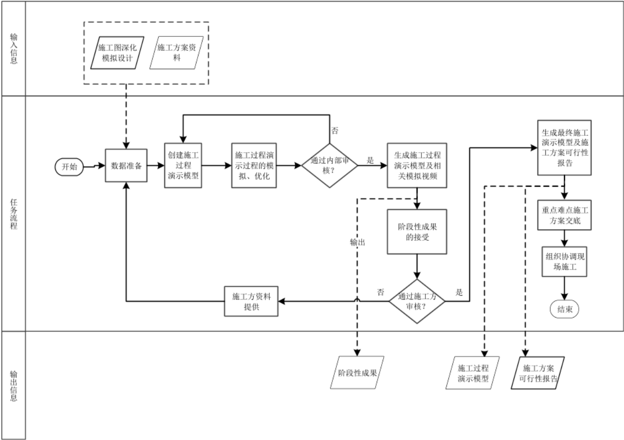
图19 施工方案模拟 BIM 应用操作流程
