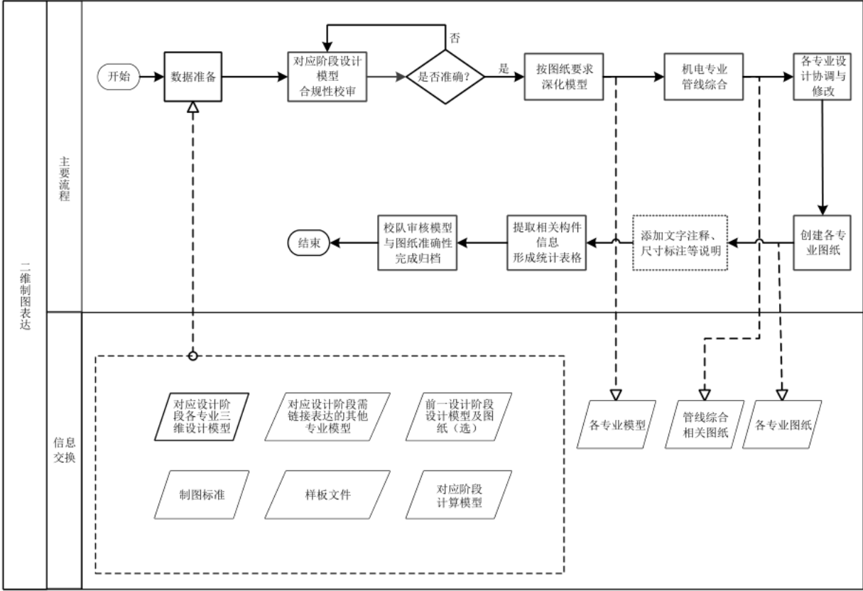
图9 二维制图表达 BIM 应用操作流程
