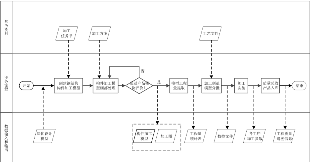
图30 钢结构构件加工制作设计 BIM 应用流程图
