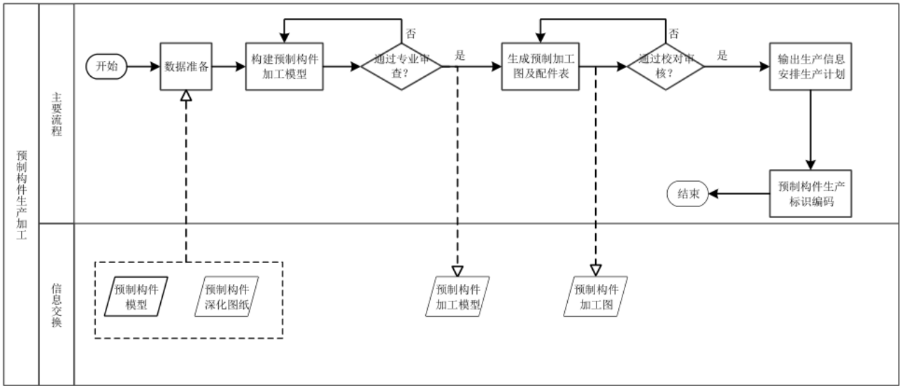
图33 预制构件生产加工 BIM 应用操作流程流程图
