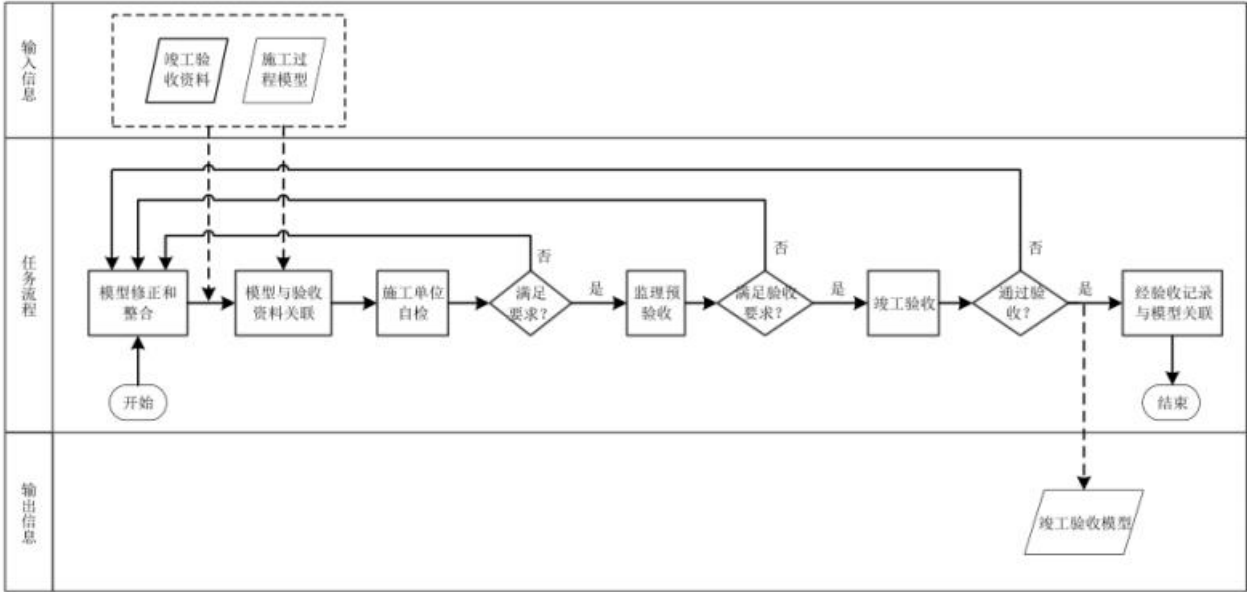
图26 竣工验收 BIM 应用流程图
