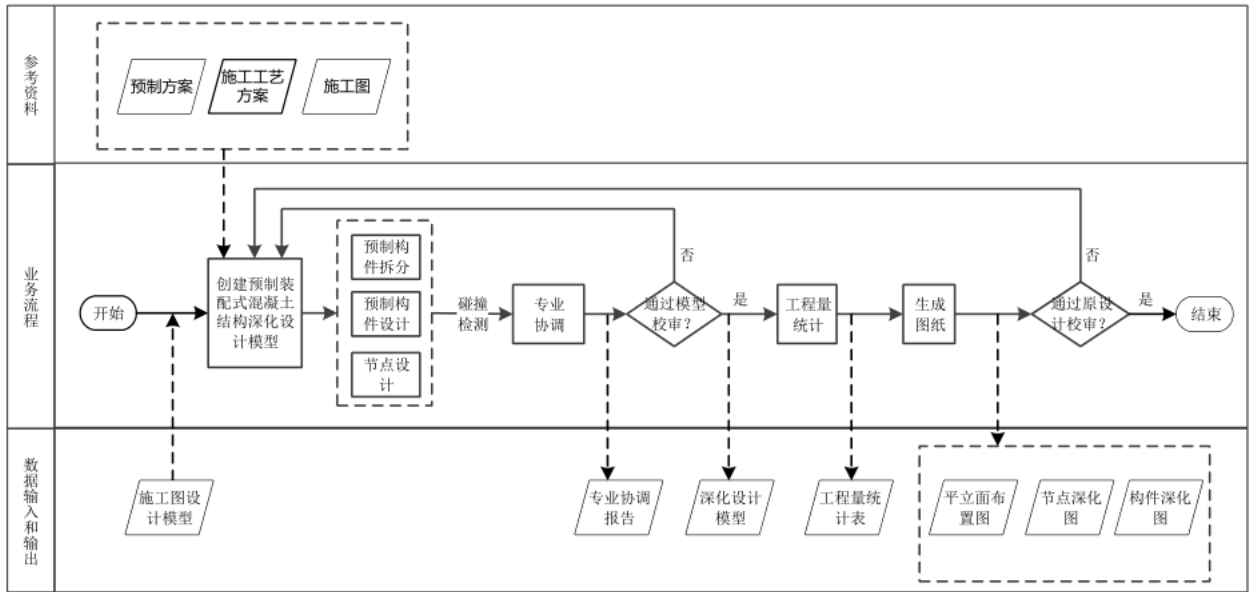
图27 装配式混凝土结构深化设计 BIM 应用流程图
