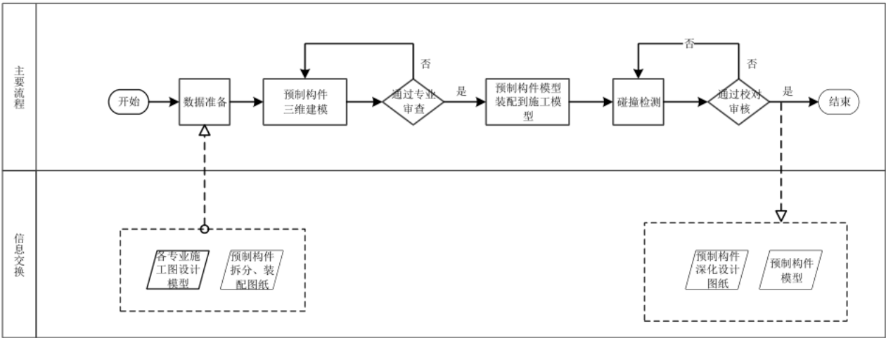
图32 预制构件碰撞检测 BIM 应用操作流程流程图
