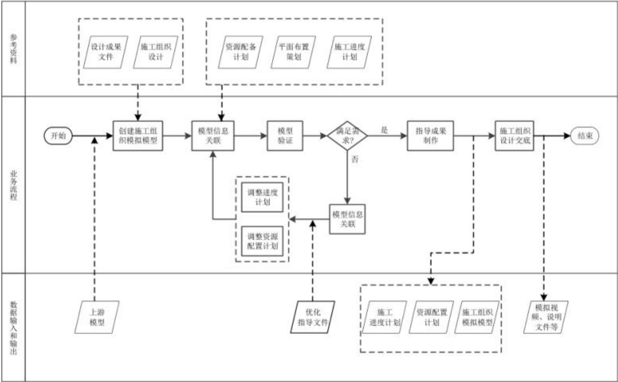
图15 施工组织模拟 BIM 工作流程图
