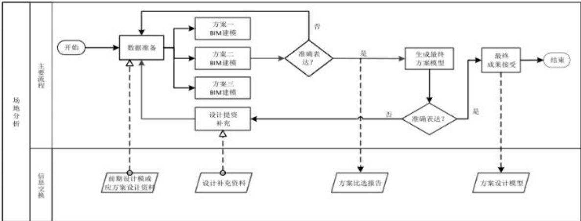
图3 方案设计比选 BIM 应用操作流程
