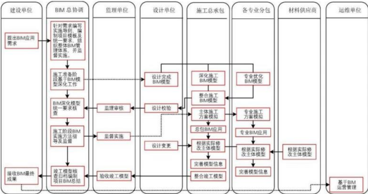
图1 工程 BIM 管理实施流程图
