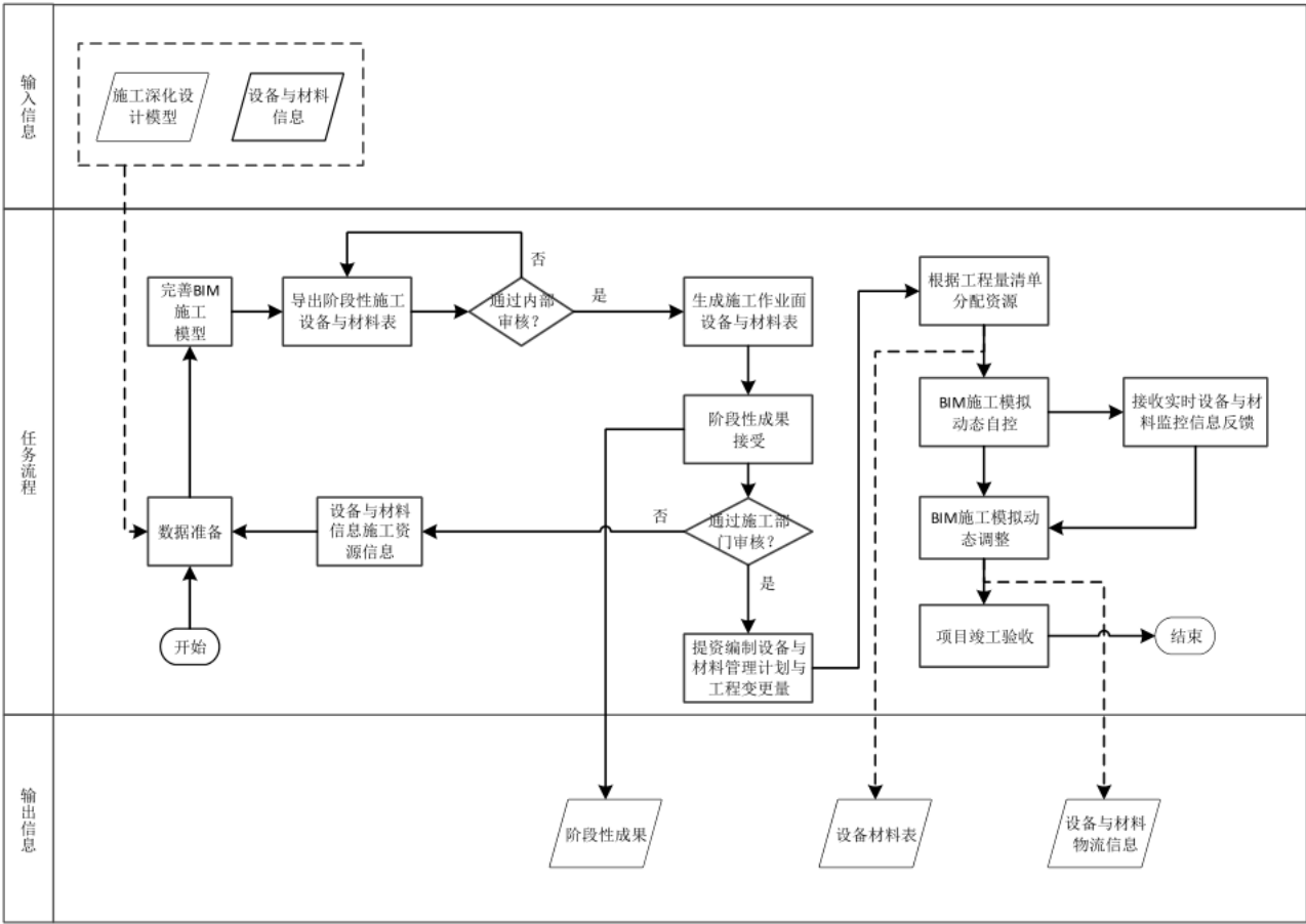
图24 设备与材料管理 BIM 应用操作流程
