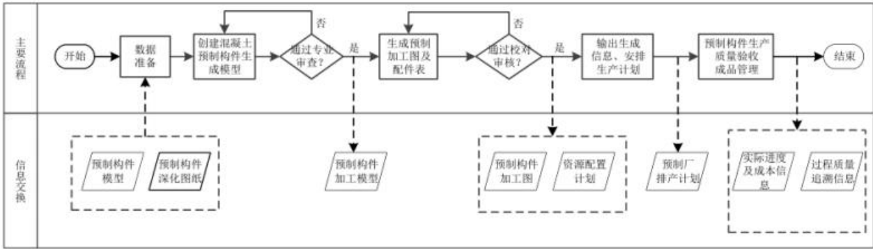
图28 混凝土预制构件生产 BIM 应用流程图
