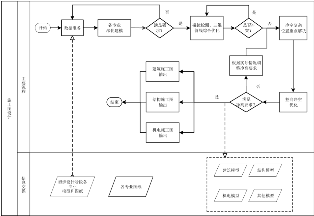
图7 施工图设计阶段 BIM 应用操作流程
