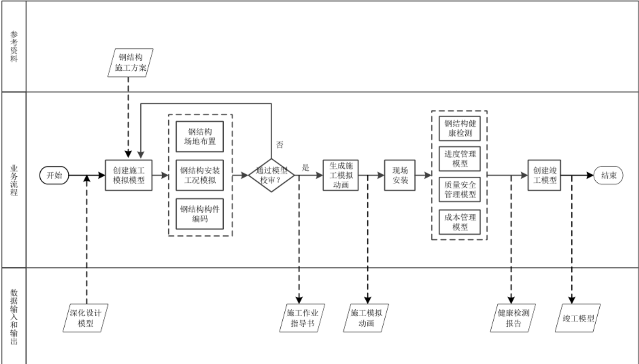
图31 钢结构现场安装施工模拟流程图
