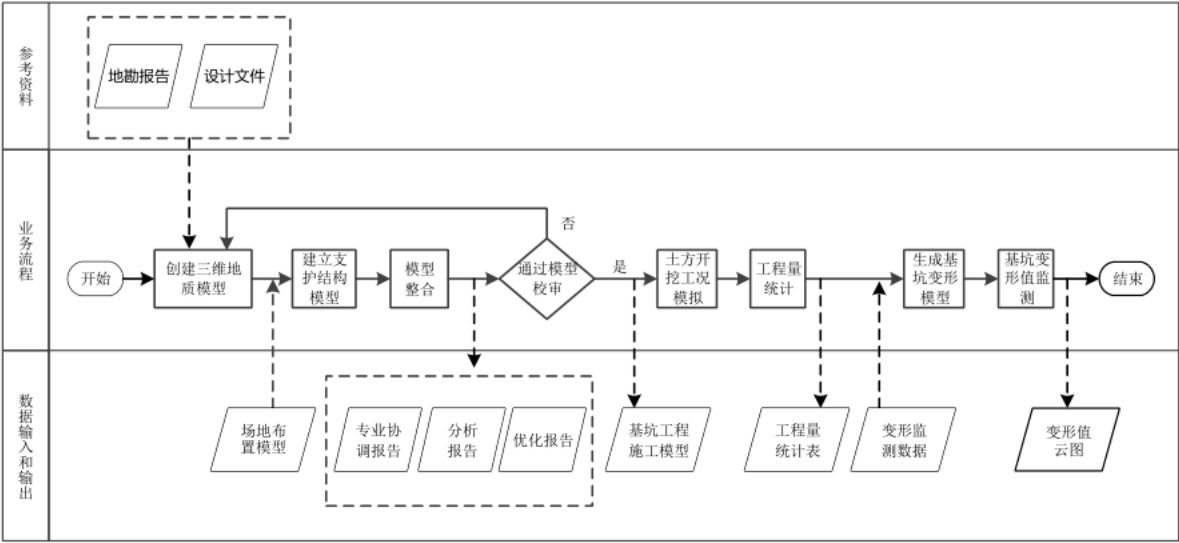
图10 基坑工程深化设计 BIM 应用流程图
