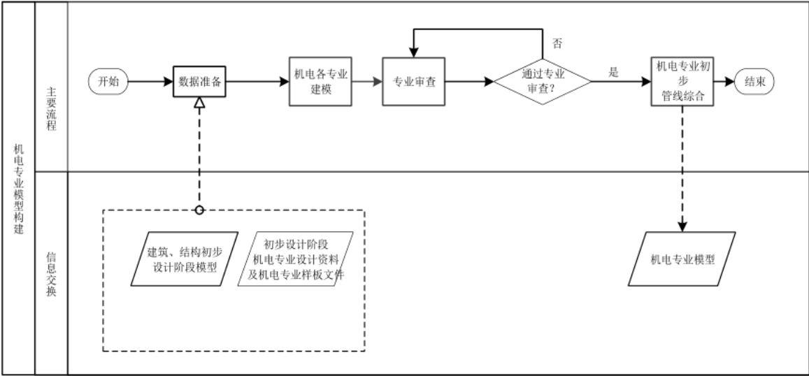
图6 机电专业初步设计阶段 BIM 应用操作流程
