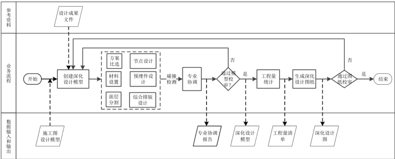
图13 装饰装修深化设计 BIM 应用流程图
