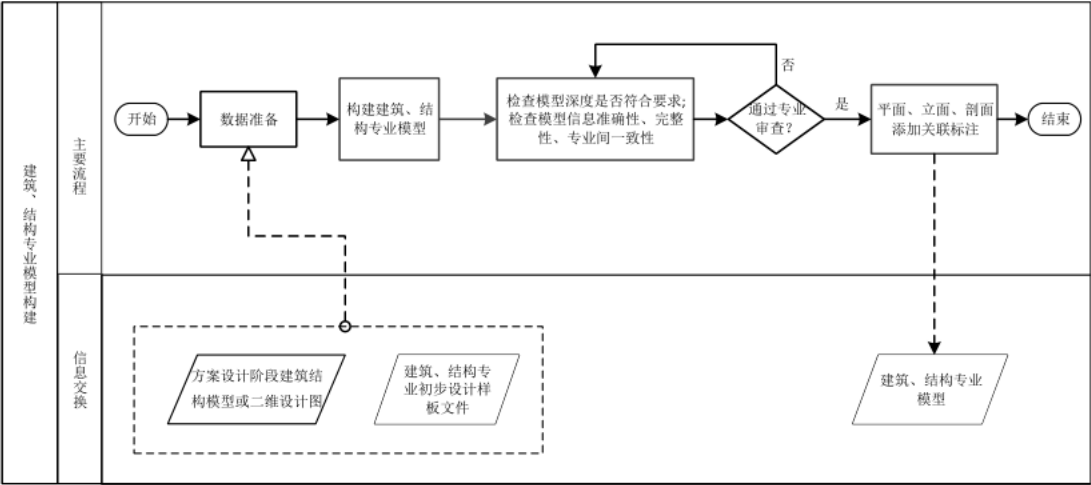
图5 建筑、结构专业初步设计阶段 BIM 应用操作流程
