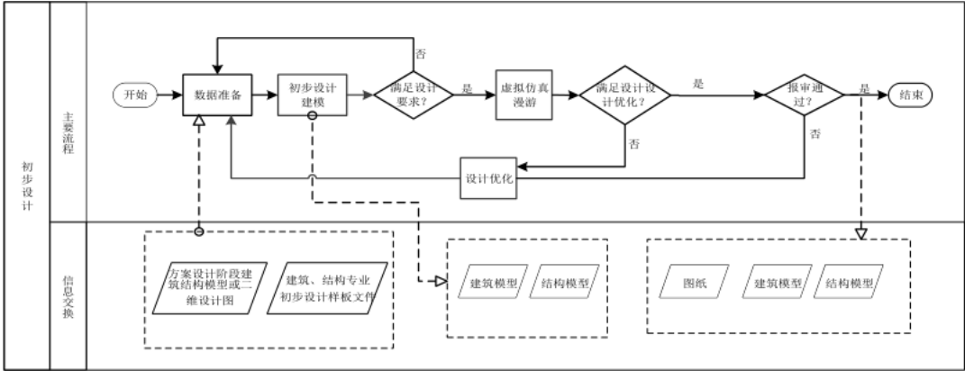
图4 初步设计阶段 BIM 应用操作流程
