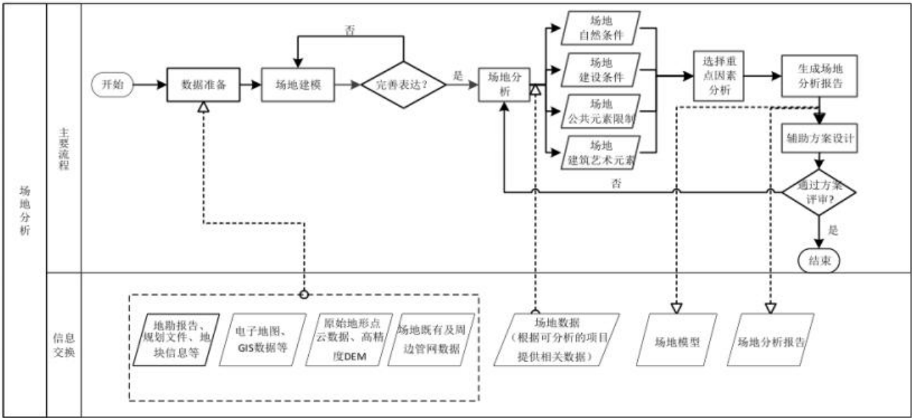
图2 场地分析 BIM 应用操作流程
