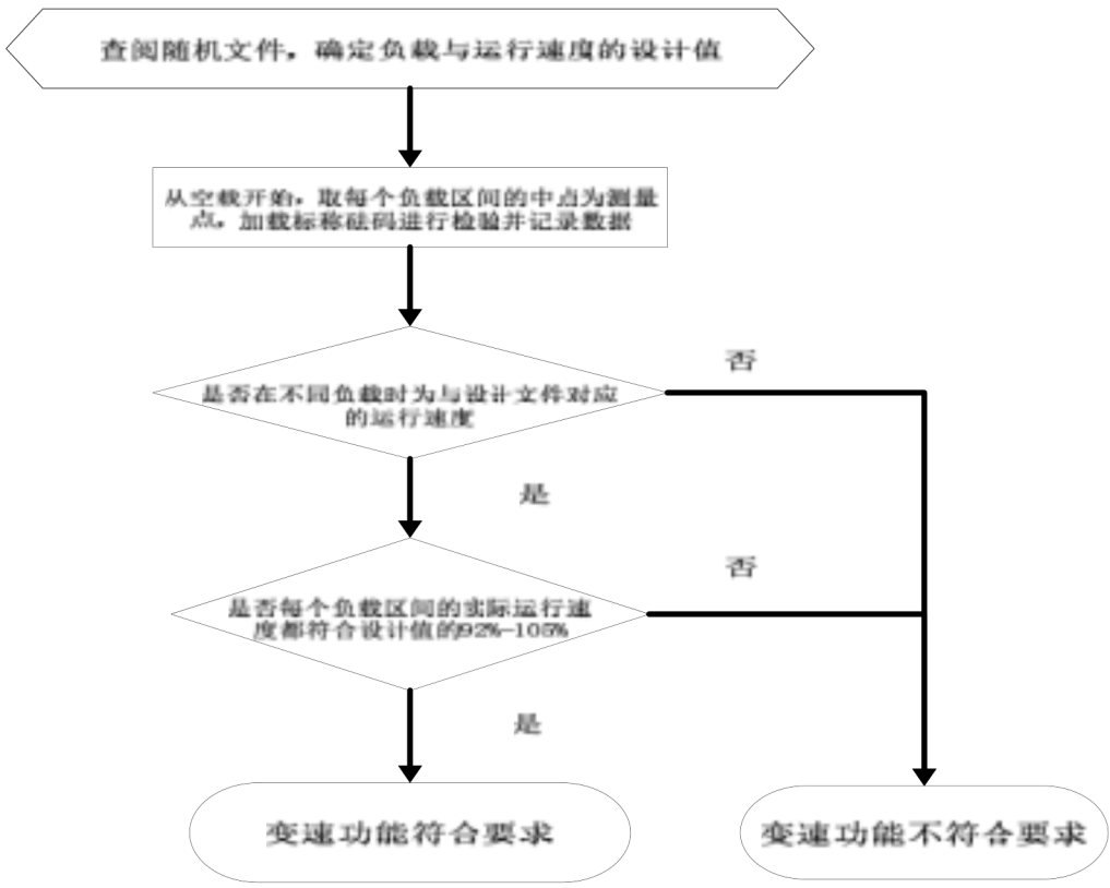
图B.1 变速功能试验流程图
